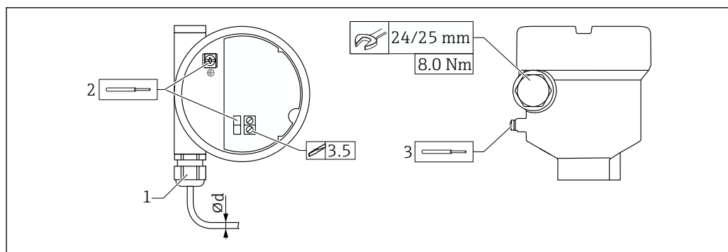
図 31 カップリングの例（電線管接続口、エレクトロニックインサートと端子）
