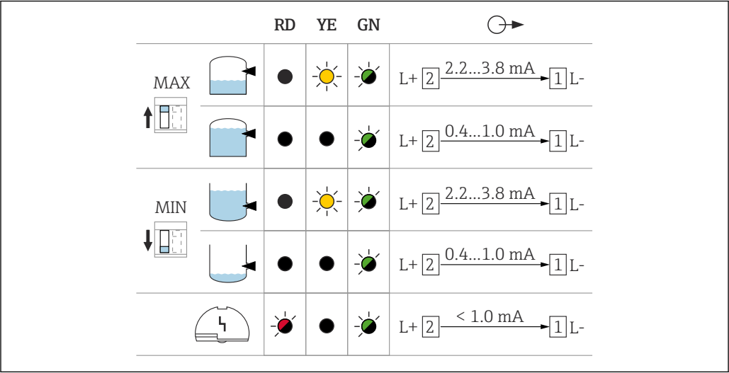
図 28 スイッチ出力および信号伝達の動作、エレクトロニックインサート FEL68
