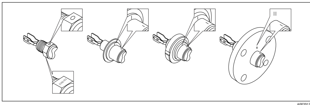
図 11 マークを使用して容器に水平に設置する場合の音叉部の位置
