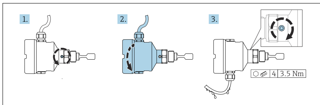
図 14 外部のロックネジおよびドリッブループ付きハウジング
