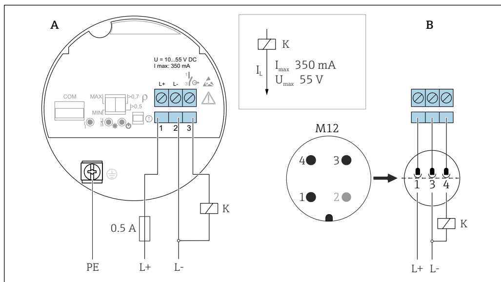
19 3線式DC-PNP、エレクトロニックインサート FEL62
