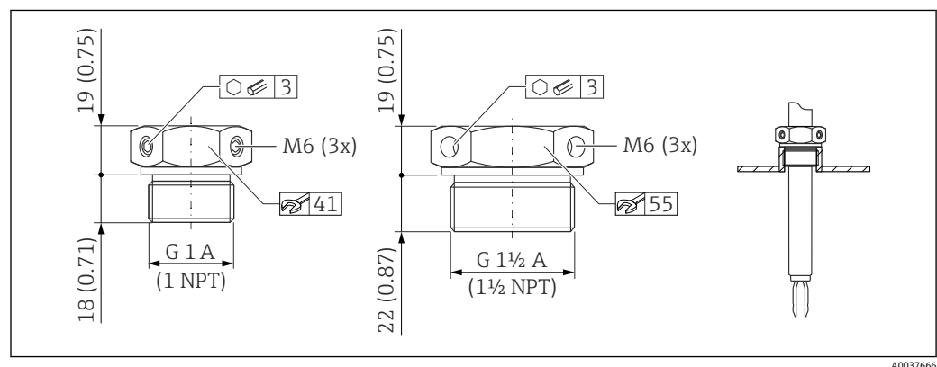
図 48 スライディングスリーブ（大気圧用： p_e = 0 \text{ MPa} (0 psi)）。測定単位 mm (in)
