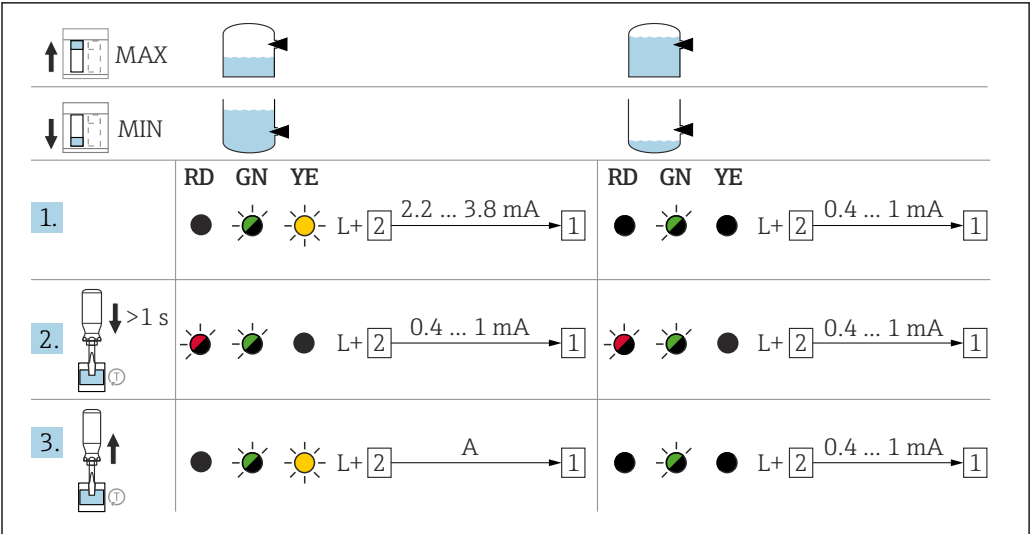
図 40 NAMUR 電子モジュールSwitching動作および信号伝達
