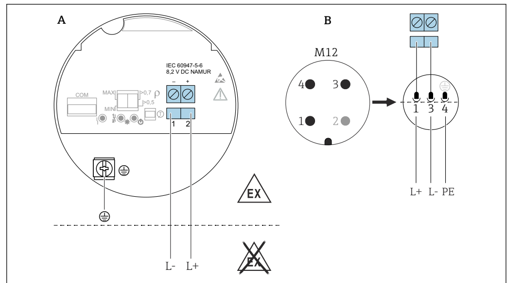
図 27 2 線式 NAMUR \geq 2.2 \text{ mA} / \leq 1.0 \text{ mA} 、エレクトロニックインサート FEL68
