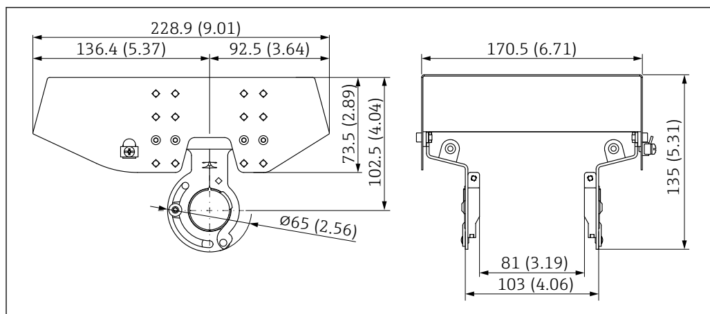
図 44 アルミニウム製デュアルコンパートメントハウジング用保護カバー。測定単位 mm (in)
