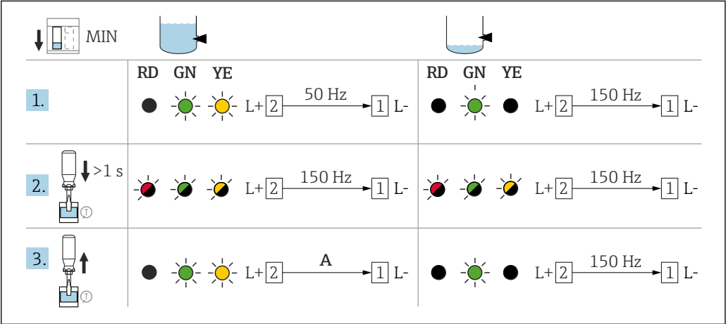
39 FEL67 下限 (MIN) スイッチング動作および信号伝達
