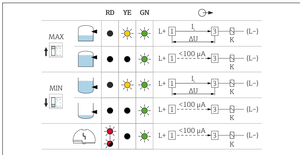
20 スイッチ出力および信号伝達の動作、エレクトロニックインサート FEL62
