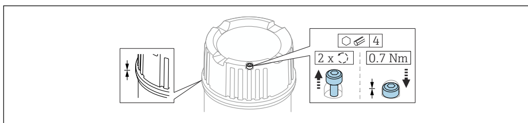
図 15 固定ねじ付きカバー
