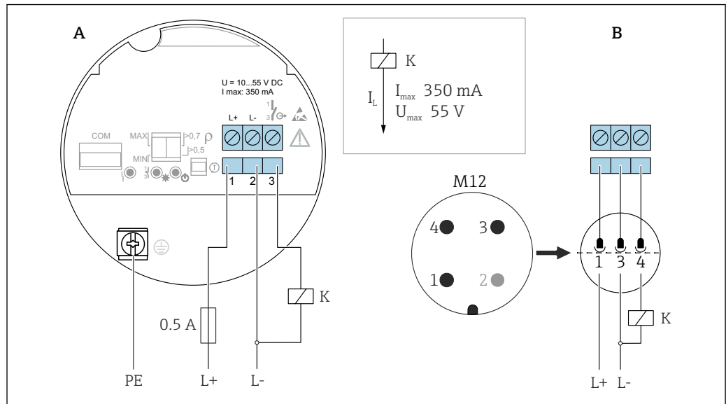
図 19 3線式 DC-PNP、エレクトロニックインサート FEL62
