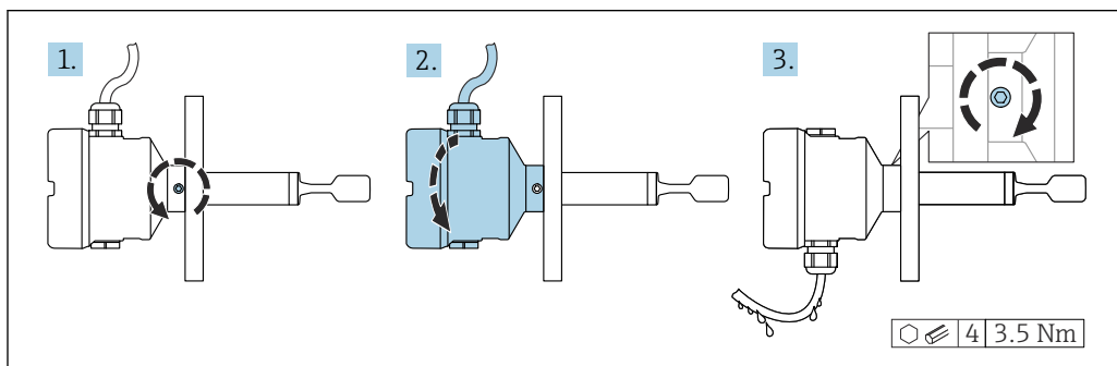
図 14 外部のロックネジおよびドリッループ付きハウジング
