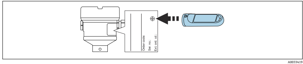
図 42 テストマグネットを使用した機能テスト
