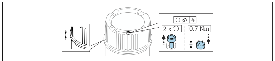
図 15 固定ねじ付きカバー
