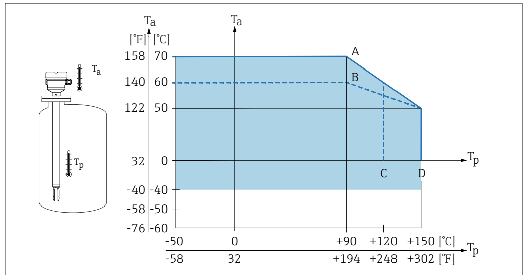
図 49 容器内のプロセス温度 T_p に応じたハウジングの許容周囲温度 T_a
