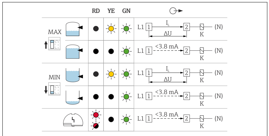
図 17 スイッチ出力および信号伝達の動作、エレクトロニックインサート FEL61
