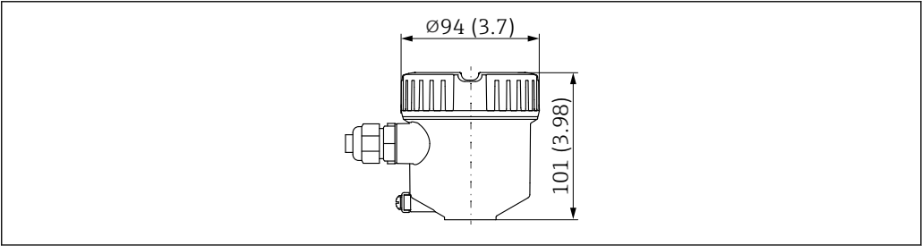
图 28 单腔体塑料外壳的外形尺寸示意图；外壳盖不带观察窗。测量单位 mm (in)
