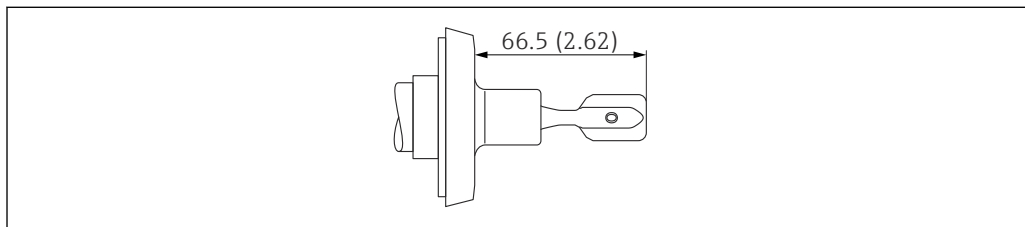
图 41 DIN11851 管接头。测量单位 mm (in)
