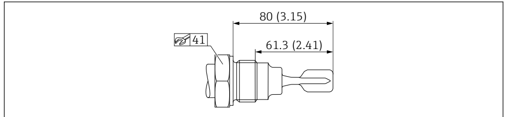
38 ISO228 G 1 螺纹。测量单位 mm (in)
