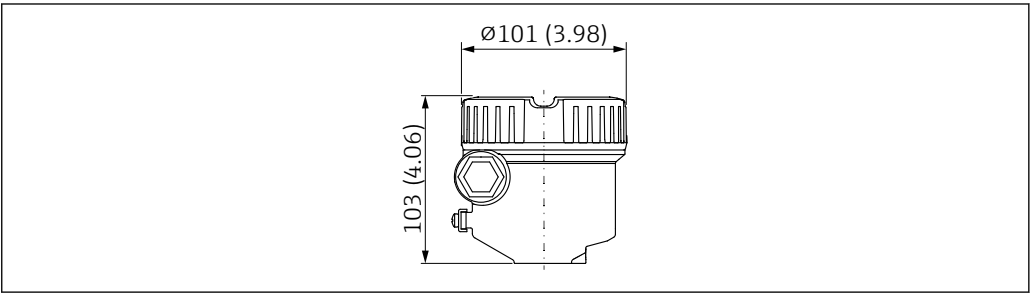
图 29 单腔体铝外壳的外形尺寸示意图；外壳盖不带观察窗。测量单位 mm (in)
