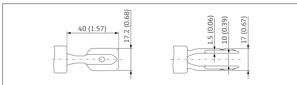
图 35 叉体。测量单位 mm (in)
