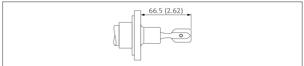
43 DRD 接头。测量单位 mm (in)
