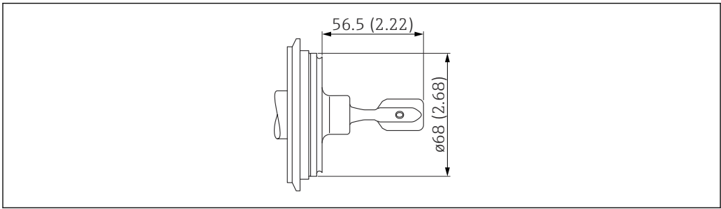
45 Varivent N 型接头，DN65-162 PN25 配合管道。测量单位 mm (in)
