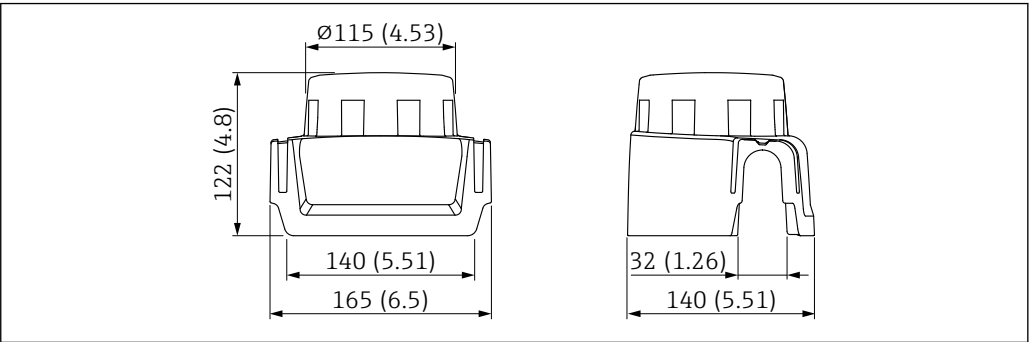
图 53 防护罩，适用单腔体铝外壳。测量单位 mm (in)
