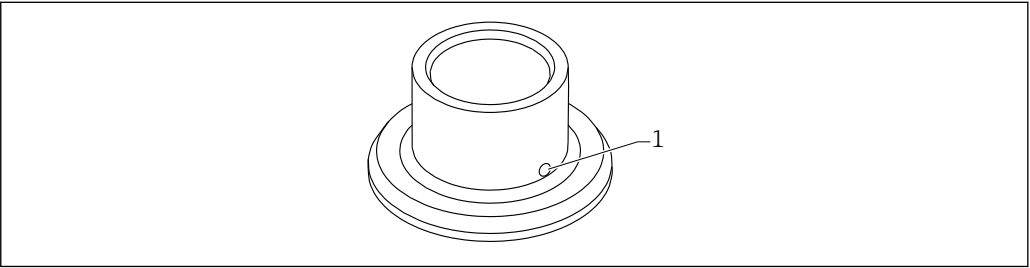
图 54 焊座，带泄漏检测孔（示意图）
