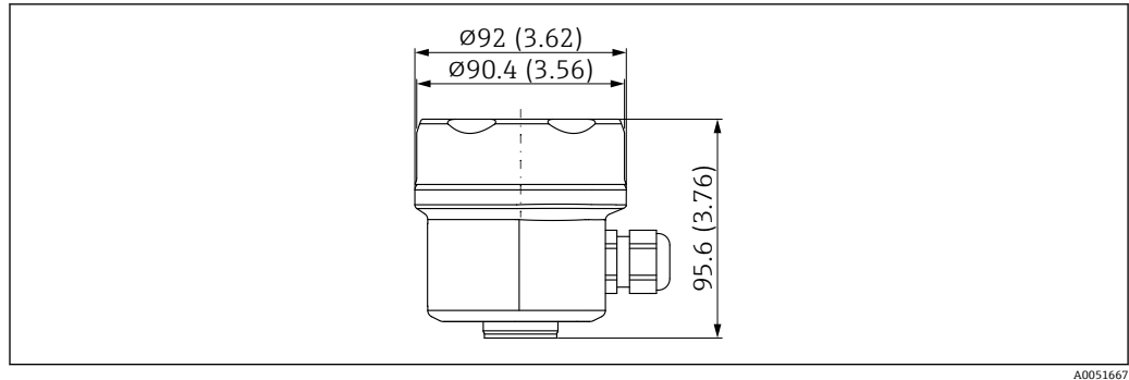
图 31 单腔体 316L 外壳（卫生型）的外形尺寸示意图；外壳盖不带观察窗。测量单位 mm (in)
