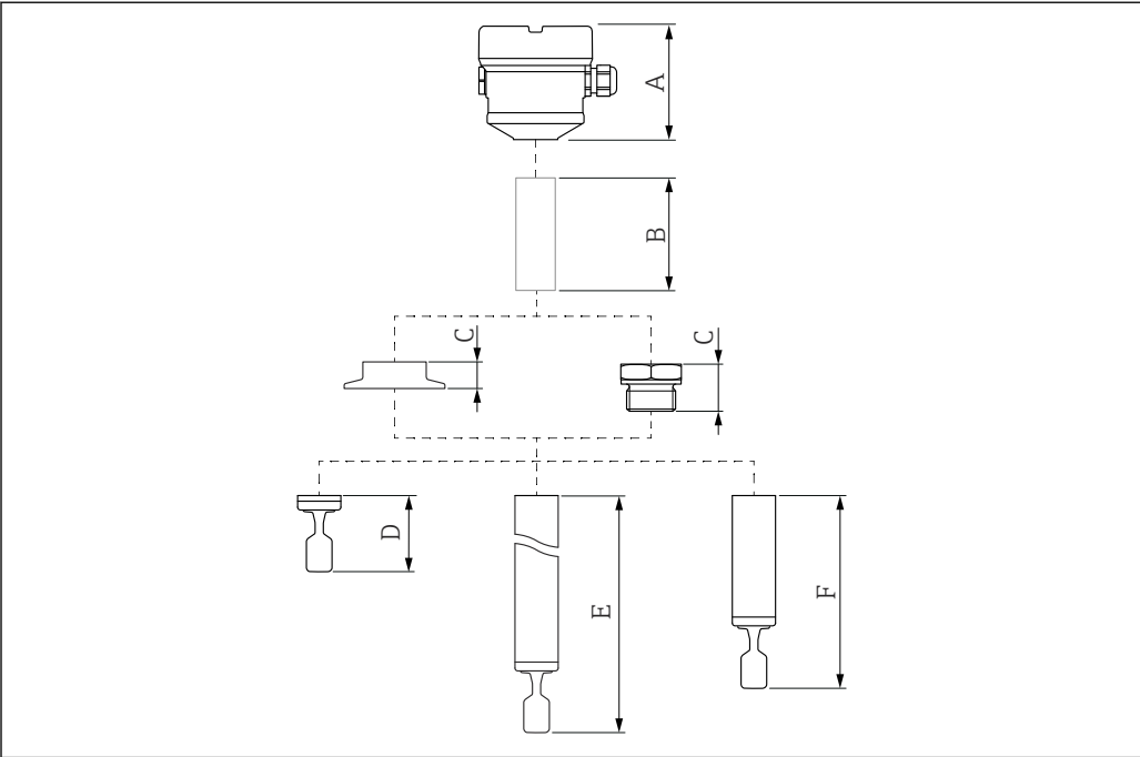
图 27 计算设备高度所需考虑的部件
