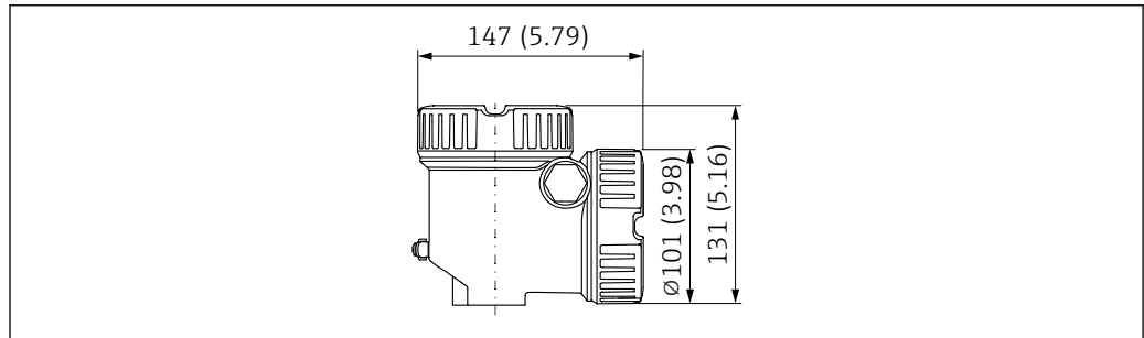
图 32 双腔体 L 型铝外壳（带涂层）的外形尺寸示意图；适用 Ex d/XP、粉尘防爆场合；外壳盖不带观察窗。测量单位 mm (in)
