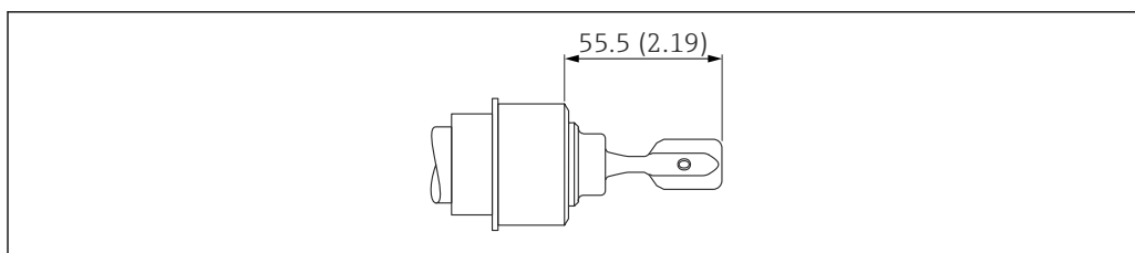
图 40 罐体接头（齐平安装在焊座中）。测量单位 mm (in)
