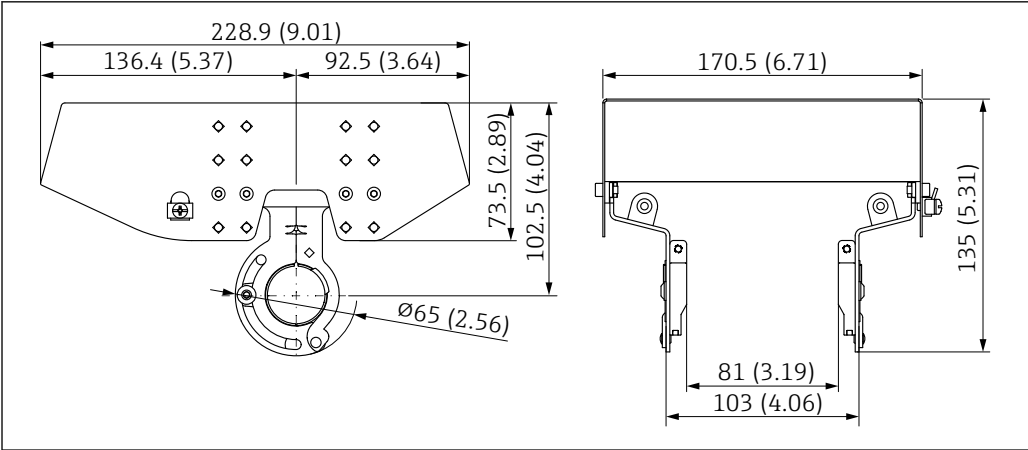
52 双腔体铝外壳的防护罩。测量单位 mm (in)
