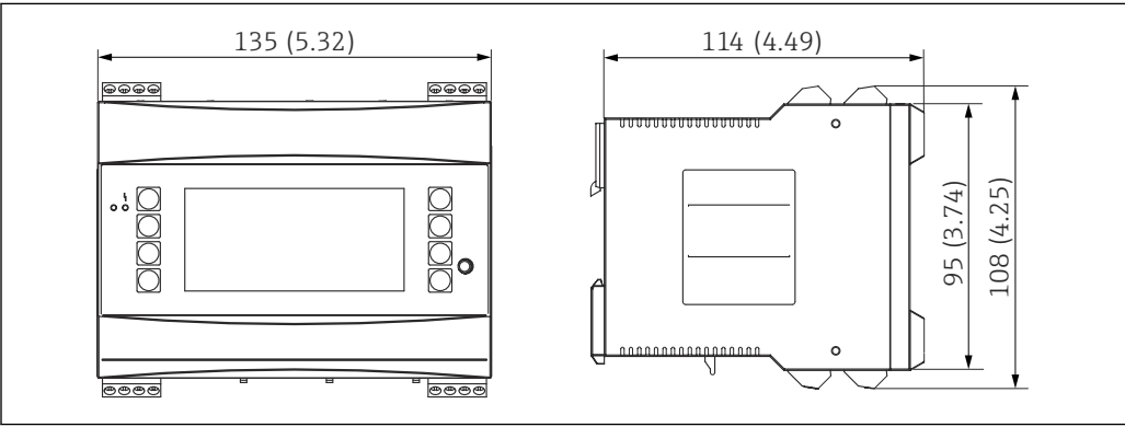
图 48 DIN 导轨盘装型外壳，符合 IEC 60715 标准。测量单位 mm (in)
