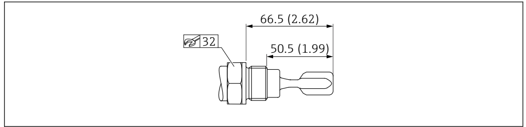
37 ISO228 G 3/4 螺纹。测量单位 mm (in)
