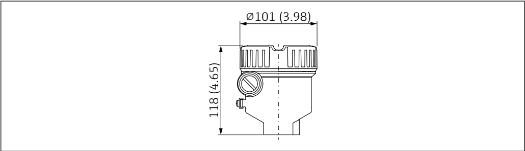
图 30 单腔体铝外壳（带涂层）的外形尺寸示意图；适用 Ex d/XP、粉尘防爆场合；外壳盖不带观察窗。测量单位 mm (in)
