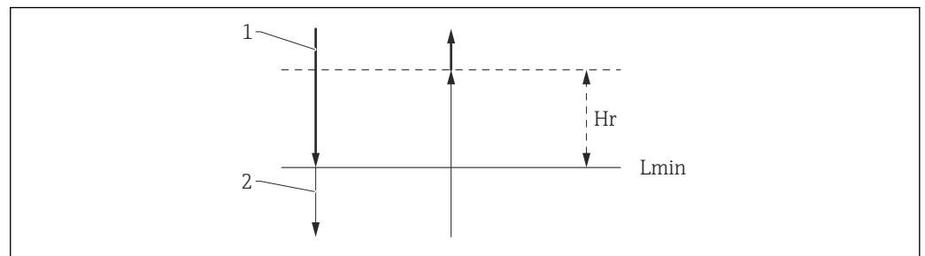
98 HTMS 单点回差控制范围
