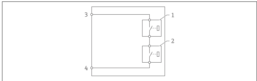
🔍 92 数字量输出的两个继电器
