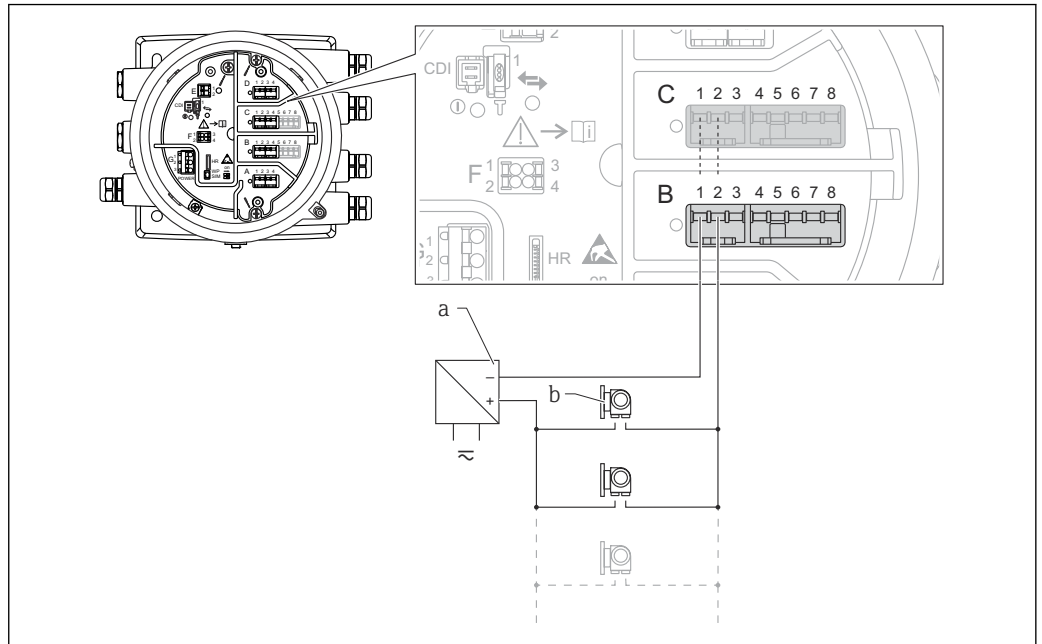
图 23 HART 主站模式下的无源模拟量输入/输出模块
