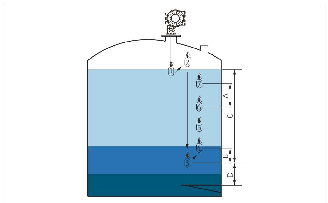
图 56 手动梯度位移 (数字显示浮子的移动顺序) 示意图
