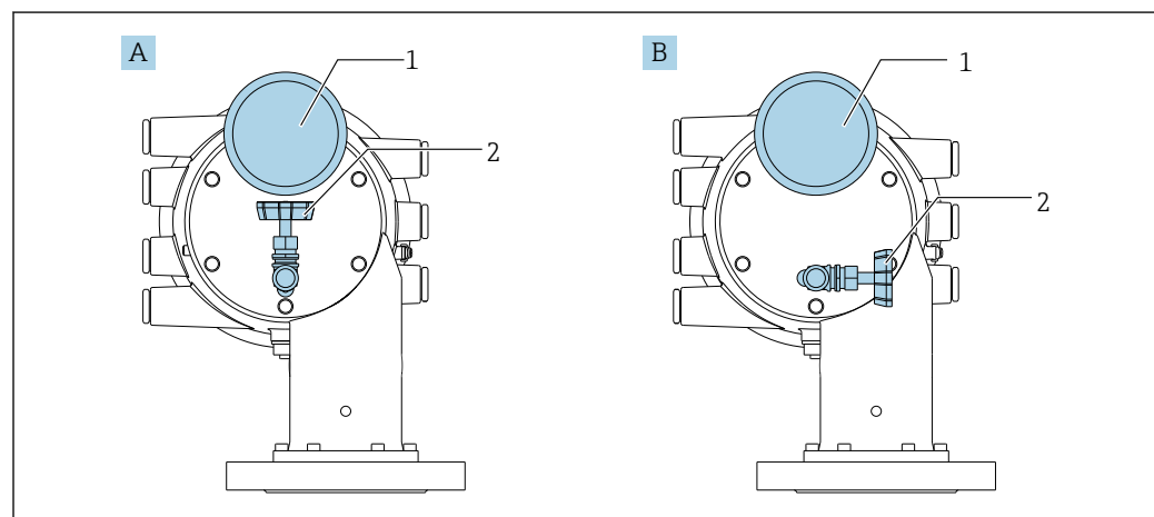
图 80 减压阀和压力表的安装位置
