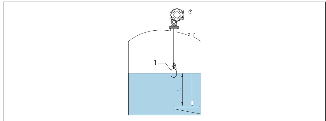
图 48 设置敞开式储罐液位示意图
