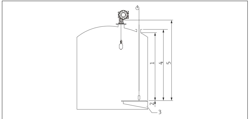
图 47 罐体高度
