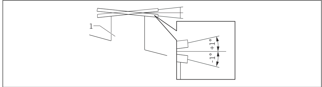
图 11 安装法兰的允许倾角
