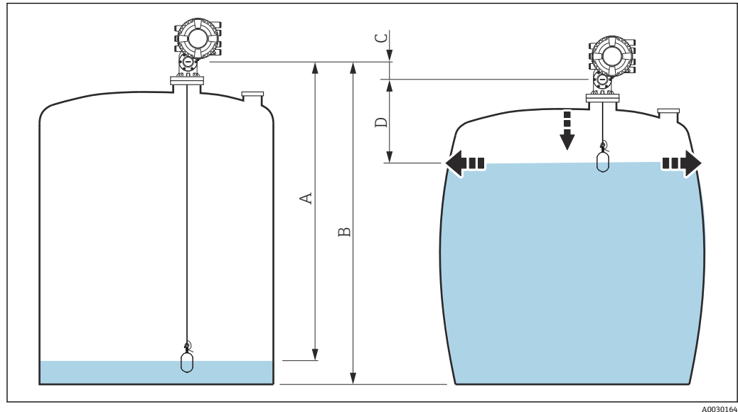
图 65 静压式储罐变形校正值 (HyTD)
