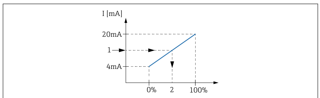
图 61 4...20 mA 输入对应过程变量
