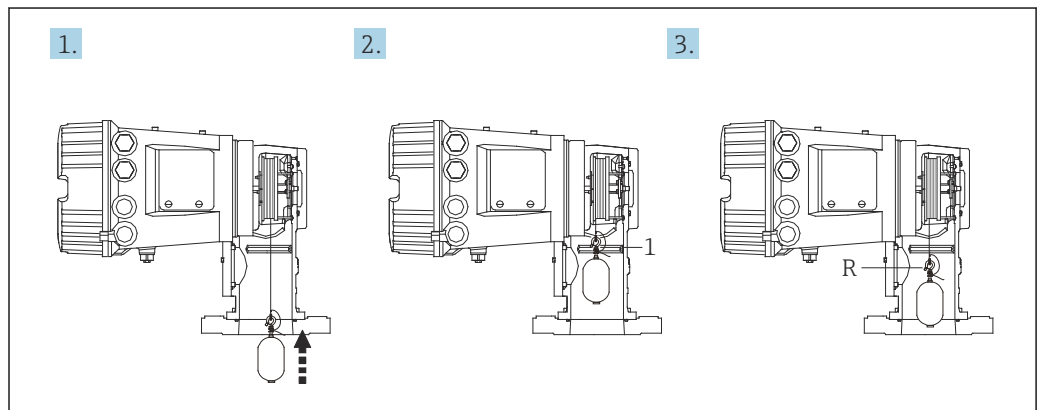
图 44 参考标定步骤
