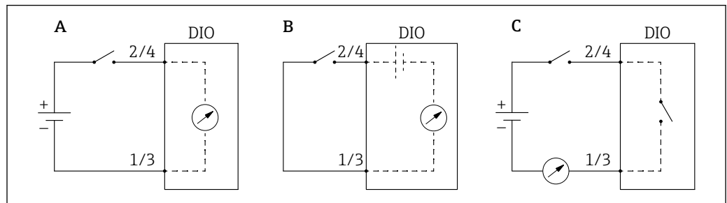
图 91 数字量输入/输出模块的工作模式
