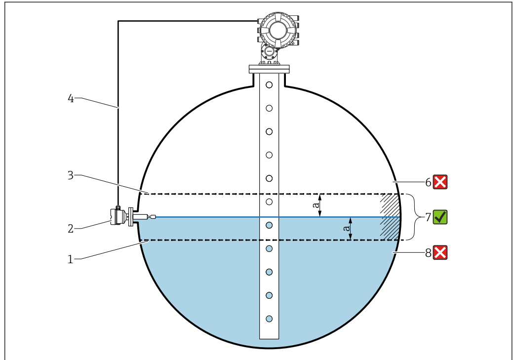
图 67 带液位开关的应用实例
