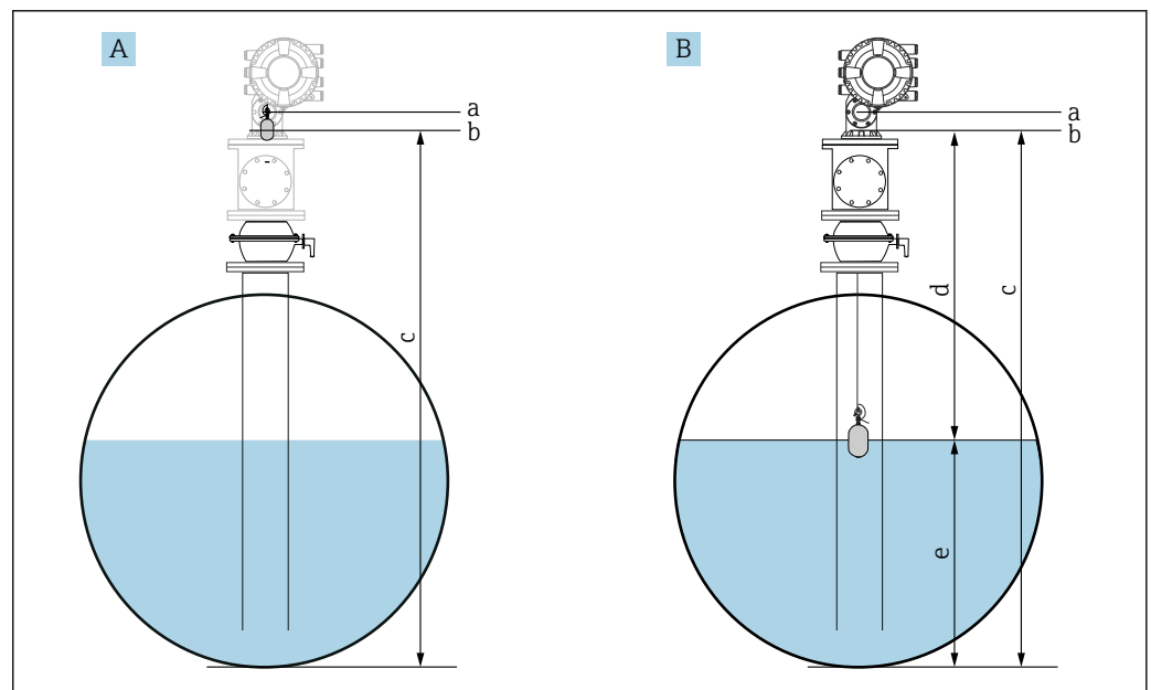
图 51 空罐液位设置示意图 (NMS80/81)
