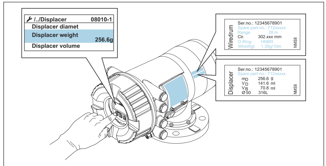
图 41 验证数据
