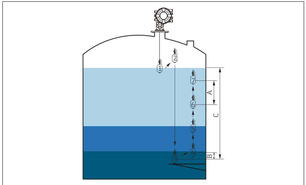
图 54 罐体梯度位移（数字显示浮子的移动顺序）示意图
