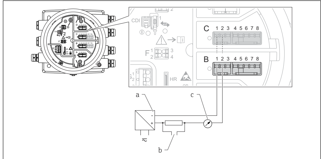
图 21 输出模式下的无源模拟量输入/输出模块
