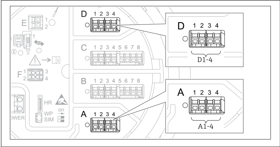
36 A „Modbus” vagy „V1” modulok lehetséges helyei (példák); a készülék verziójától függően ezek a modulok a B vagy a C modulfoglalatban is lehetnek.
