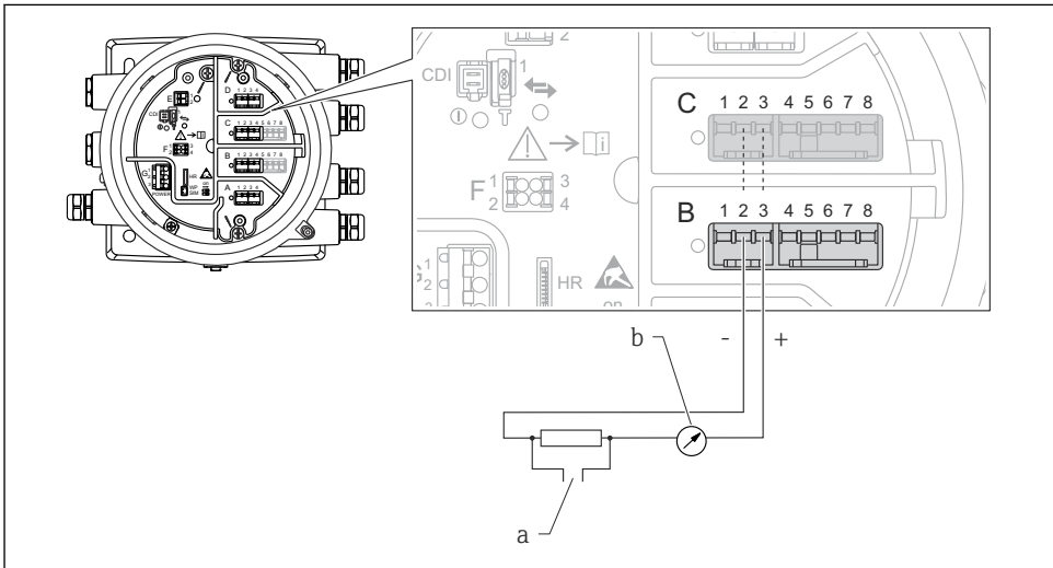
15 Az analóg I/O modul aktív használata kimeneti módban
