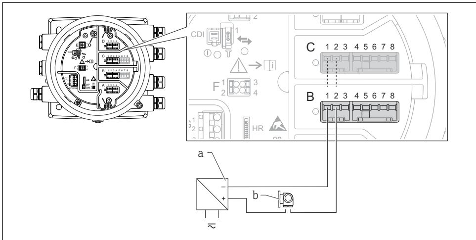
13 Az analóg I/O modul passzív használata bemeneti módban
