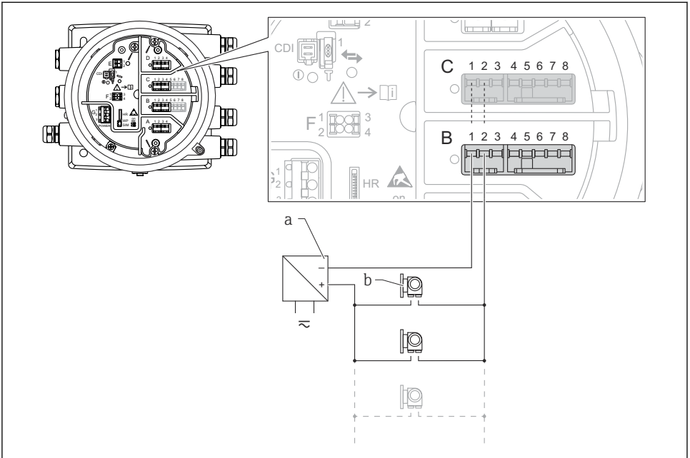
图 14 HART 主站模式下的无源模拟量输入/输出模块
