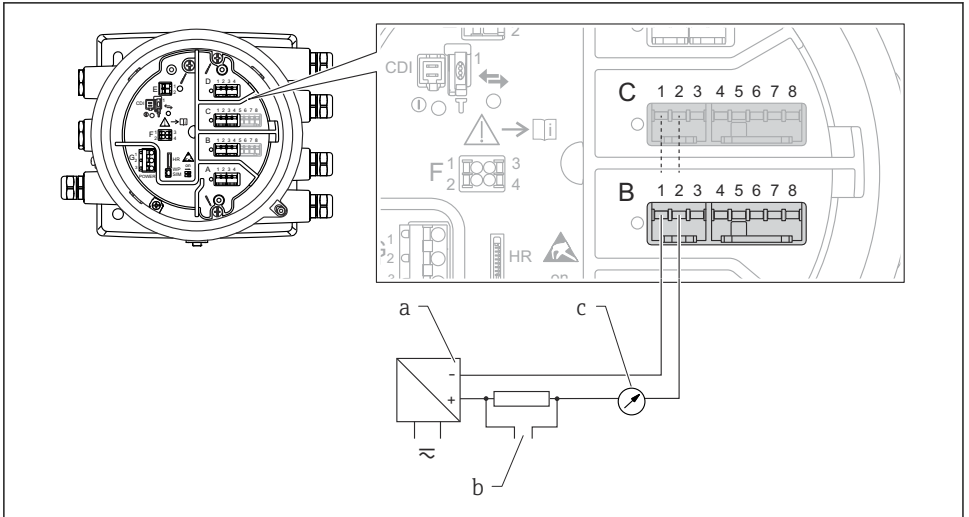
图 12 输出模式下的无源模拟量输入/输出模块
