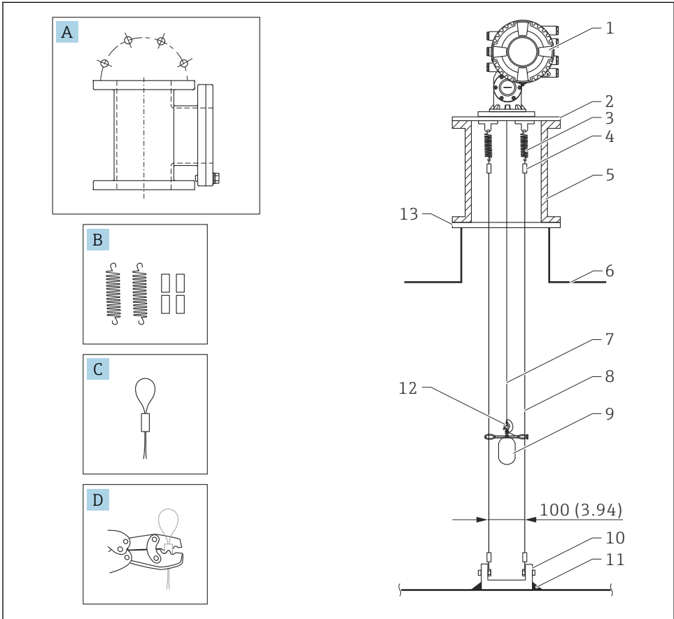
图 3 导向钢丝；单位：mm (in)
