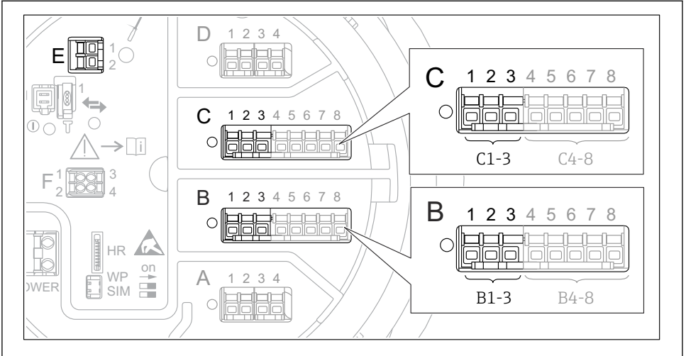
图 29 HART 回路的可能接线端子
