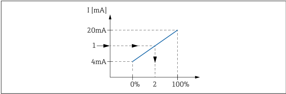
图 31 4...20 mA 输入对应过程变量
