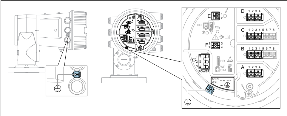
图 8 端子接线腔（典型实例）和接地端子示意图
