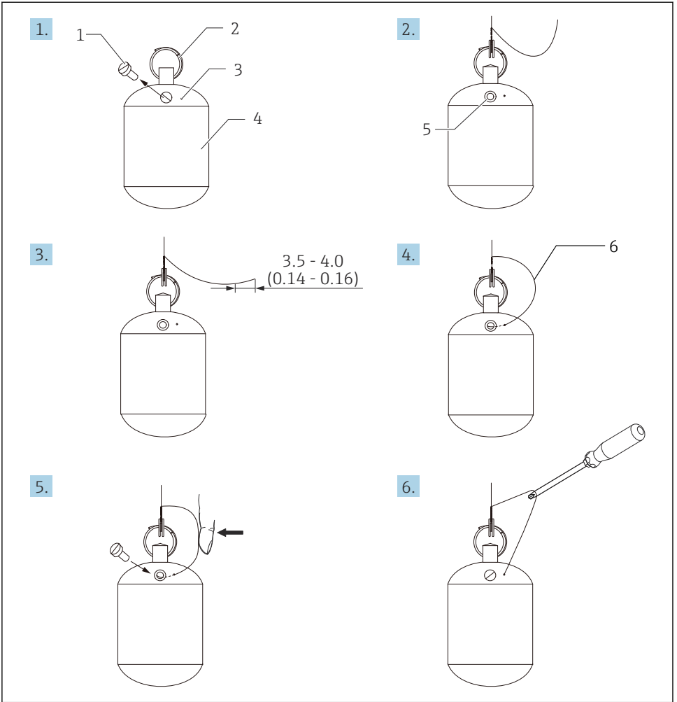
图 7 PTFE 材质型浮子的安装示意图；单位：mm (in)
