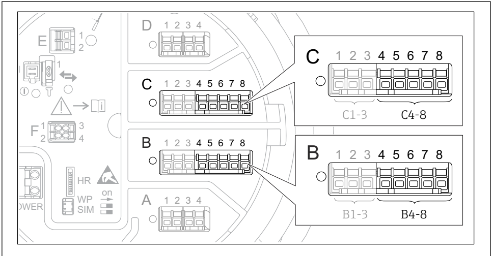
图 32 已连接 RTD 的模拟量输入/输出模块的可能安装位置。设备的订货号确定当前使用的模块。
