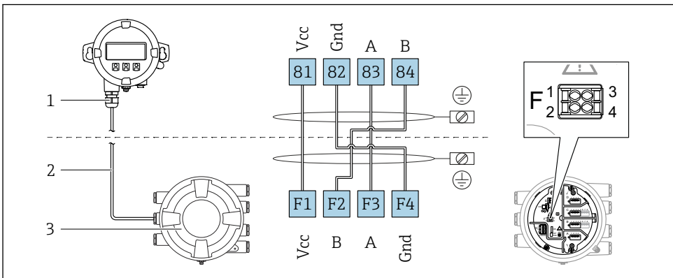
图 10 分离型显示单元与操作单元 DKX001 连接至伺服罐表设备 (NMR8x、NMS8x 或 NRF8x)
