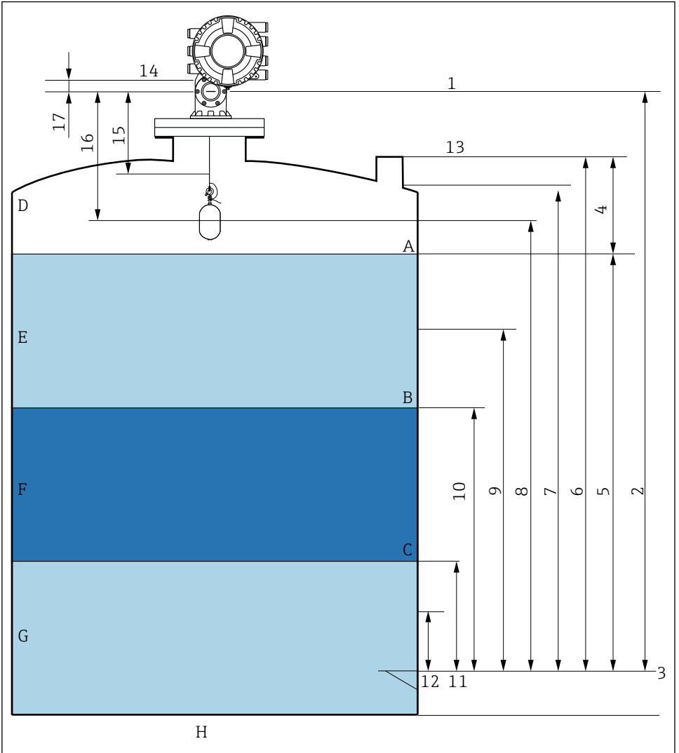
图 23 NMS8x 安装术语 (例如 NMS81)
