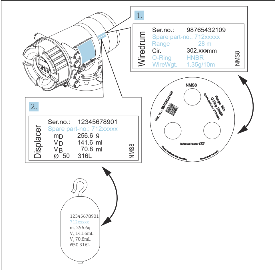
4 验证浮子和轮鼓
