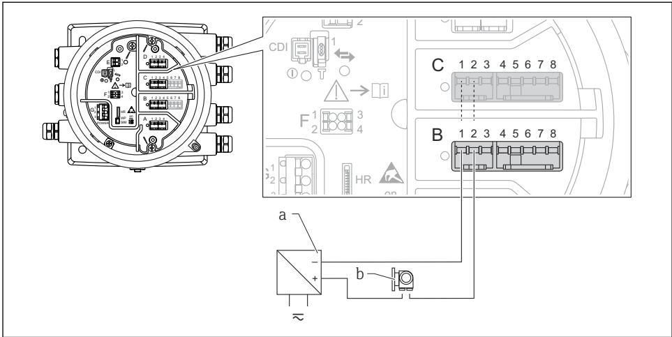
图 13 输入模式下的无源模拟量输入/输出模块
