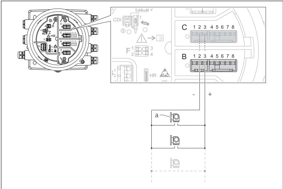
图 17 HART 主站模式下的有源模拟量输入/输出模块
