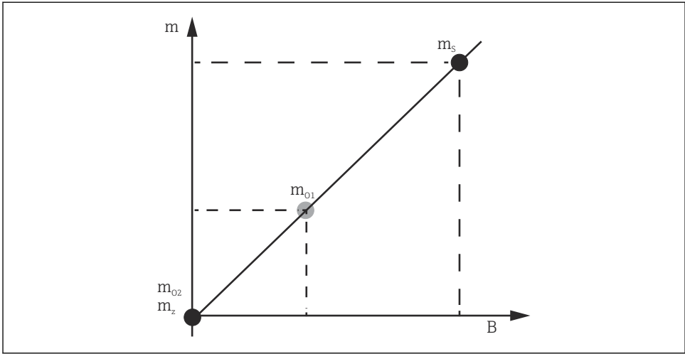
图 26 传感器标定原理
