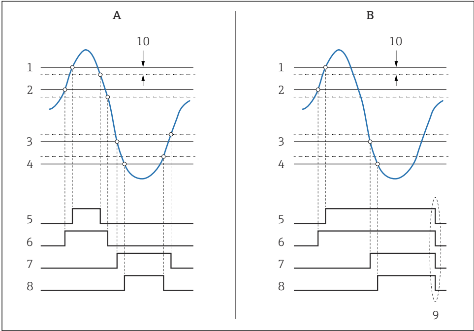
34 限定值计算原理
