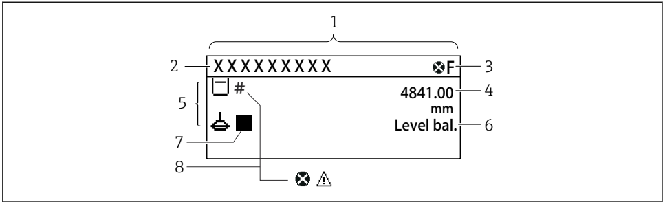
图 20 典型的标准显示界面（测量值显示）
