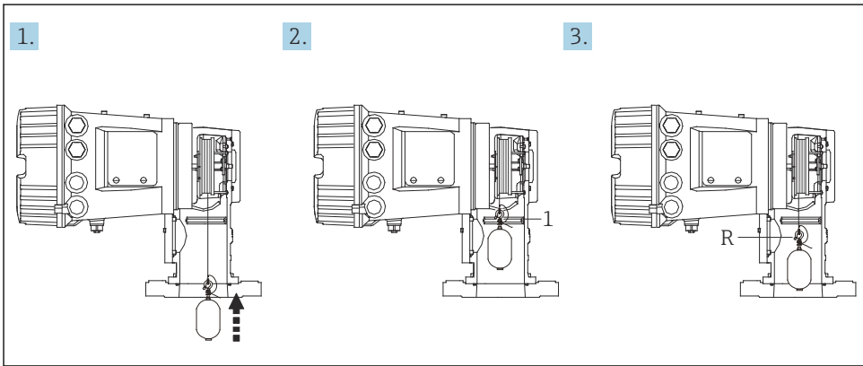
图 27 参考标定步骤
