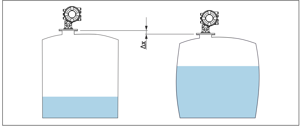
24 Movimenti \Delta x del livello di riferimento del serbatoio che si generano per la deformazione delle pareti del serbatoio causata dalla pressione idrostatica
