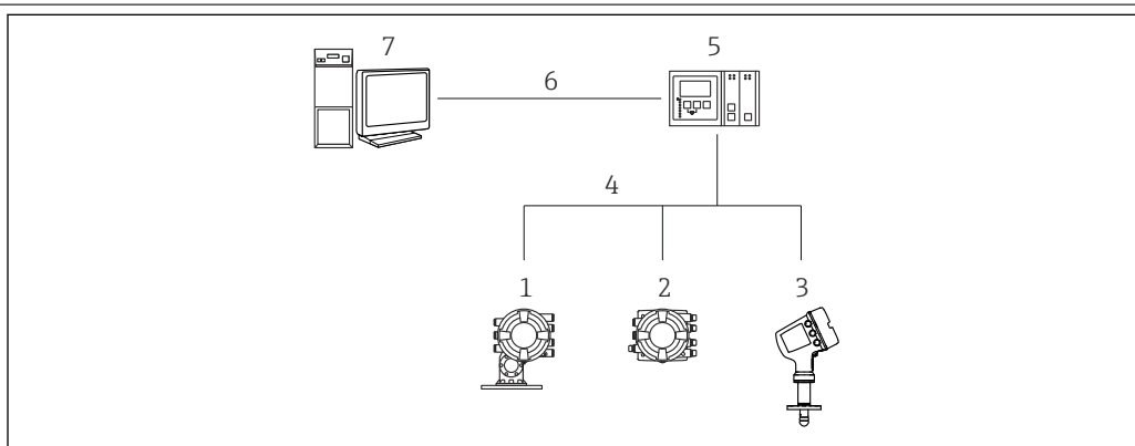
22 Comando a distanza dei dispositivi di misura nei serbatoi
