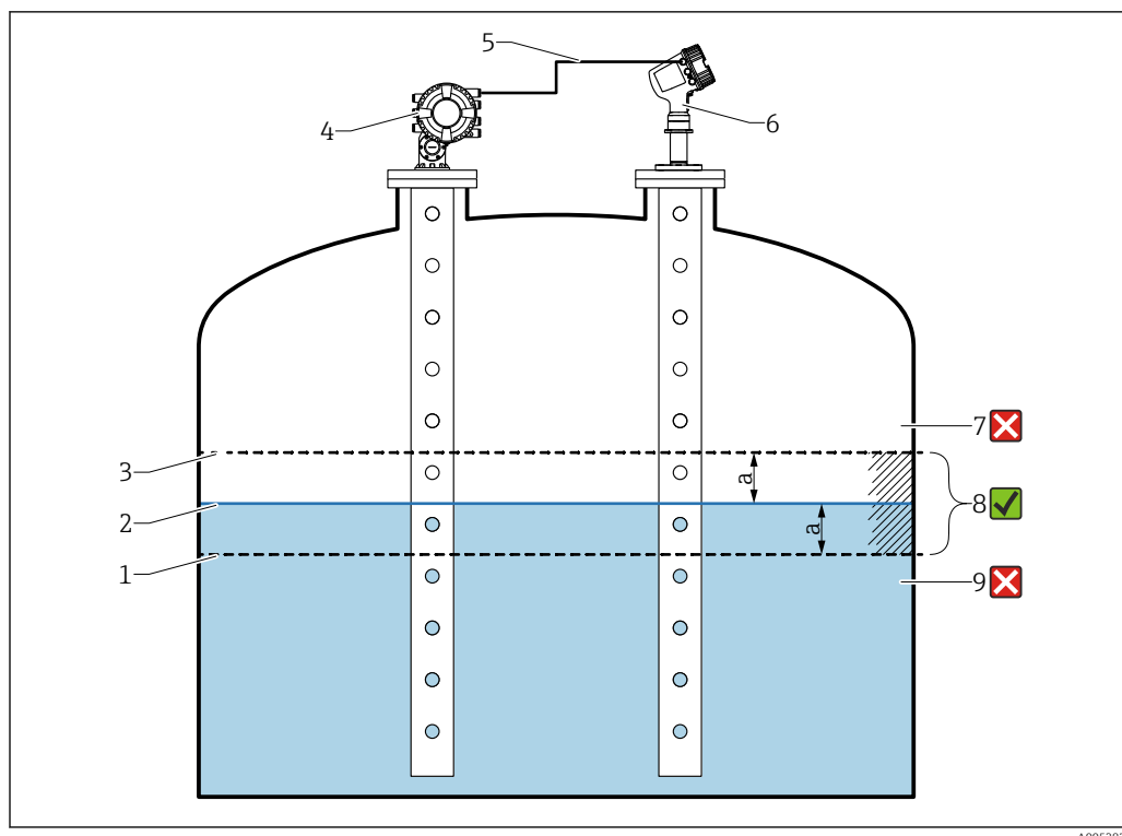
25 Esempio di applicazione con Proservo NMS8x
