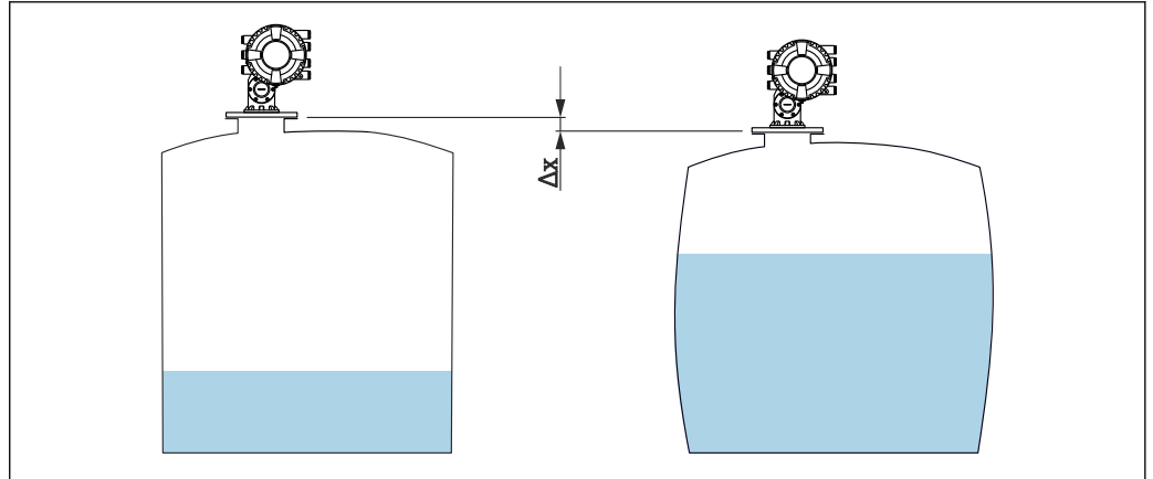
24 Movimento \Delta x da altura de referência do tanque devido ao abaulamento do tanque causado pela pressão hidrostática
