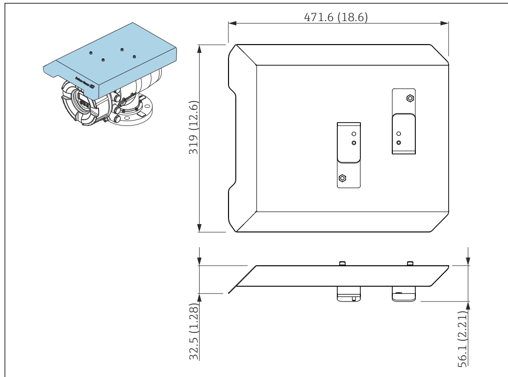
27 Tampa de proteção contra tempo, dimensões: mm (pol.)
