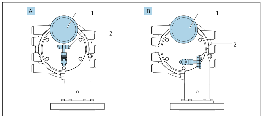
28 Posição de instalação da válvula de alívio e do medidor de pressão
