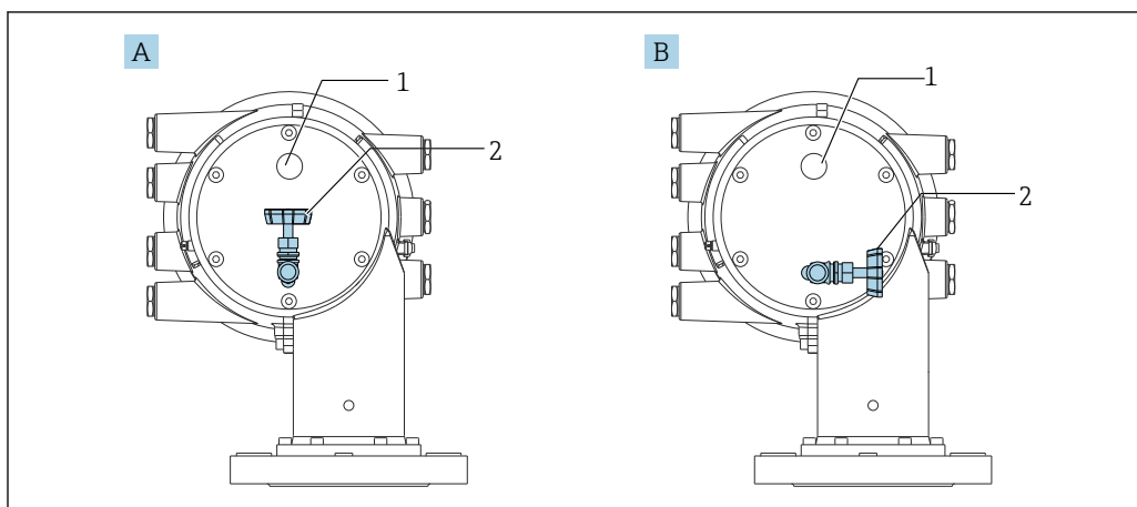
32 Buse de nettoyage et soupape de décharge
