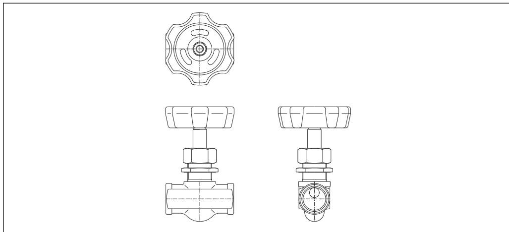
29 Soupape de décharge
