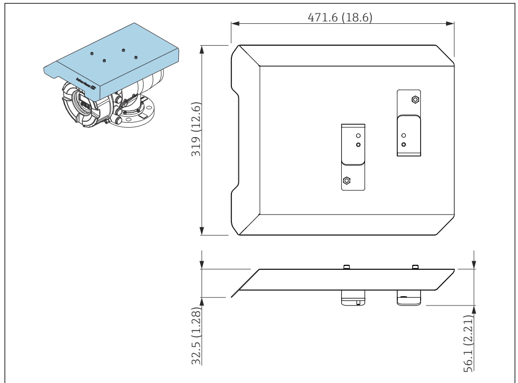
27 Capot de protection climatique ; unité de mesure : mm (in)
