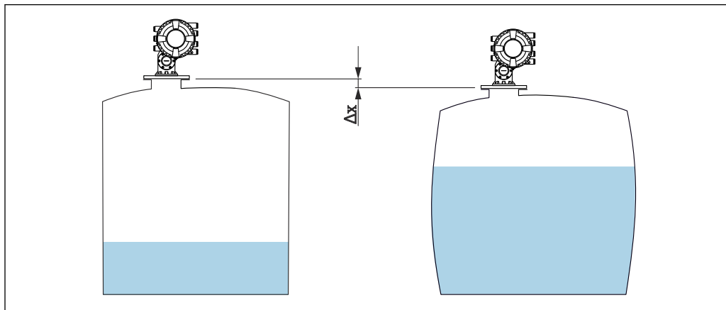
24 Mouvement \Delta x de la hauteur de référence de la cuve dû au gonflement de la paroi du réservoir engendré par la pression hydrostatique
