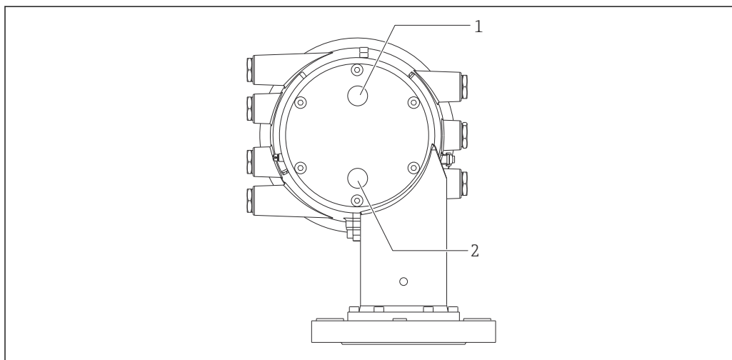
31 Trous pour la buse de nettoyage et la buse de dégazage
