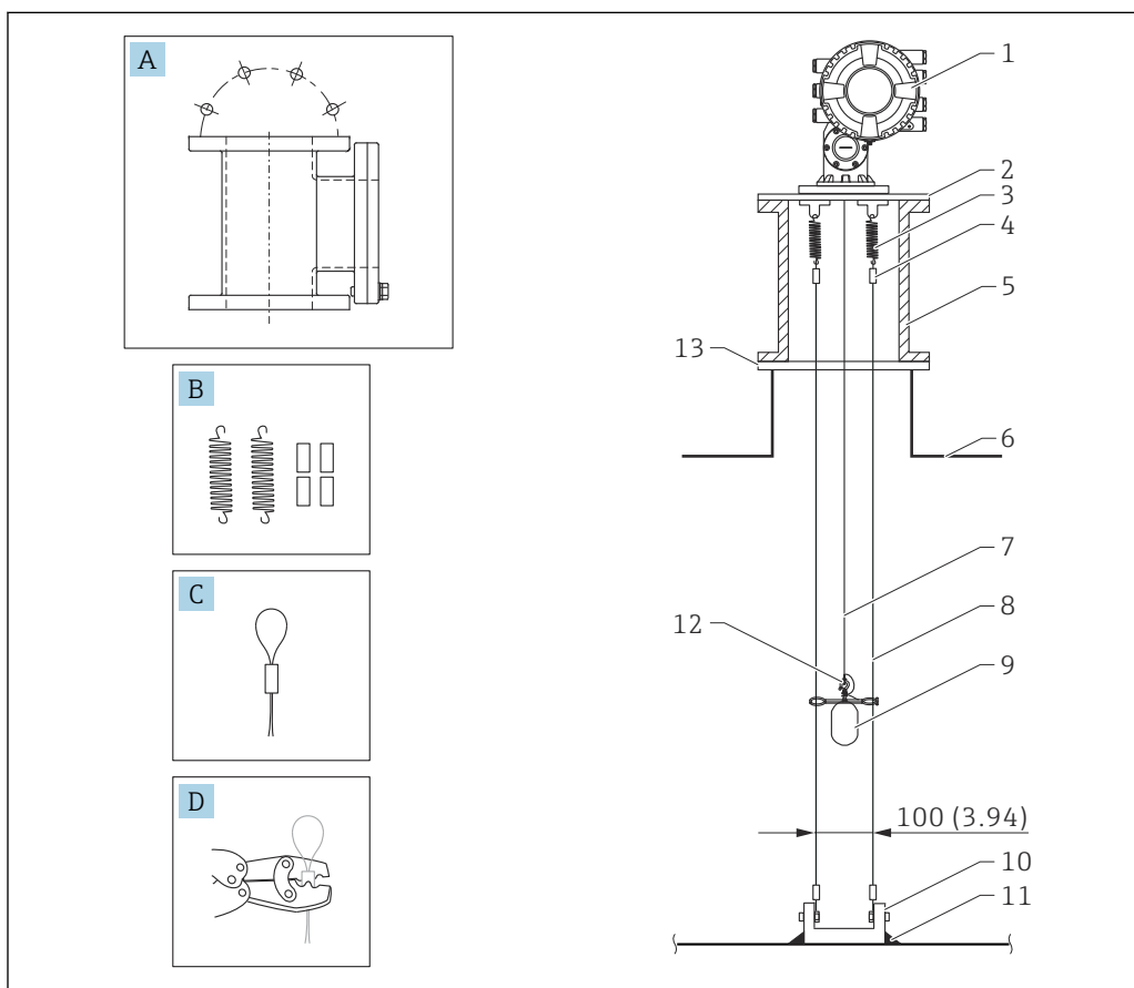
17 Fil guide ; dimensions mm (in)
