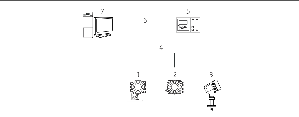
22 Configuración a distancia de equipos de medición de depósitos
