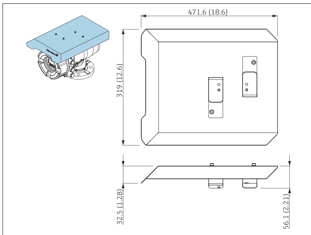
27 Tapa de protección ambiental, medidas: mm (in)
