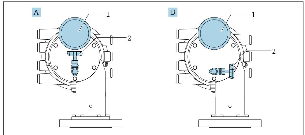
28 Posición de montaje de la válvula de descarga y el medidor de presión
