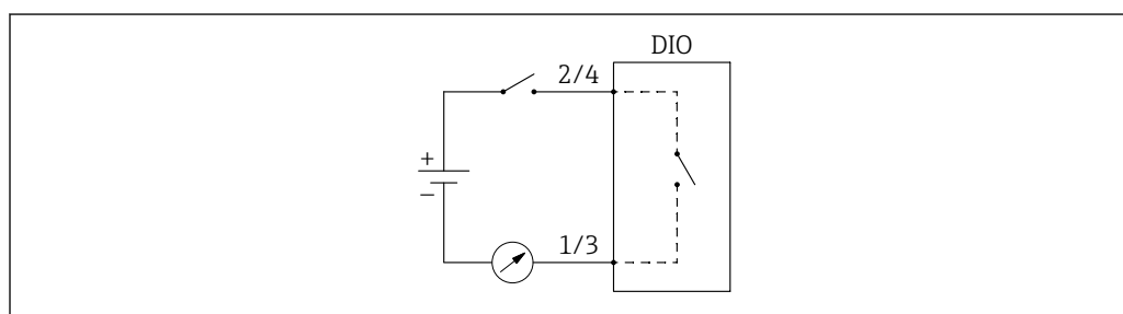
46 Uso del módulo E/S digital como salida digital
