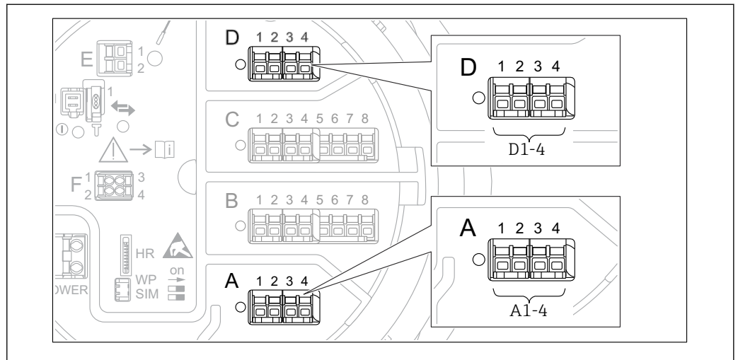
7 Designación de los módulos "Modbus", "V1" o "WM550" (ejemplos); según la versión del equipo, estos módulos también se pueden encontrar en las ranuras B o C.
