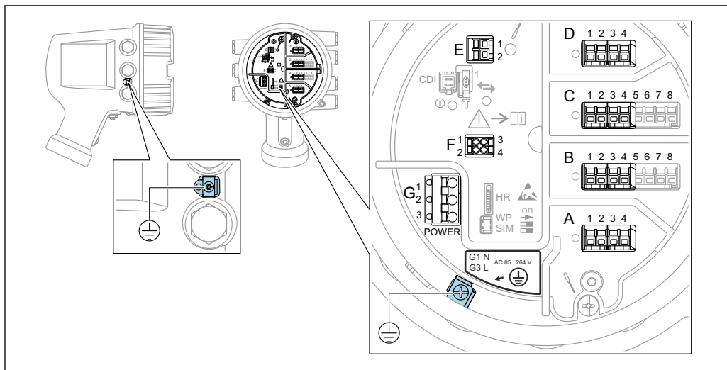
4 Compartimento de terminales (ejemplo típico) y bornes de tierra
