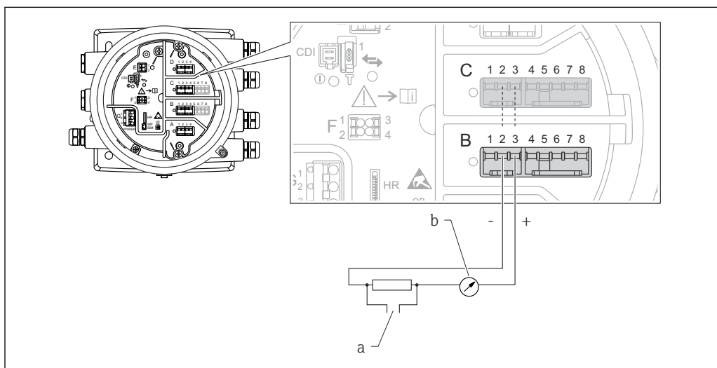
11 Uso activo del módulo de E/S analógica en el modo de salida
