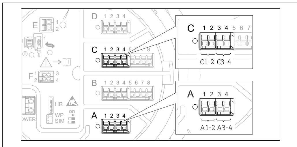
33 Ubicaciones posibles de los módulos E/S digitales (ejemplos); el código de pedido define el número y la ubicación de los módulos de entrada digital → 23.
