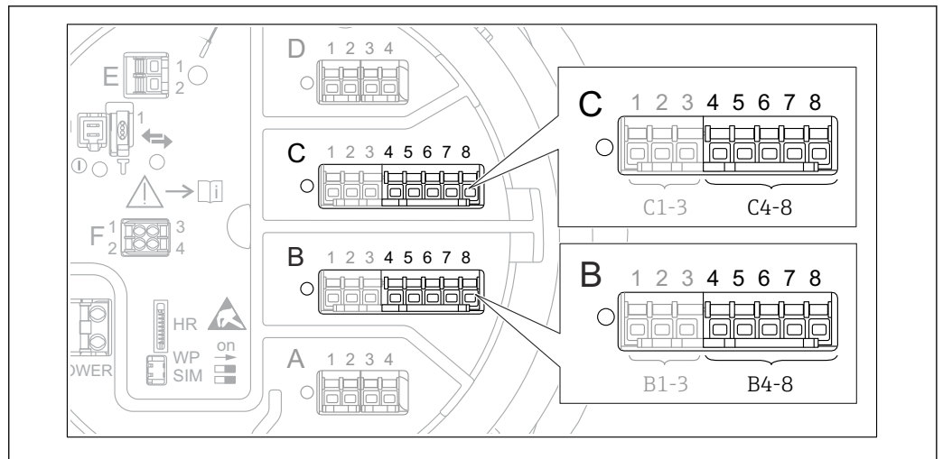
31 Ubicaciones posibles de los módulos E/S analógicos, a los que se puede conectar una RTD. Los módulos que están realmente presentes dependen del código de producto del equipo → 23.
