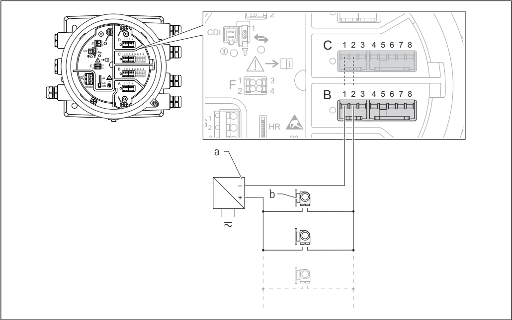
10 Uso pasivo del módulo de E/S analógica en el modo maestro HART
