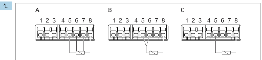
32 Tipos de conexión RTD
