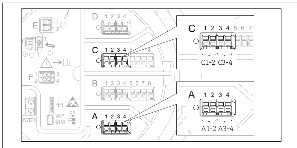
45 Ubicaciones posibles de los módulos E/S analógicos (ejemplos); el código de producto define el número y la ubicación de los módulos E/S digitales → 23.
