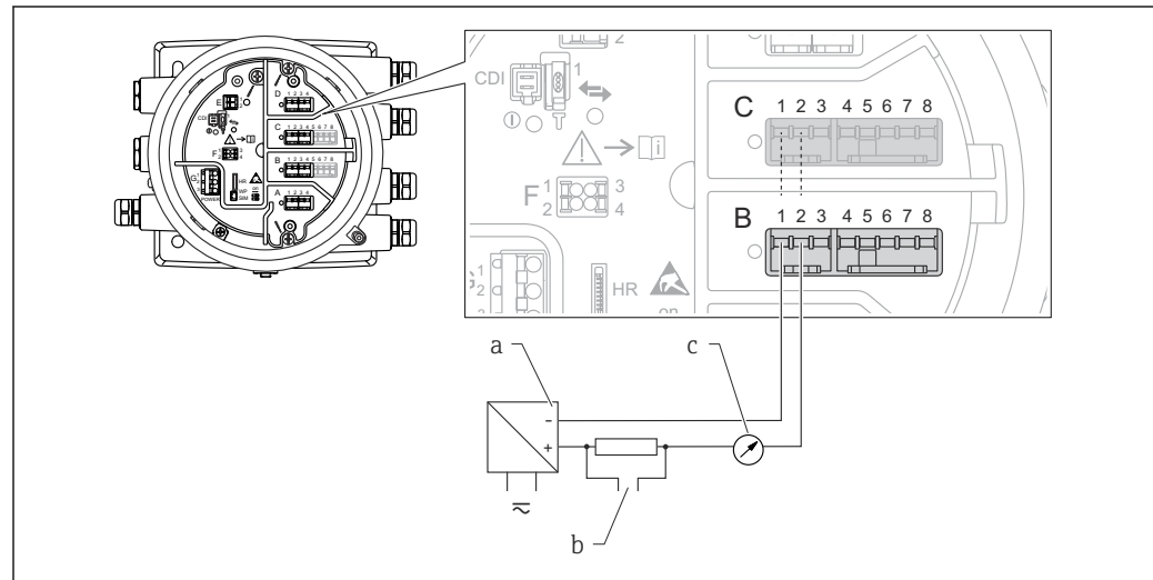
8 Uso pasivo del módulo de E/S analógica en el modo de salida
