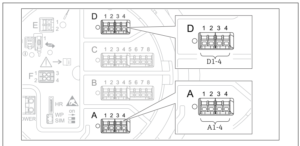
44 Ubicaciones posibles de los módulos WM550 (ejemplos); en función de la versión del equipo, estos módulos también pueden ocupar las ranuras B o C → 23.
