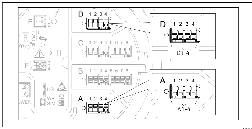
42 Ubicaciones posibles de los módulos Modbus (ejemplos); en función de la versión del equipo, estos módulos también pueden ocupar las ranuras B o C → 23 .
