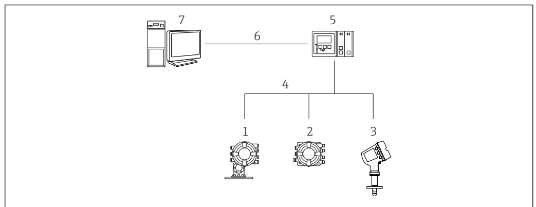
24 Conectar equipos de medición de tanques a FieldCare mediante Tankvision Tank Scanner NXA820
