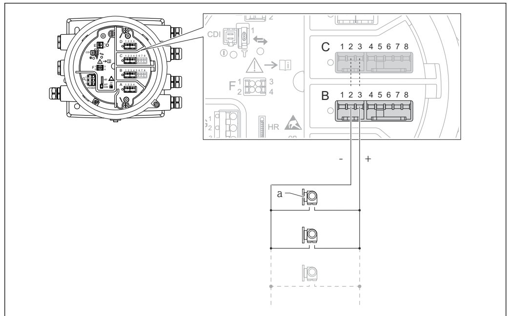
13 Uso activo del módulo de E/S analógica en el modo maestro HART
