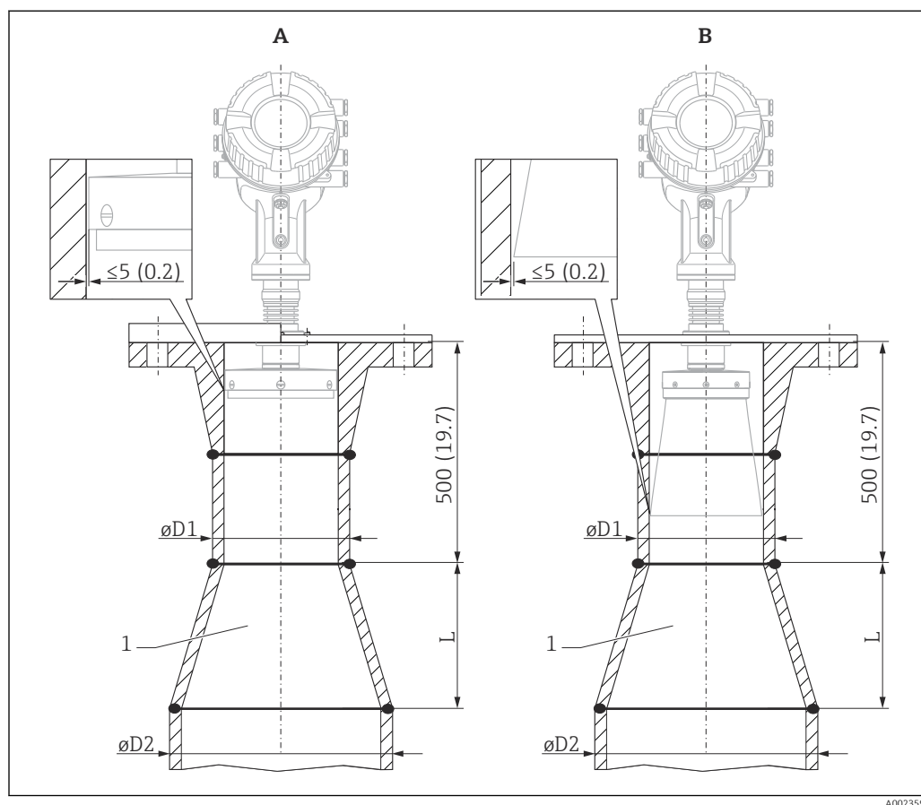
3 Instalación del NMR84 en tubos tranquilizadores de diámetro mayor
