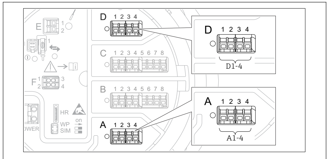
43 Ubicaciones posibles de los módulos V1 (ejemplos); en función de la versión del equipo, estos módulos también pueden ocupar las ranuras B o C → 23.
