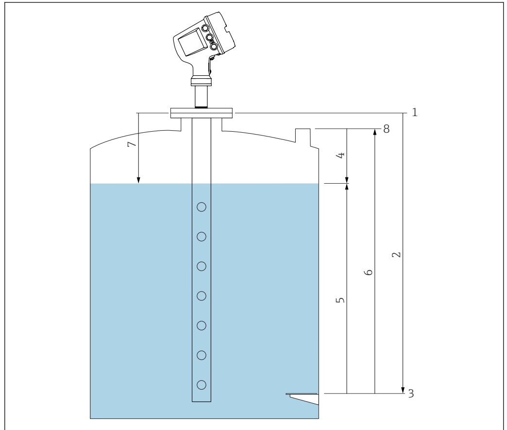
25 Términos relativos a la medición de depósitos por radar
