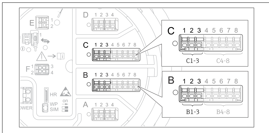
29 Ubicaciones posibles de los módulos E/S analógicos, que pueden utilizarse como entrada 4-20 mA. Los módulos que están realmente presentes dependen del código de producto del equipo → 23.
