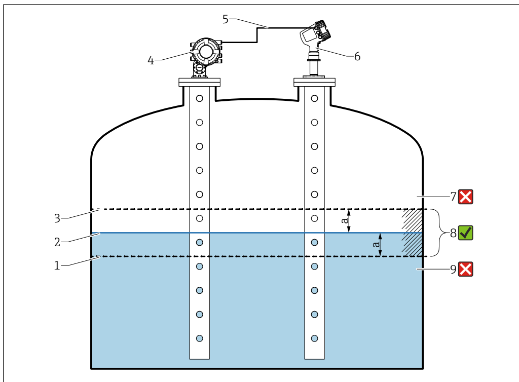
35 Ejemplo de aplicación con Proservo NMS8x
