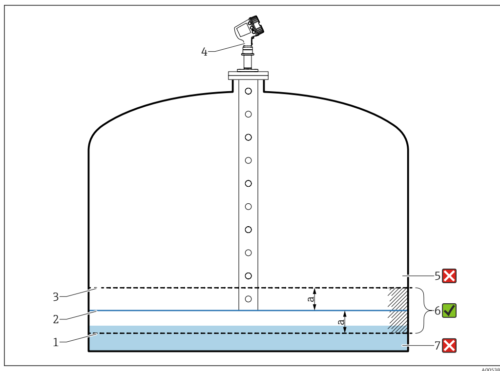
36 Ejemplo de aplicación con punto de referencia fijado en el extremo del tubo tranquilizador
