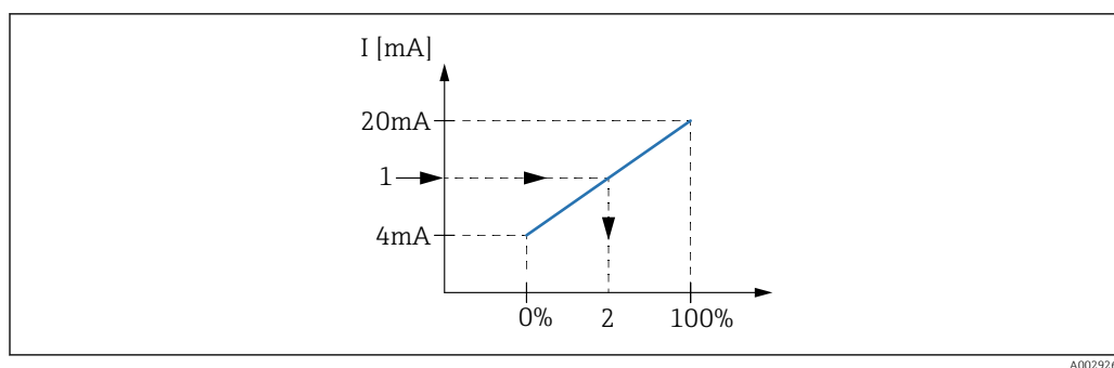
30 Escalado de la entrada 4-20 mA a la variable de proceso
