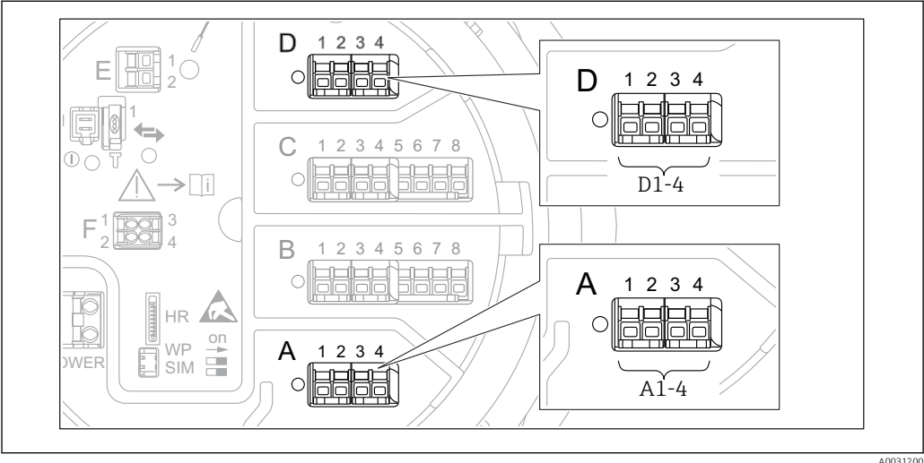
54 Designación de los módulos "Modbus", "V1" o "WM550" (ejemplos); según la versión del equipo, estos módulos también se pueden encontrar en las ranuras B o C.
