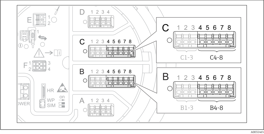
49 Terminales para el Submenú "Analog IP" ("B4-8" o "C4-8", respectivamente)
