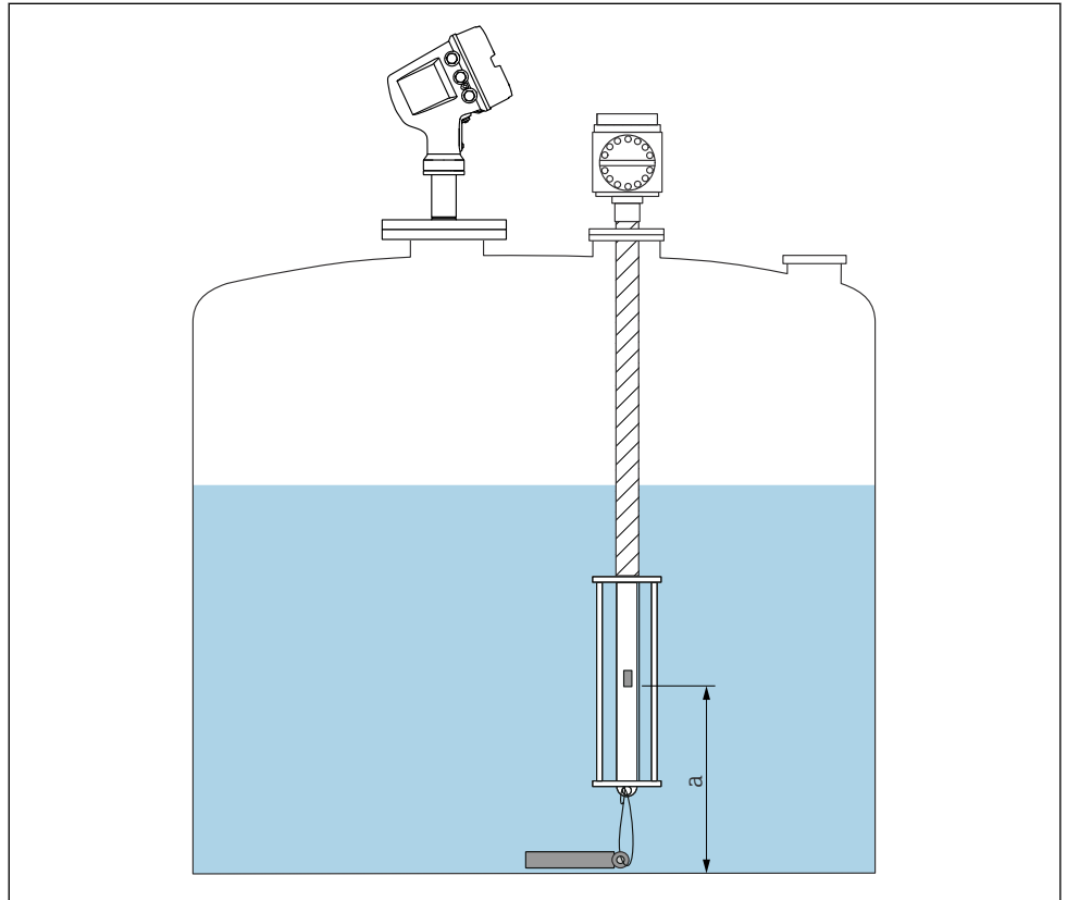
27 Prothermo NMT53x: posición del elemento de temperatura inferior
