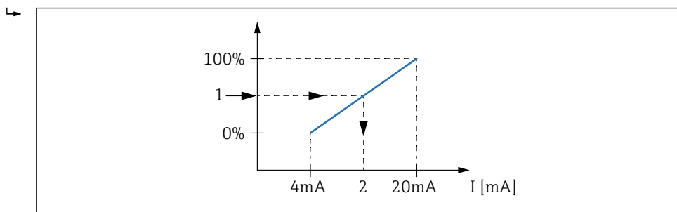
40 Escalado de la variable del depósito a la corriente de salida
