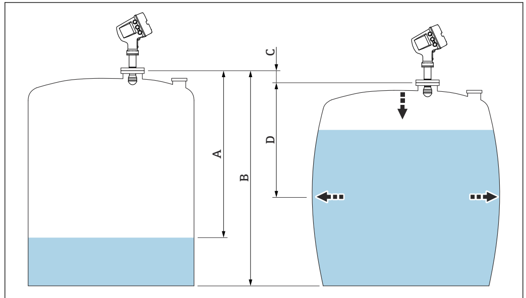
34 Corrección de la deformación hidrostática de depósitos (HyTD)
