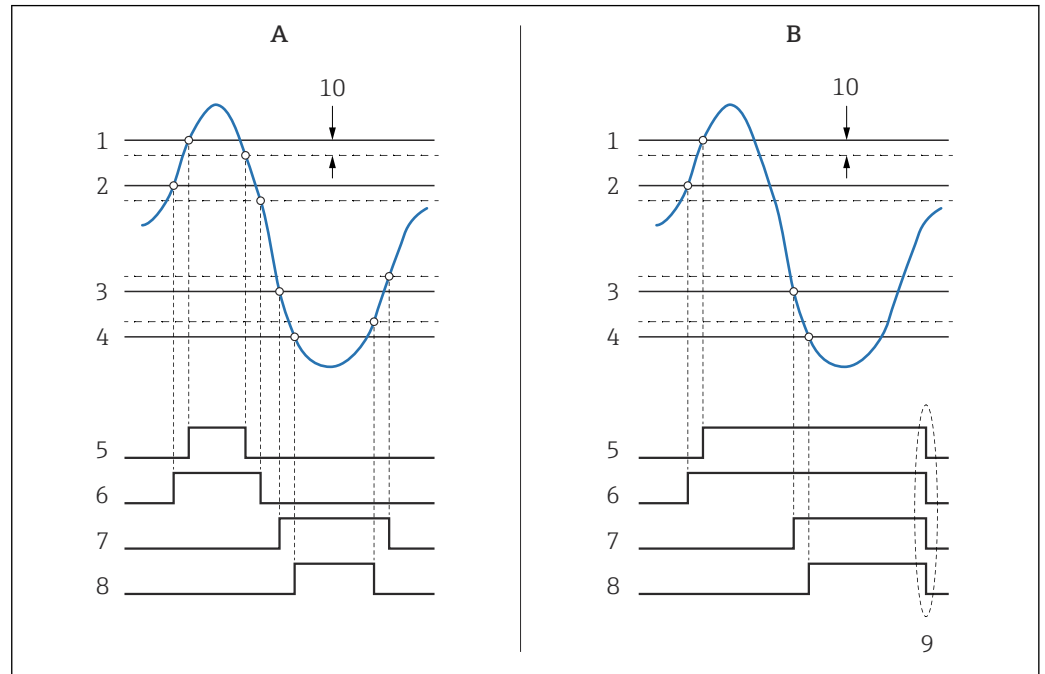
38 Principio de la evaluación de límites
