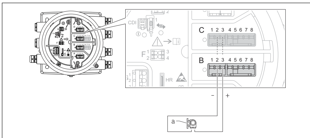
12 Uso activo del módulo de E/S analógica en el modo de entrada
