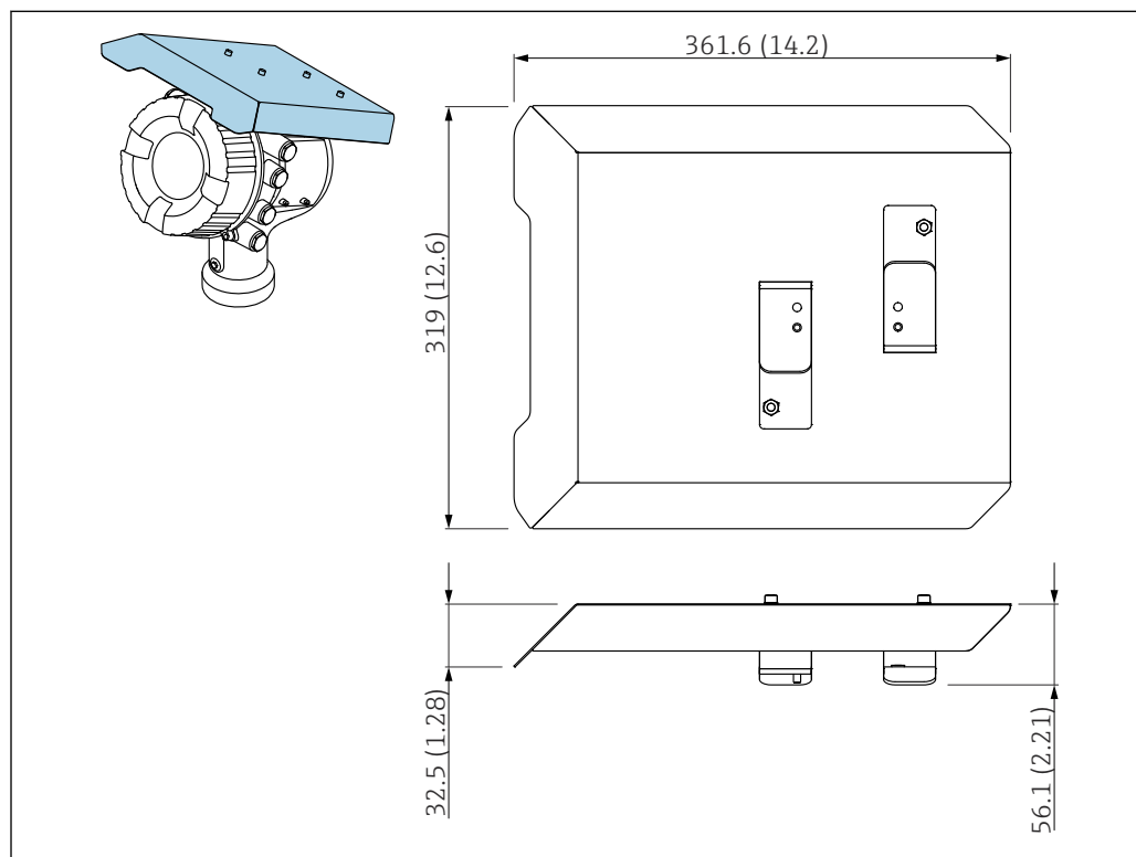
48 Tapa de protección ambiental, medidas: mm (in)
