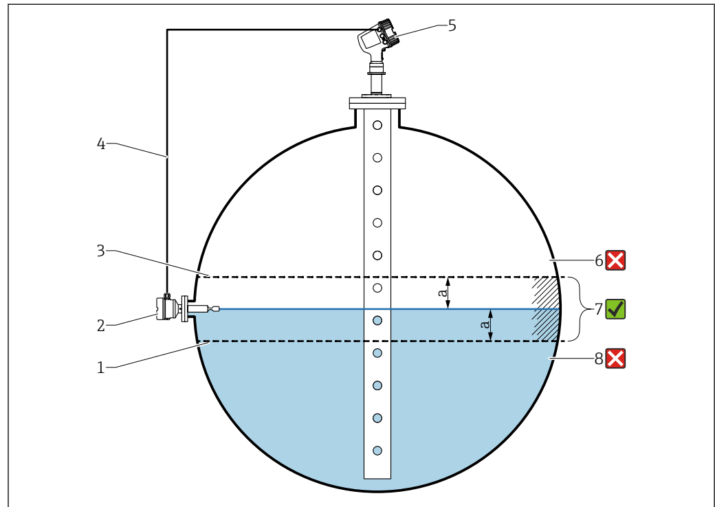
图 37 带液位开关的应用实例
