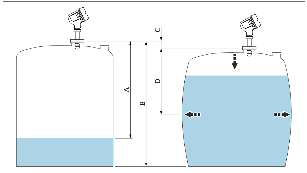
图 34 静压式储罐变形校正值 (HyTD)
