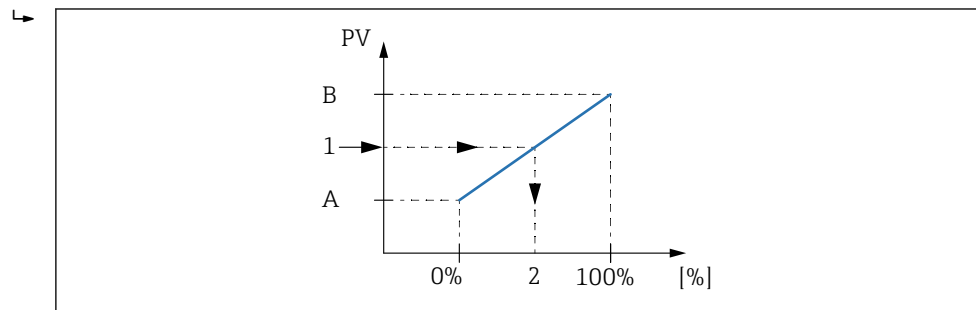
图 41 按百分比调整罐体参数
