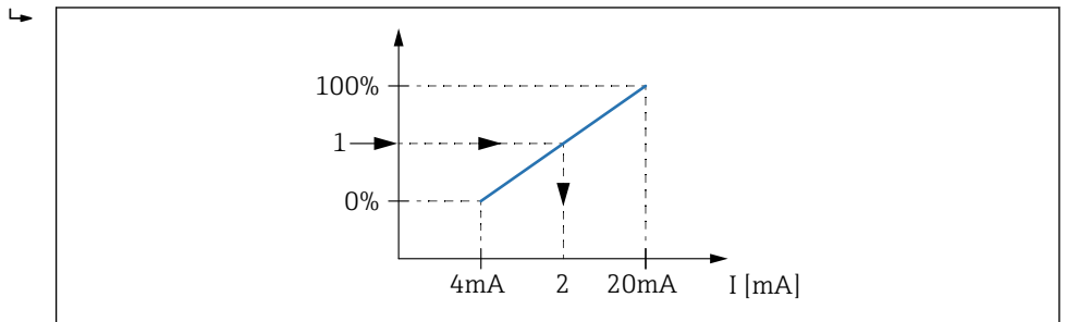
图 40 按输出电流调整罐体参数
