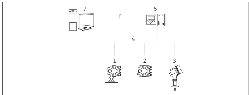
图 24 通过 Tankvision 储罐扫描仪 NXA820 连接伺服罐表设备至 FieldCare
