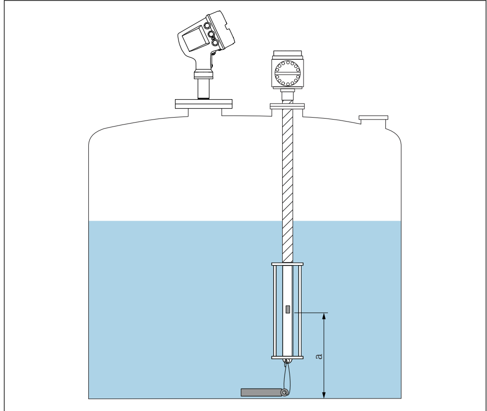
图 27 Prothermo NMT53x: 罐底测温元件位置
