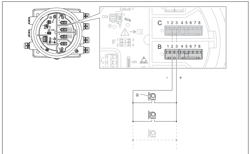
图 13 HART 主站模式下的有源模拟量输入/输出模块
