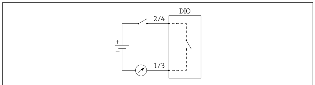
图 46 数字量输入输出模块用作数字量输出
