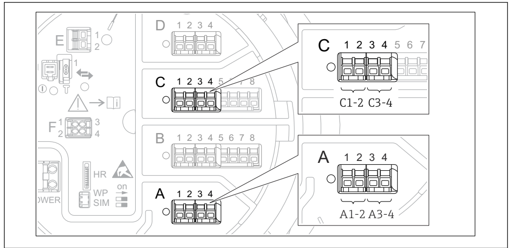
图 33 数字量输入/输出模块的可能安装位置 (示例) ; 订货号确定数字量输入模块的数量和位置→ 20。
