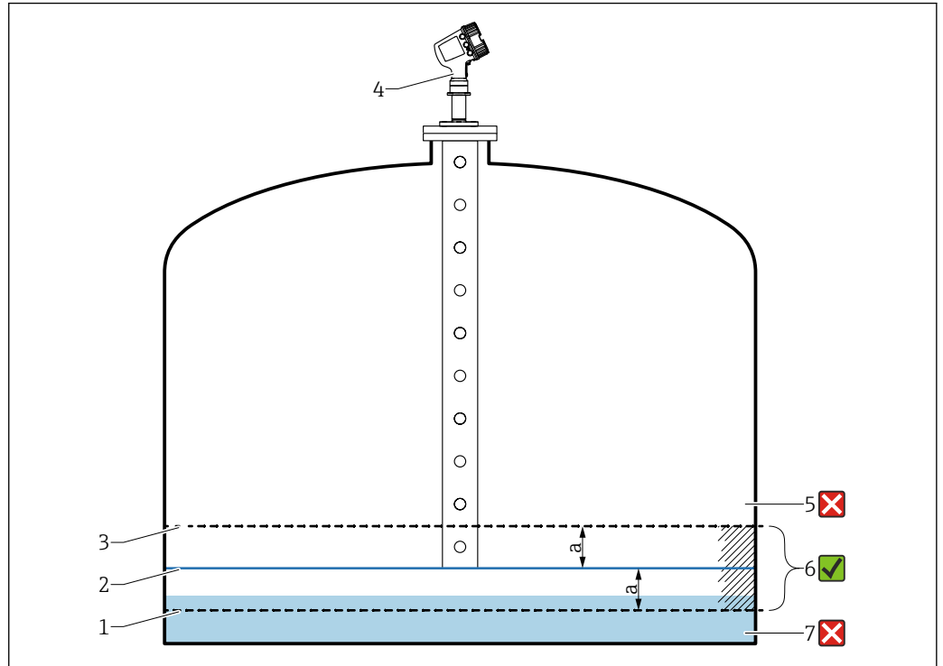
图 36 导波管末端固定参考点的应用实例
