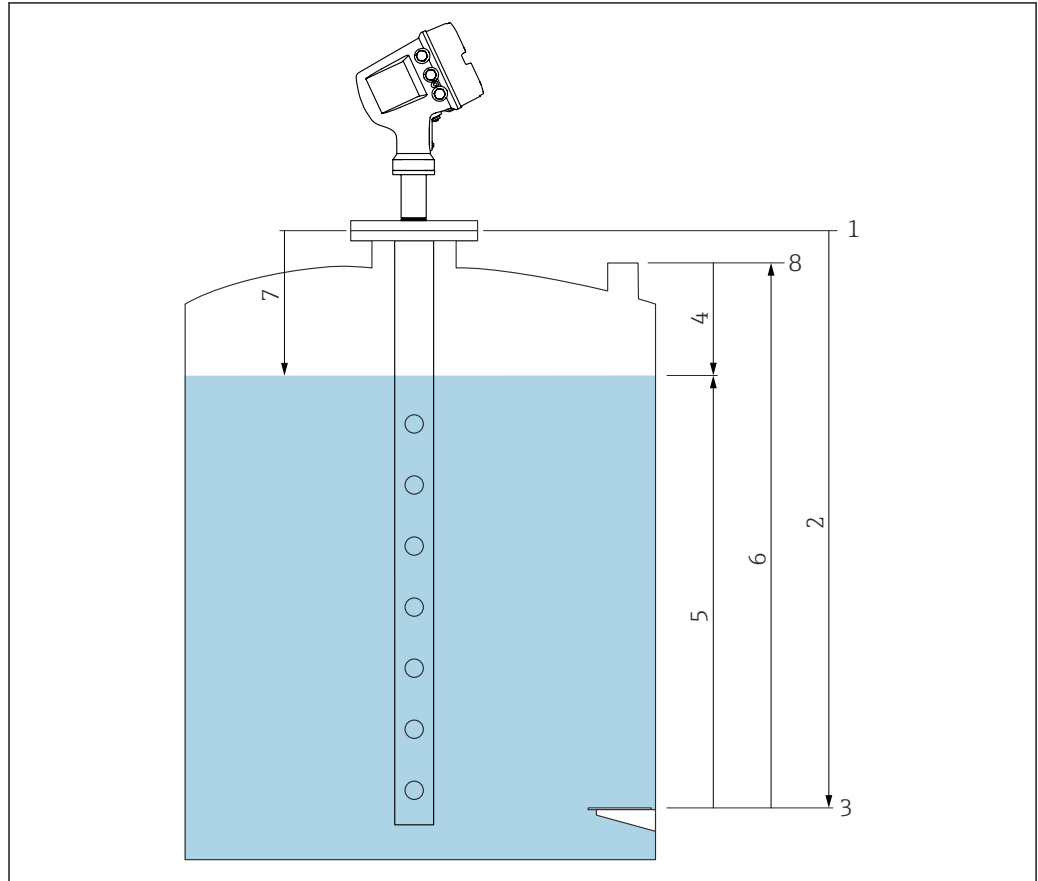
图 25 雷达罐体测量术语
