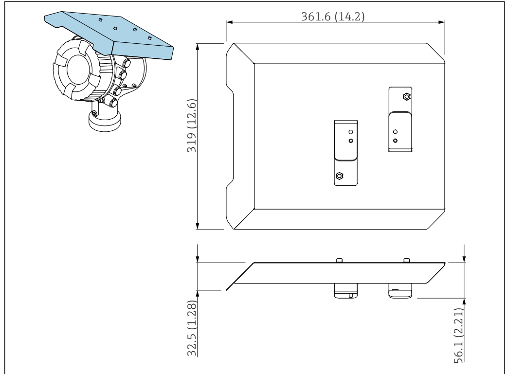
图 48 防护罩的外形尺寸示意图；单位：mm (in)
