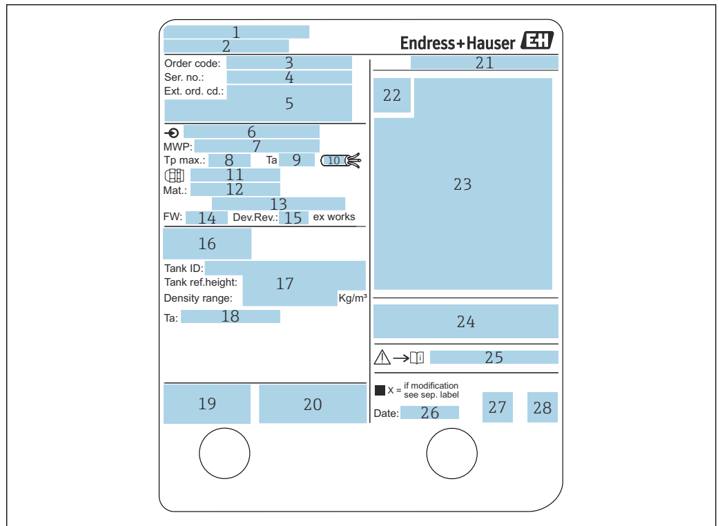
图 2 铭牌
