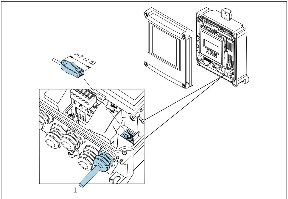
1 Serviceschnittstelle (CDI-RJ45)
