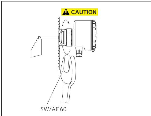
☐ 2 계기 설치
