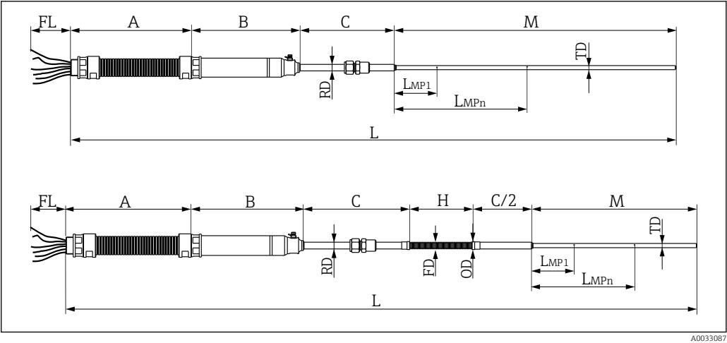
6 Starre und flexible Bauform des modularen Multipoint-Thermometers. Alle Abmessungen in mm (in)
