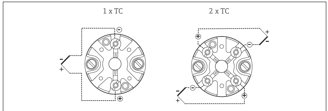
2 Montierter Anschlussklemmenblock
