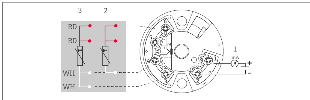
3 Im Anschlusskopf montierter Transmitter TMT18x (ein Sensoreingang)
