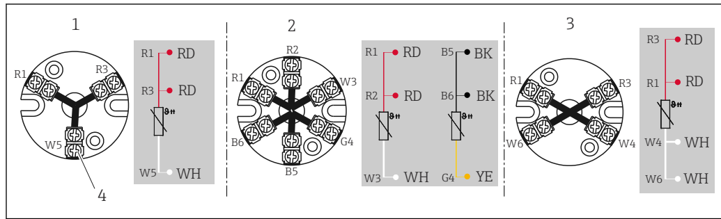
2 Montierter Anschlussklemmenblock
