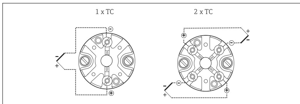
8 Montierter Anschlussklemmenblock
