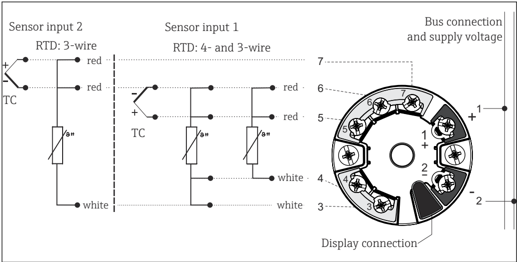
1 Anschlussplan der Kopftransmitter mit dualen Sensoreingang (TMT8x)
