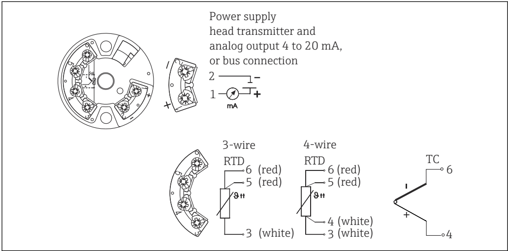
2 Anschlussplan der Kopftransmitter mit einzelem Sensoreingang (TMT18x)
