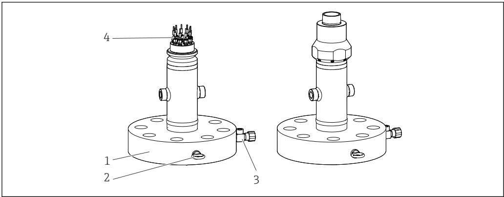
9 Flansch als Prozessanschluss
