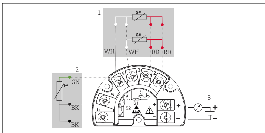
6 Transmetteur de terrain TMT162 (deux entrées)
