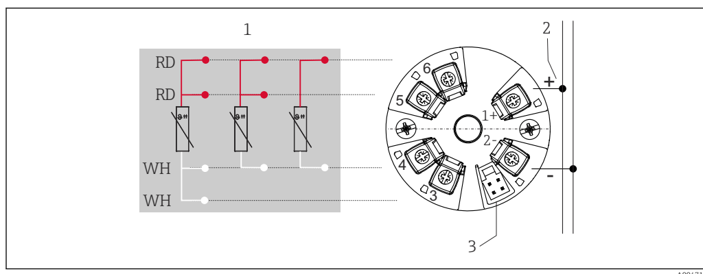
3 Transmetteur monté dans la tête de raccordement TMT31 (une entrée)
