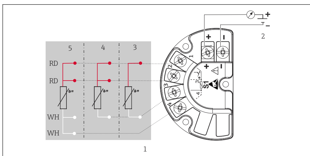
7 Transmetteur de terrain TMT142B (une entrée)
