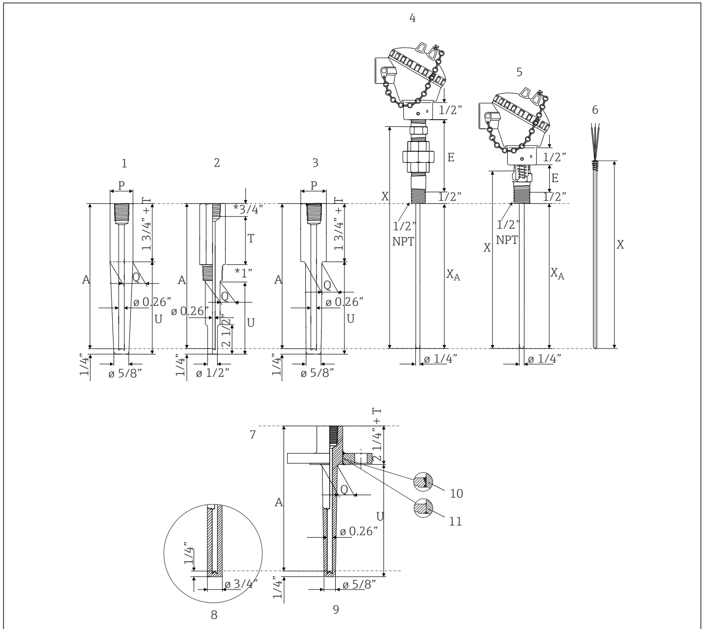
11 Dimensions des unités de capteur.
