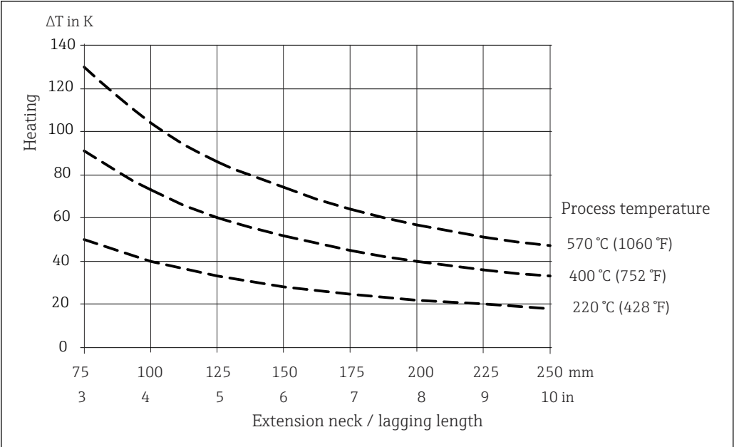
12 Chauffage de la tête de raccordement en fonction de la température du process. Température dans la tête de raccordement = température ambiante 20 °C (68 °F) + ΔT
