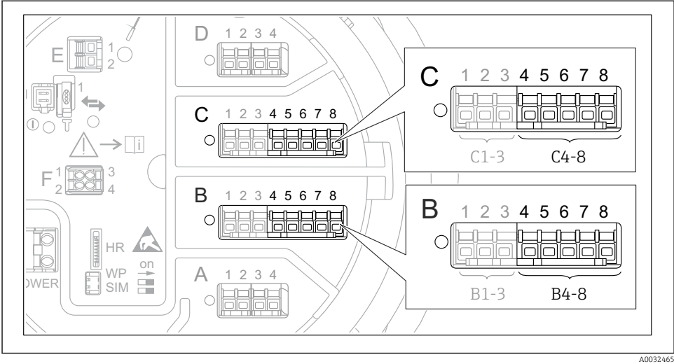
32 Mögliche Positionen der Analog I/O-Module, an die ein Widerstandsthermometer angeschlossen werden kann. Der Bestellcode des Geräts legt fest, welches dieser Module tatsächlich vorhanden ist.
