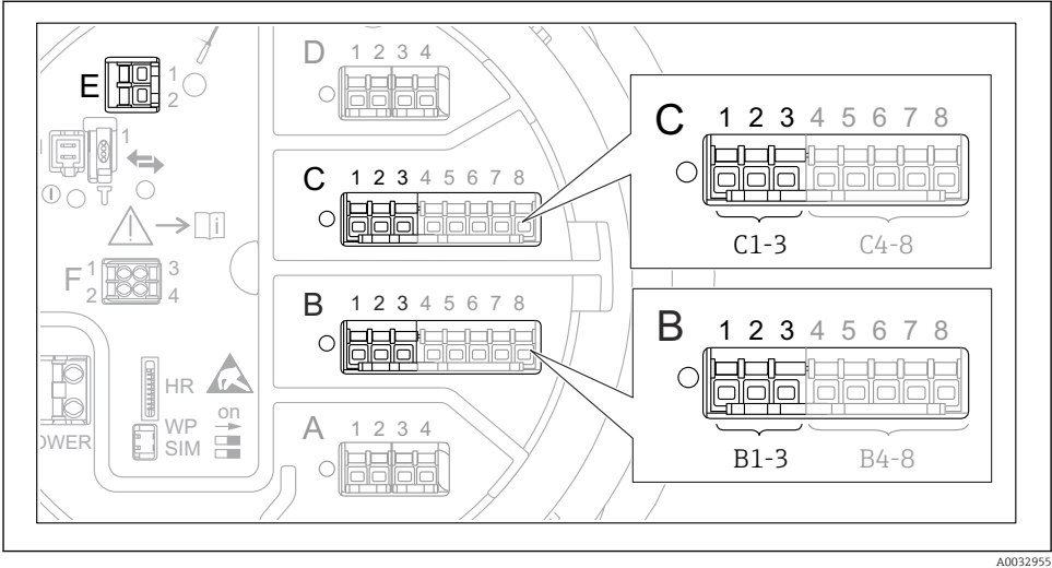
29 Mögliche Anschlüsse für HART-Loops
