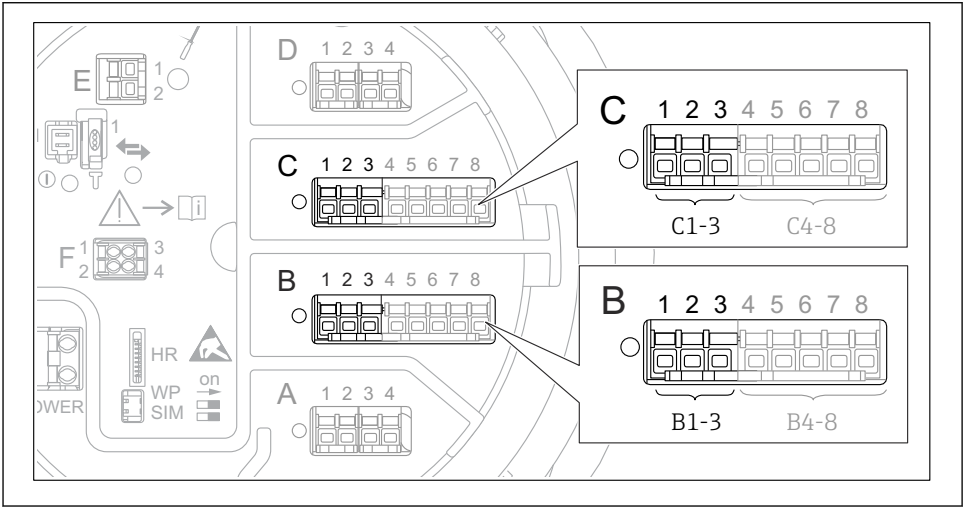
35 Mögliche Positionen der Analog I/O-Module, die als 4 ... 20 mA-Ausgang verwendet werden können. Der Bestellcode des Geräts legt fest, welches dieser Module tatsächlich vorhanden ist.
