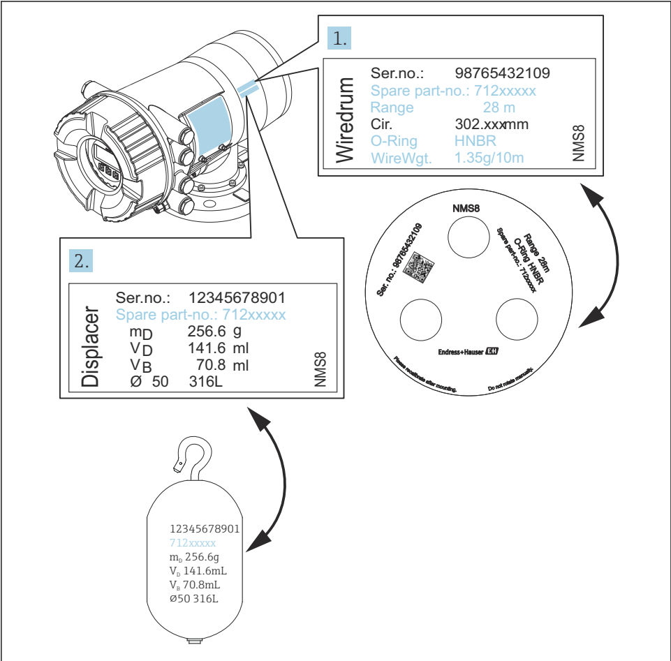
4 Verifikation von Verdränger und Messtrommel
