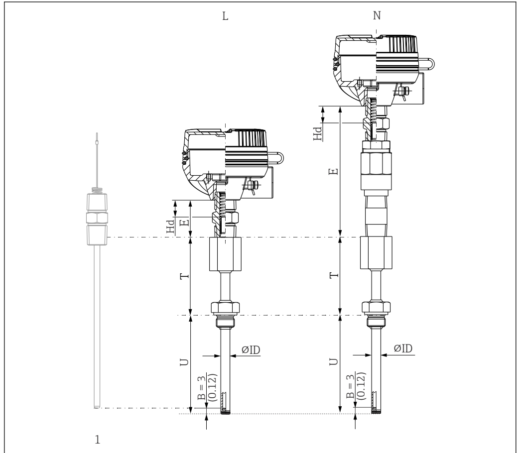
图 22 温度计配置，安装有 TS111 铠装芯子，压簧式对中安装。
