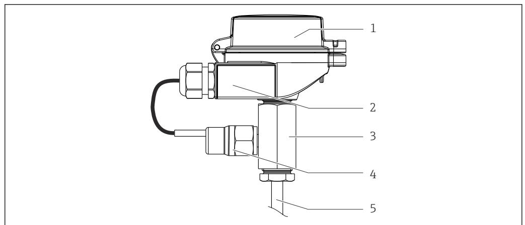
图 29 延长颈, 二次密封设计
