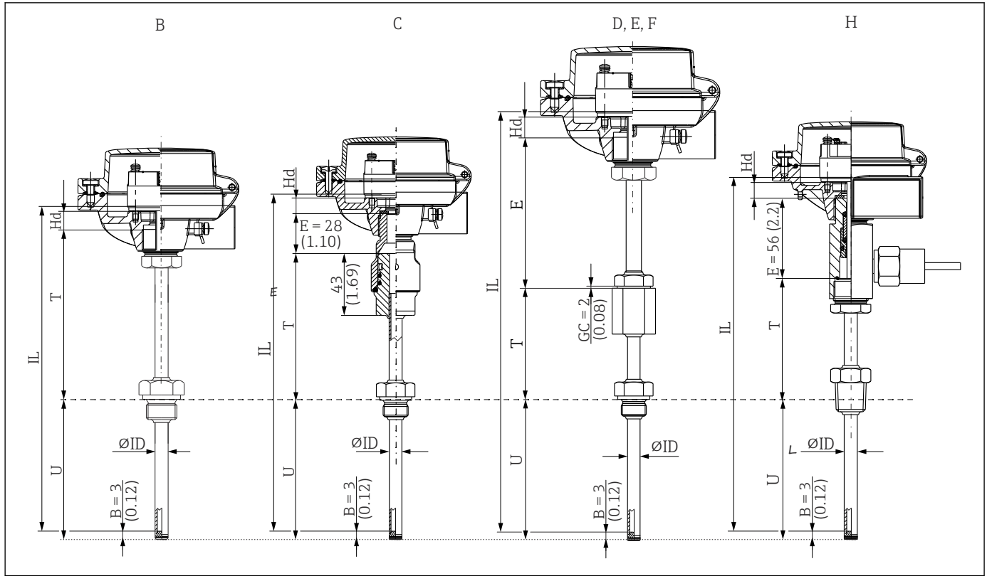
图 21 温度计配置，安装有 TS111 铠装芯子和垫圈。
