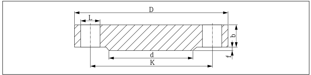
图 24 密封面形式：凸面 (B1 型)
