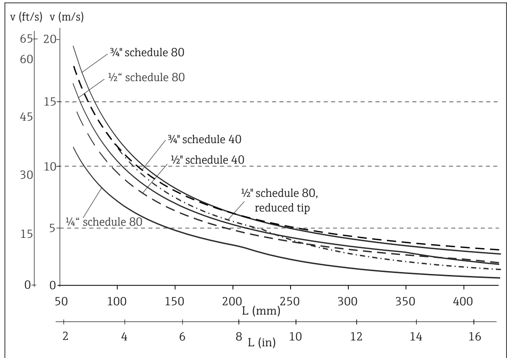
图 16 不同管径的温度计在过程介质“水”中的允许流速, T = 50 °C (122 °F)
