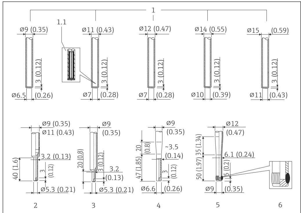
图 26 保护套管末端类型（缩径型、直管型、锥管型），最大表面光洁度 Ra \leq 0.76 \mu\text{m} (30 \mu\text{in} )，直管型保护套管的末端厚度为 3 mm (0.12 in)，定制直管型保护套管末端厚度为 4 mm (0.16 in)
