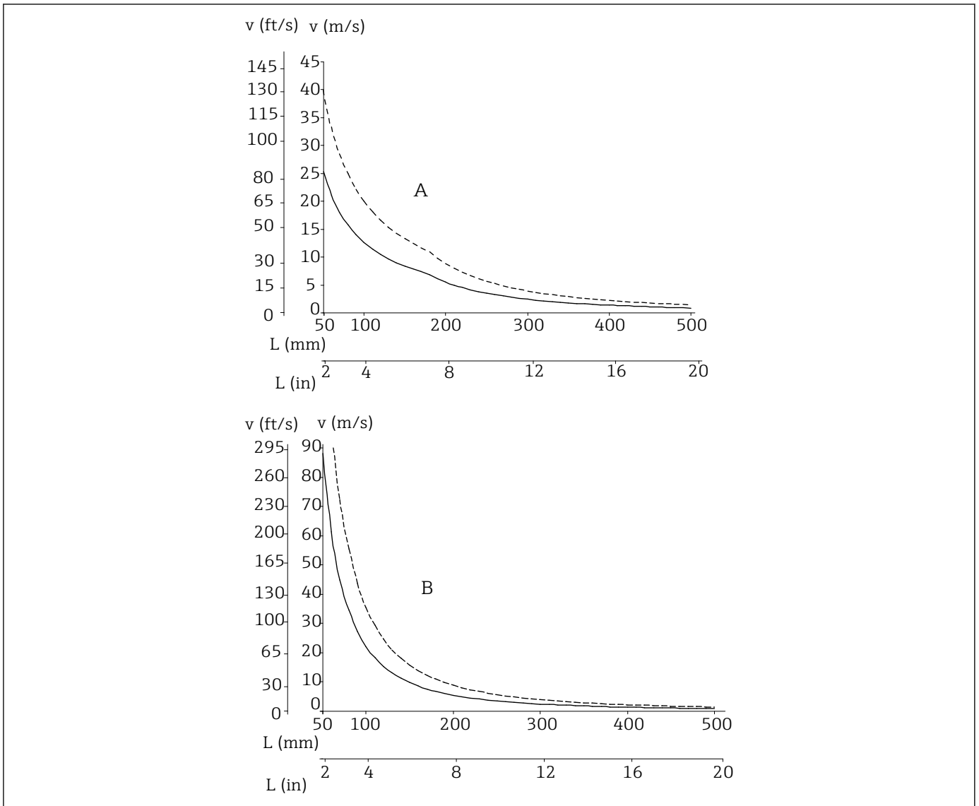
图 18 最大允许流速：9 mm (0.35 in) 保护套管 (——) 或 12 mm (0.47 in) 保护套管 (-----)
