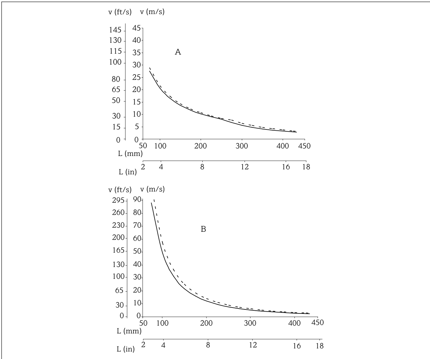
图 19 最大允许流速：14 mm (0.55 in)保护套管 (——) 或 15 mm (0.6 in)保护套管 (-----)
