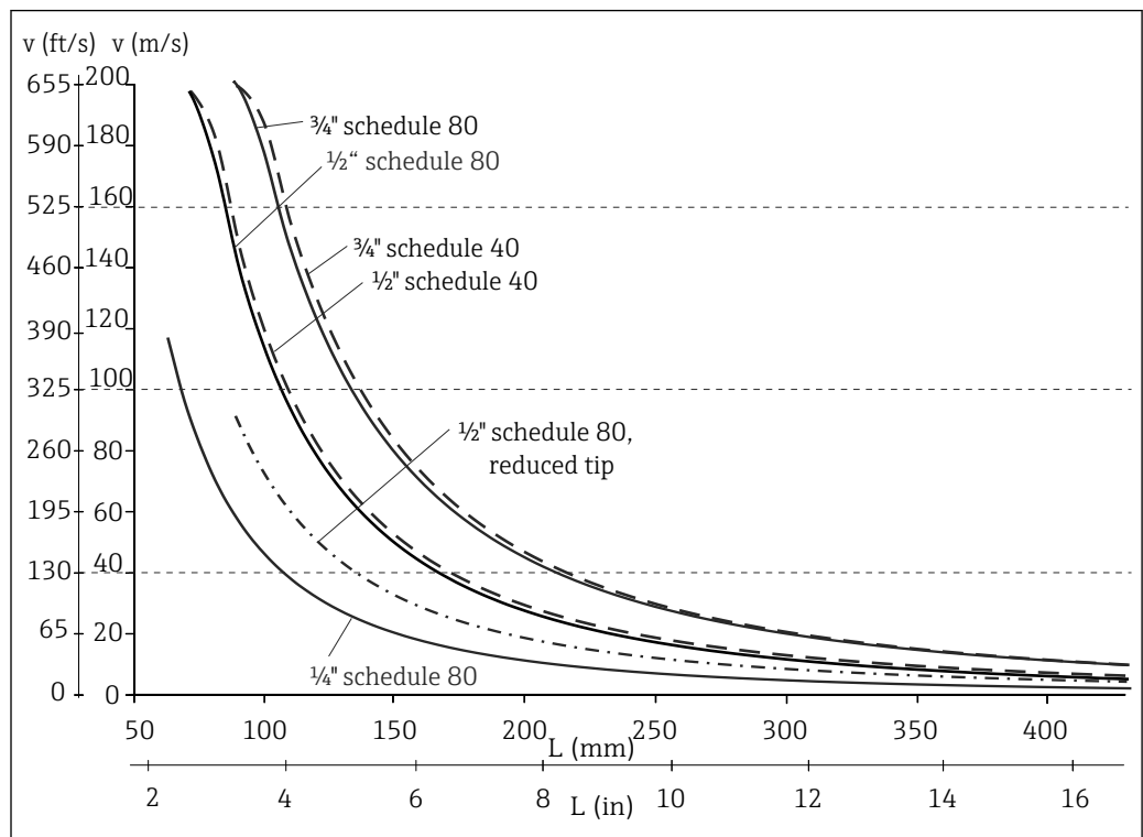
图 17 不同管径的温度计在过程介质“过热蒸汽”中的允许流速, T = 400 °C (752 °F)
