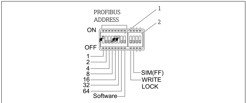
图 10 通过 DIP 开关进行硬件设置
