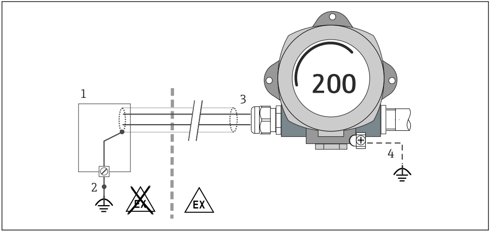
图 6 PROFIBUS®PA 通信电缆的单端屏蔽和接地连接
