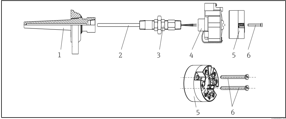
Abb. 4: Kopftransmittermontage
