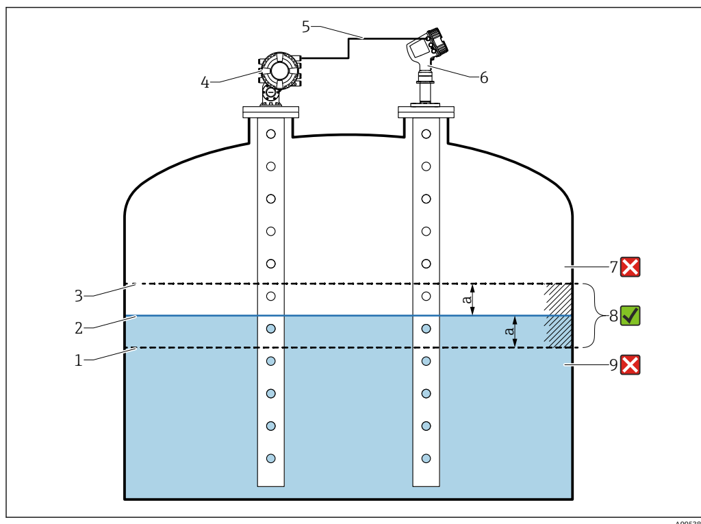
図 25 Proservo NMS8x を使用したアプリケーション事例
