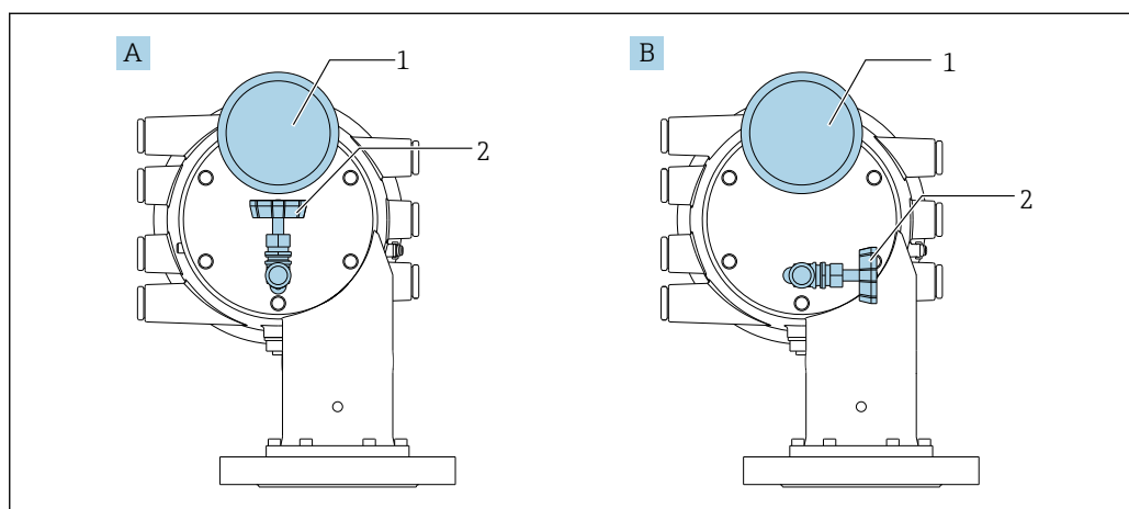
図 28 リリースバルブおよび圧力計の取付位置
