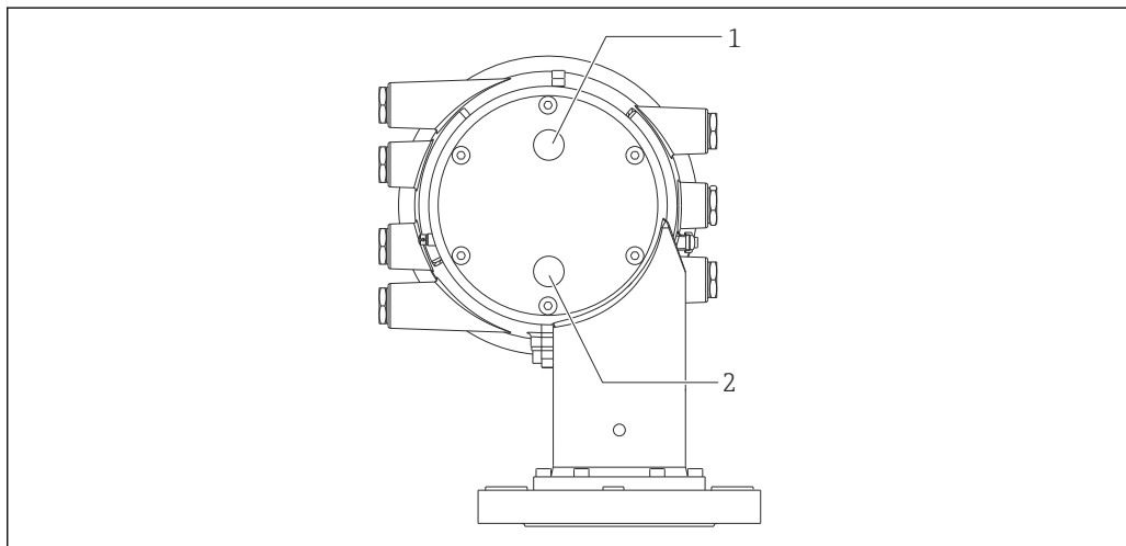
図 31 洗浄ノズルおよびガスパージノズル用の穴
