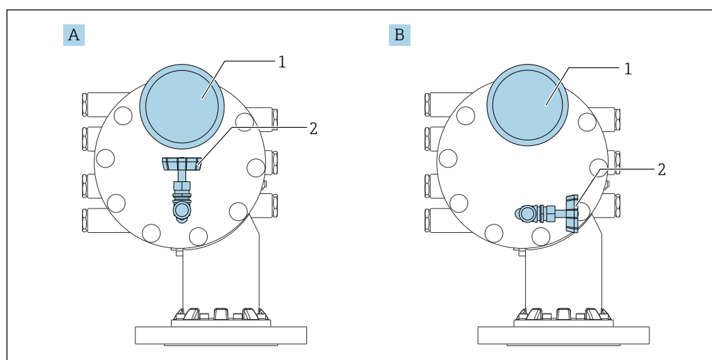
28 Position de montage de la soupape de décharge et du manomètre
