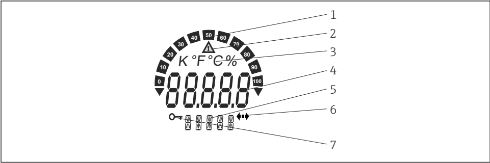
9 Afficheur LCD du transmetteur de terrain (rétroéclairé, peut être orienté par paliers de 90°)
