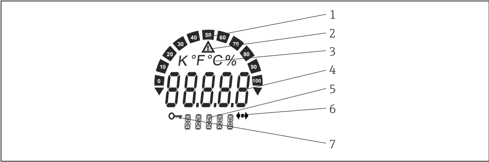
9 Indicador de cristal líquido del transmisor de campo (con iluminación de fondo, orientable en pasos de 90°)
