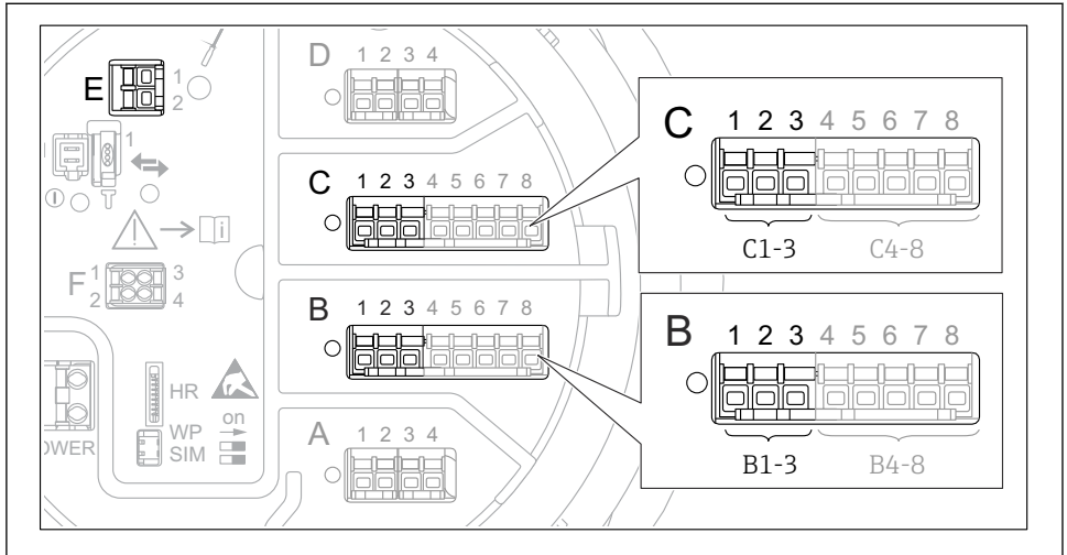
25 Possíveis terminais para malhas HART
