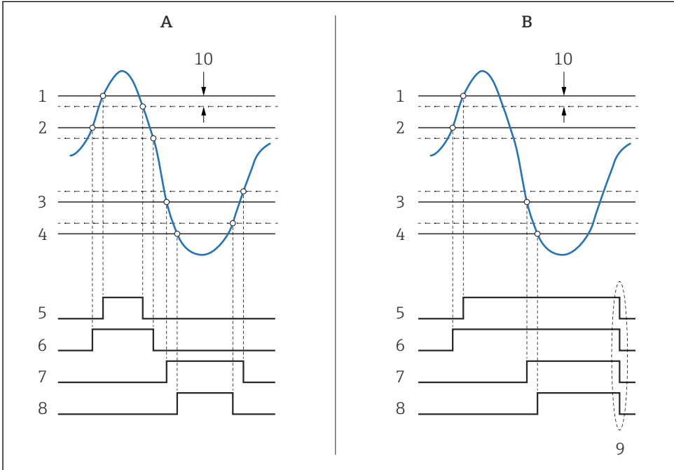
30 Princípio da avaliação de limite
