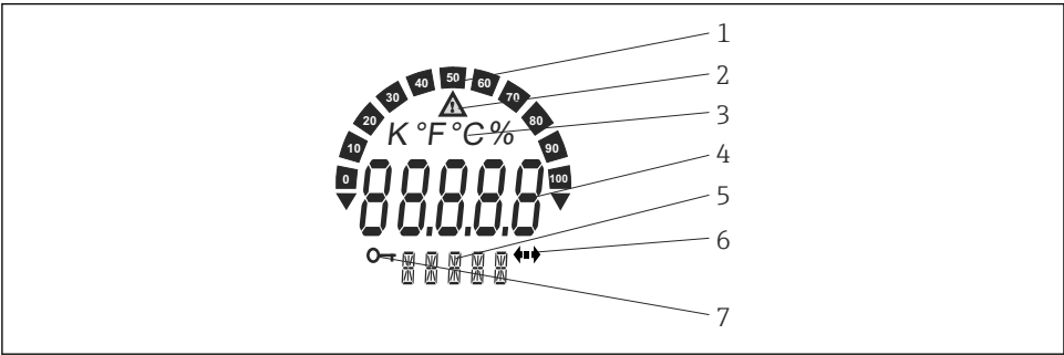
8 LC-display van de veldtransmitter (verlicht, insteekbaar in stappen van 90°)
