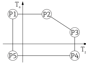
图 35 铝外壳, 带涂层; 过程温度范围: -10 \dots +150 \text{ }^{\circ}\text{C} ( +14 \dots +302 \text{ }^{\circ}\text{F} )
