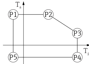
图 42 316L 外壳; 过程温度范围: -10 ... +200 °C (+14 ... +392 °F)
