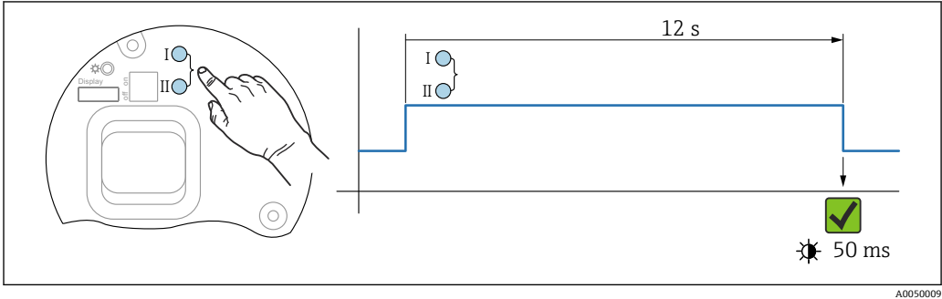
图 16 电子插件上的操作按键
