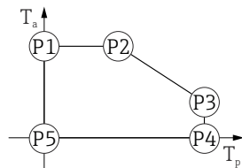
图 28 塑料外壳；过程温度范围：0 ... +150 °C (+32 ... +302 °F)，适用 CSA C/US 认证型仪表
