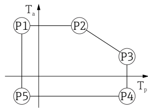
图 45 316L 外壳；过程温度范围：-40 ... +150 °C (-40 ... +302 °F)
