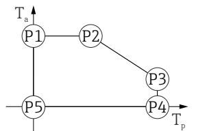
32 塑料外壳；过程温度范围：0 ... +150 °C (+32 ... +302 °F)，适用 CSA C/US 认证型仪表
