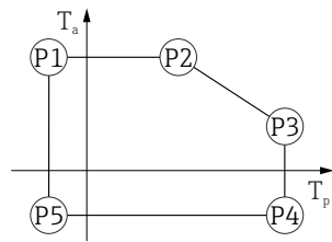
图 46 316L 外壳；过程温度范围：-40 ... +200 °C (-40 ... +392 °F)
