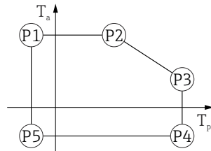
图 27 塑料外壳；过程温度范围：-20 ... +150 °C (-4 ... +302 °F)
