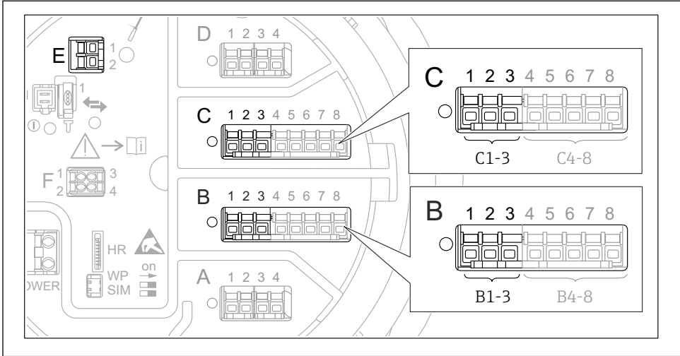
25 Possibili morsetti per loop HART
