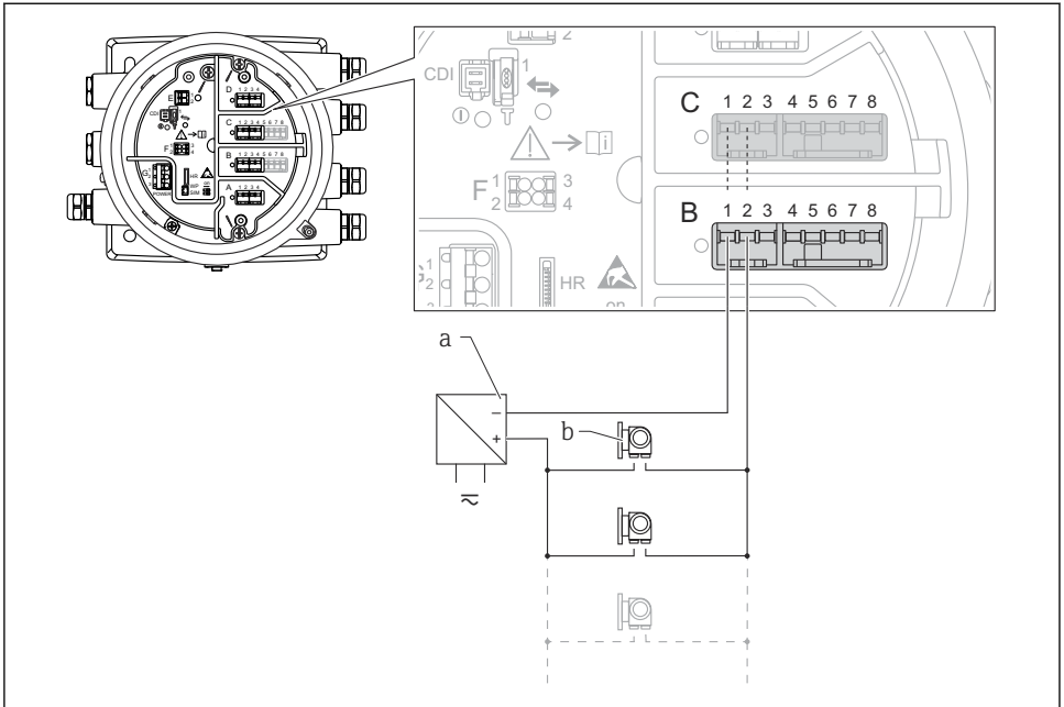
10 Useo passivo del modulo di I/O analogico in modalità master HART
