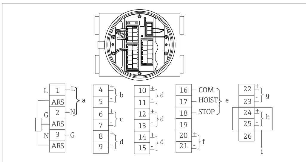
36 Bornes du NMS5
