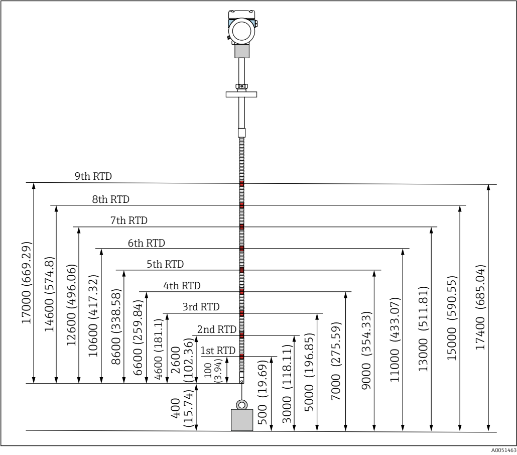
11 Position d'élément. Unité de mesure mm (in)
