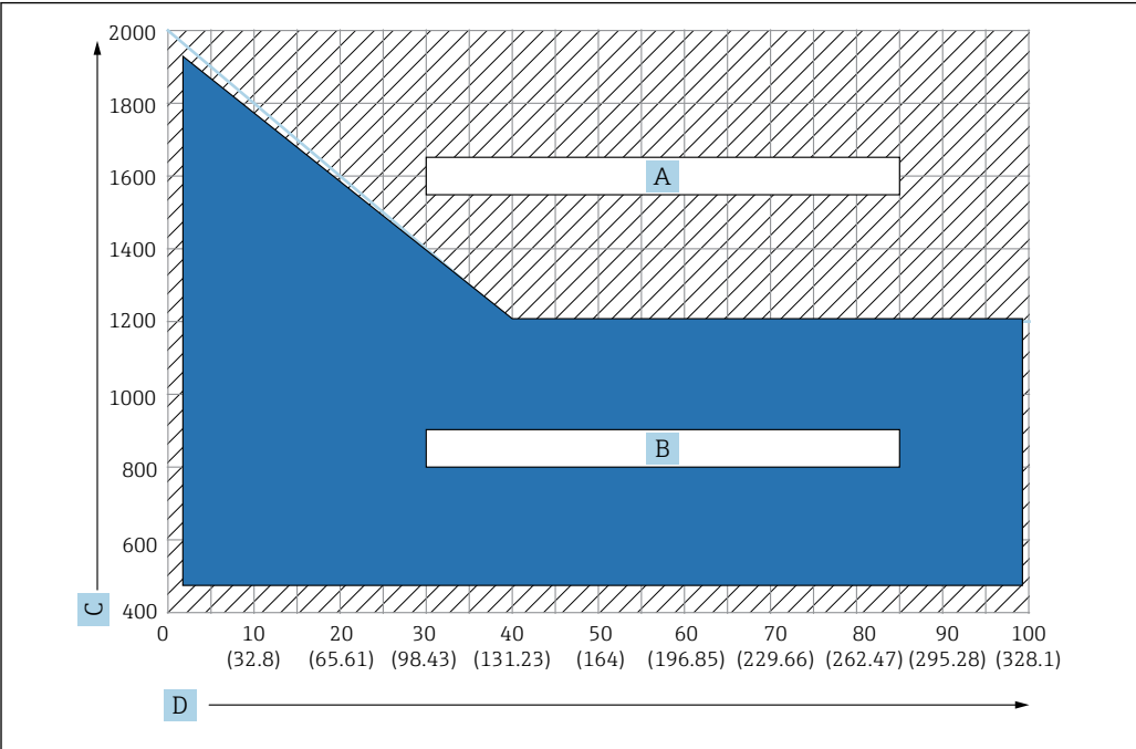
115 Tableau de sélection du poids d'ancrage, C : Unité de densité [kg/m³], D : Unité de longueur m / (ft)
