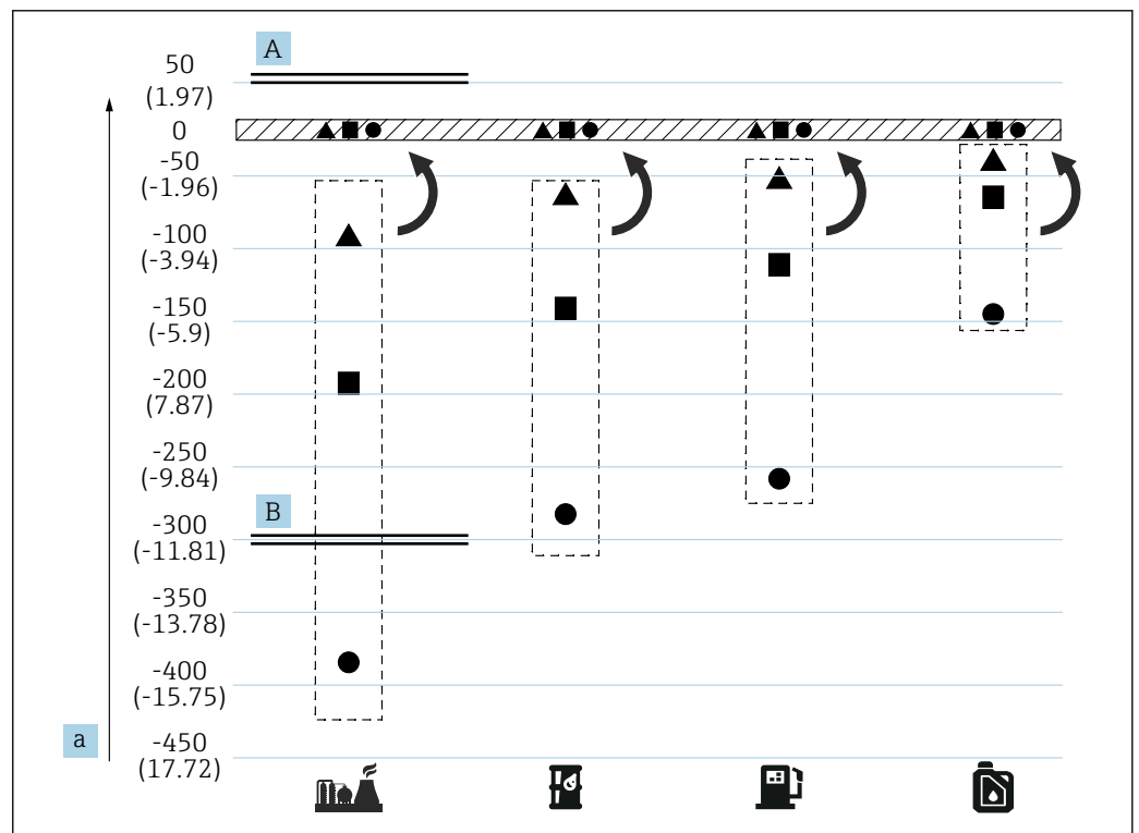
14 Effet de la compensation des trois couches
