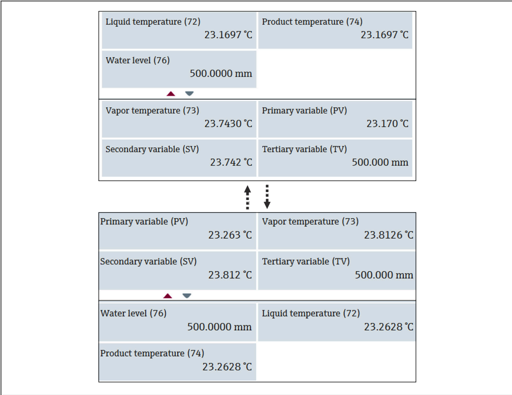
55 Zones des vues supérieure et inférieure
