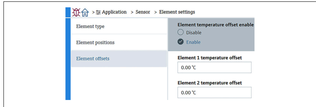
88 Écran Offsets d'élément
