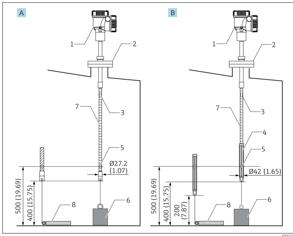
26 Méthode du poids d'ancrage. Unité de mesure mm (in)
