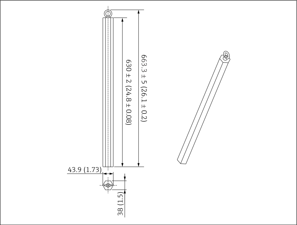
114 Accessoire de montage. Unité de mesure mm (in)
