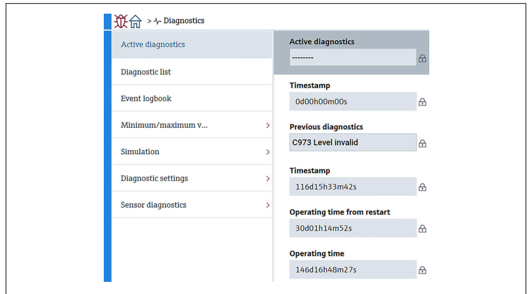
103 Écran Diagnostic actif
