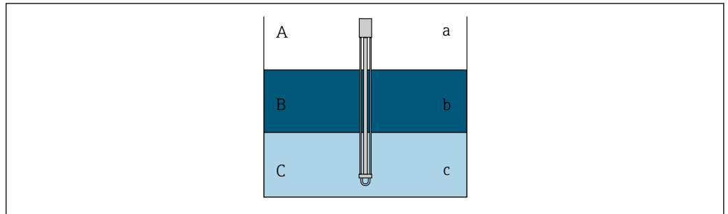
13 Mesure du niveau d'eau dans trois couches
