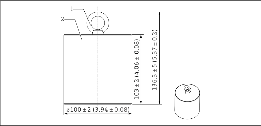
113 Accessoire de montage. Unité de mesure mm (in)
