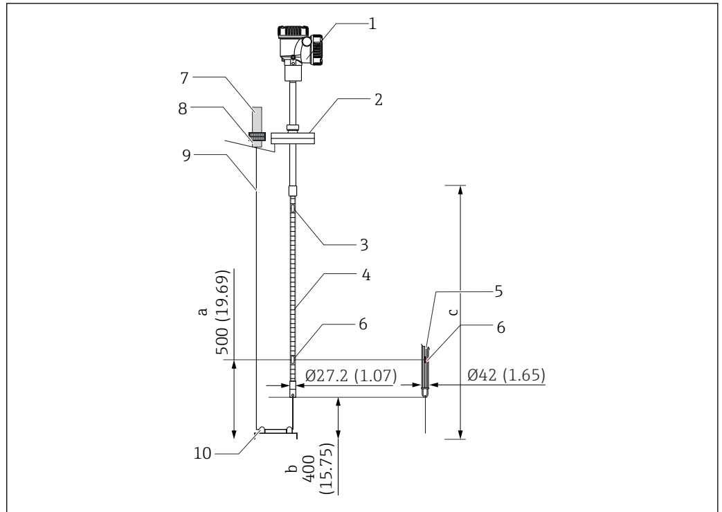
■ 22 Méthode de l'ancrage supérieur. Unité de mesure mm (in)
