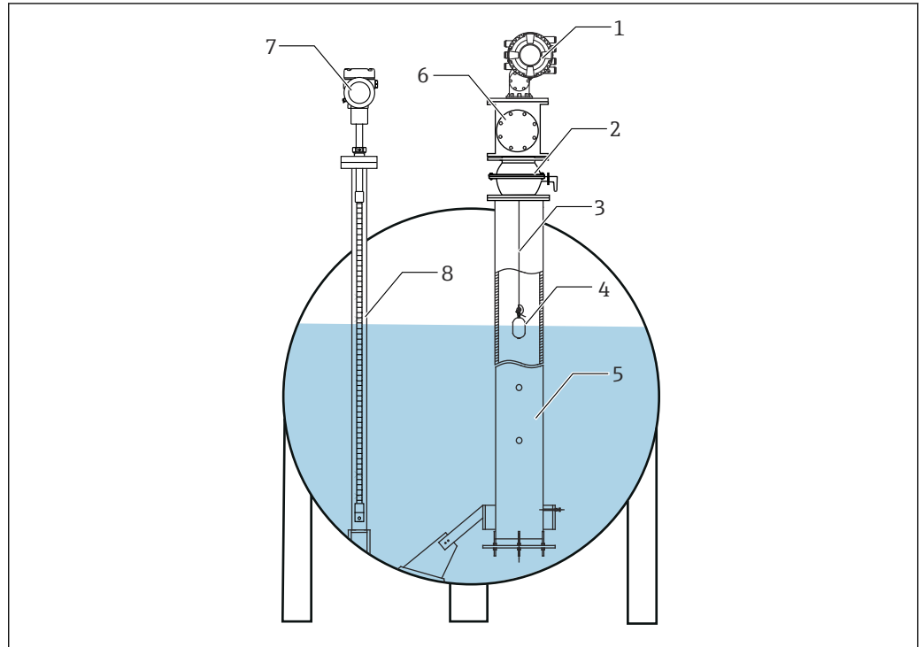
31 Protecteur pour une cuve sous pression
