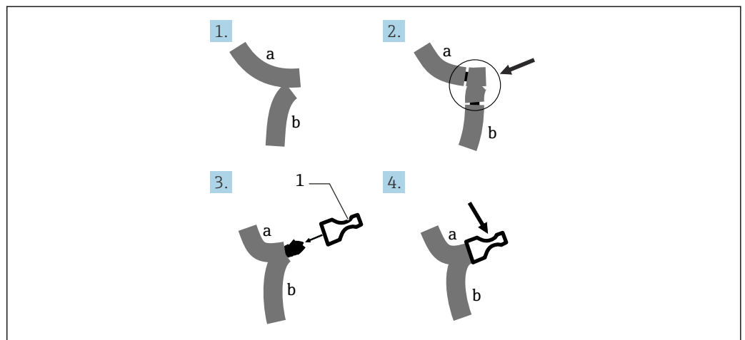
42 Raccordement des fils
