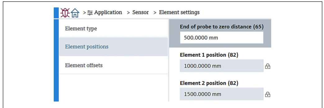
86 Écran Positions d'élément
