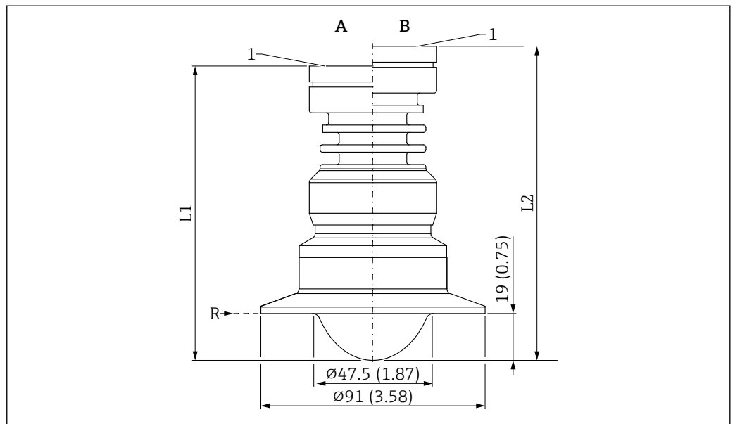
49 PTFE 外装付フラッシュマウントアンテナ (50 mm (2 in)、トリクランプ DN70-76.1 (3") ISO2852 付き) の寸法。測定単位 mm (in)
