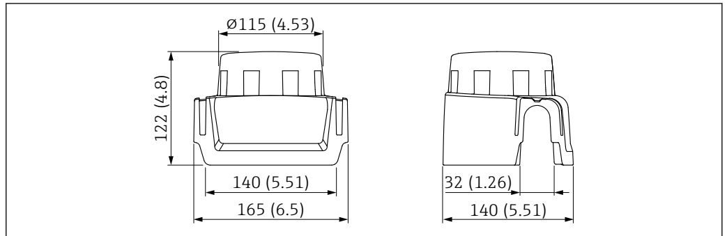
図 59 寸法。測定単位 mm (in)
