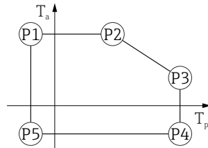
図 29 SUS 316L 相当製ハウジング ; プロセス温度 -10~+200 °C (+14~+392 °F)
