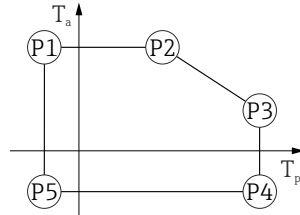
図 10 プラスチックハウジング ; プロセス温度 -10\sim+150\text{ }^{\circ}\text{C} ( +14\sim+302\text{ }^{\circ}\text{F} )
