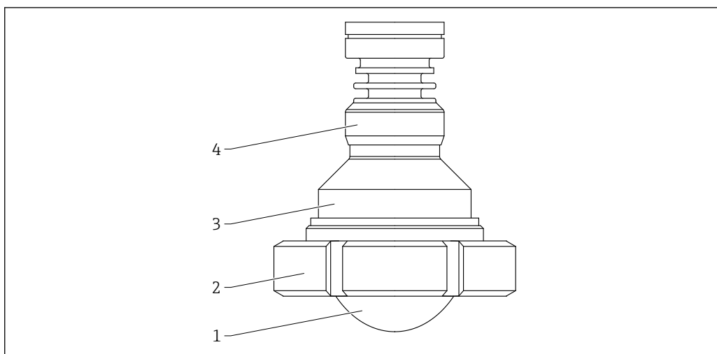
☐ 53 材質；外装付フラッシュマウントアンテナ、80 mm (3 in)、溝付ナット DIN11851。測定単位 mm (in)
