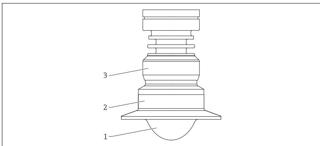
☐ 54 材質；PTFE 外装付フラッシュマウントアンテナ、50 mm (2 in)、トリクランプ ISO2852 付き。測定単位 mm (in)
