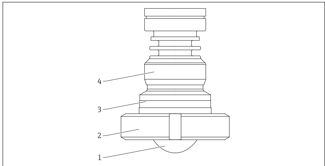
図 52 材質；外装付フラッシュマウントアンテナ、50 mm (2 in)、溝付ナット DIN11851
