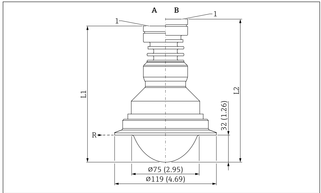
50 Dimensioni dell'antenna, flush mounted rivestita, PTFE, 80 mm (3 in), con Tri-Clamp DN101.6 (4") ISO2852. Unità di misura mm (in)
