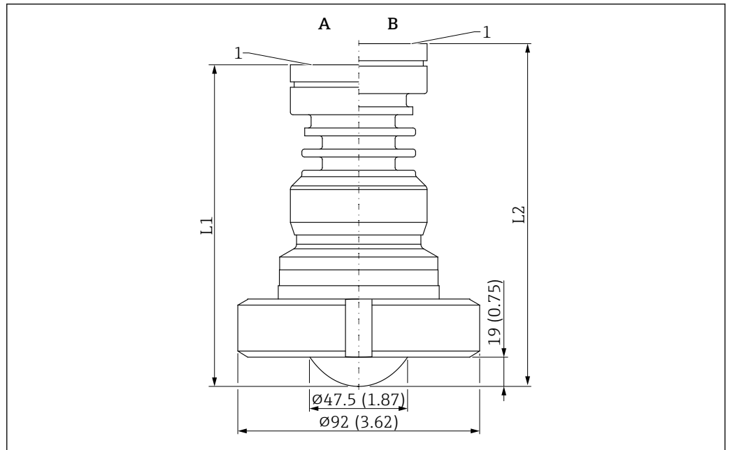
46 Dimensioni dell'antenna, flush mounted rivestita, PTFE, 50 mm (2 in), attacco a girella DIN11851. Unità di misura mm (in)
