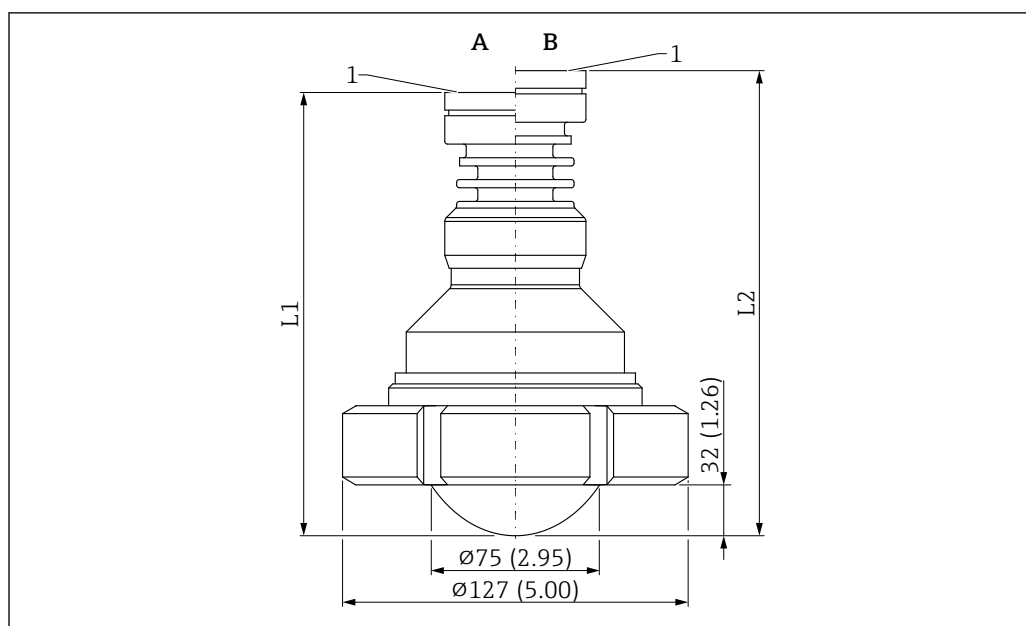
47 Dimensioni dell'antenna, flush mounted rivestita, PTFE, 80 mm (3 in), attacco a girella DIN11851. Unità di misura mm (in)
