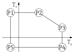
▣ 22 Custodia in alluminio; rivestita; temperatura di processo -10 \dots +150 \text{ }^{\circ}\text{C} ( +14 \dots +302 \text{ }^{\circ}\text{F} )
