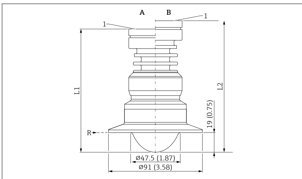
49 Dimensioni dell'antenna, flush mounted rivestita, PTFE, 50 mm (2 in), con Tri-Clamp DN70-76.1 (3") ISO2852. Unità di misura mm (in)
