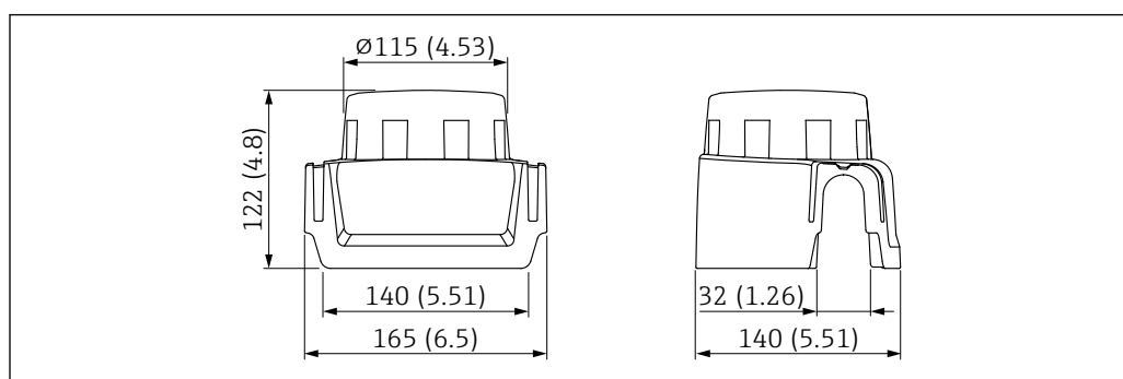
59 Dimensioni. Unità di misura mm (in)
