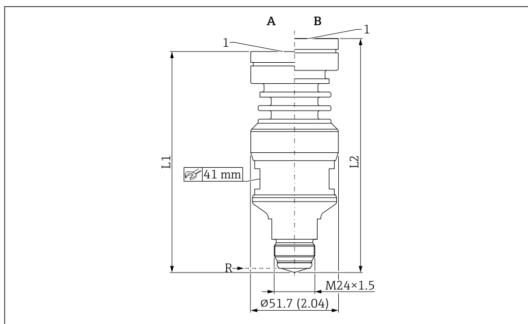
45 Dimensioni dell'antenna integrata, PEEK, 20 mm / M24×1,5. Unità di misura mm (in)
