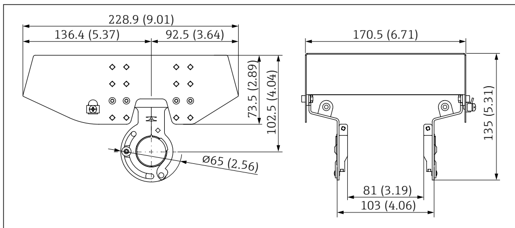
60 Размеры. Единица измерения мм (дюйм)
