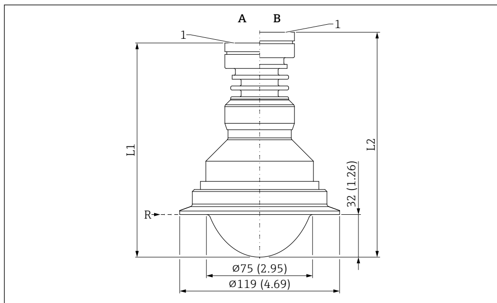
51 Размеры антенны, плакированной материалом PTFE, монтируемой заподлицо, 80 мм (3 дюйм), с соединением Tri-Clamp DN101.6 (4 дюйма) ISO 2852. Единица измерения мм (дюйм)
