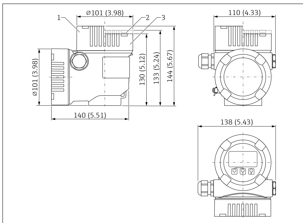
45 Размеры корпуса L-образной формы с двумя отсеками. Единица измерения мм (дюйм)
