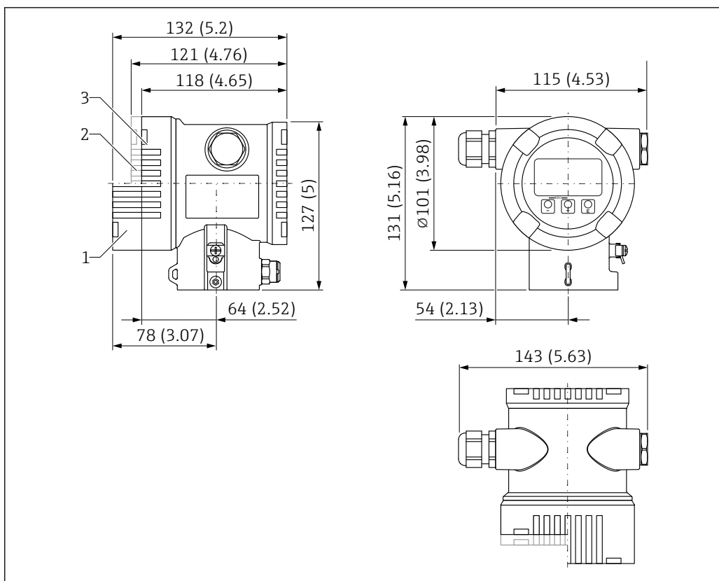
44 Размеры корпуса с двумя отсеками, алюминий. Единица измерения мм (дюйм)
