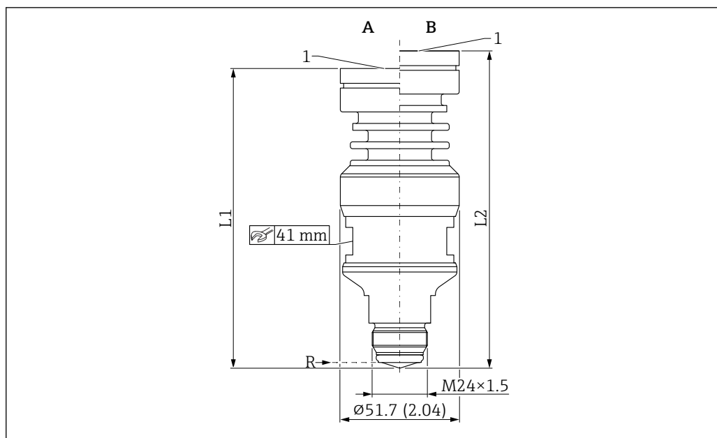
46 Размеры встроенной антенны, PEEK, 20 мм/M24 × 1,5. Единица измерения мм (дюйм)
