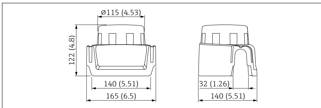
61 Размеры. Единица измерения мм (дюйм)
