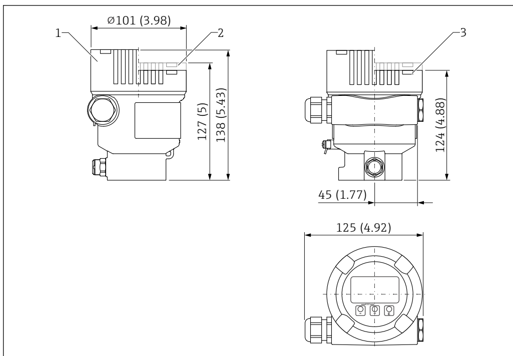
42 Размеры корпуса с одним отсеком, алюминий. Единица измерения мм (дюйм)
