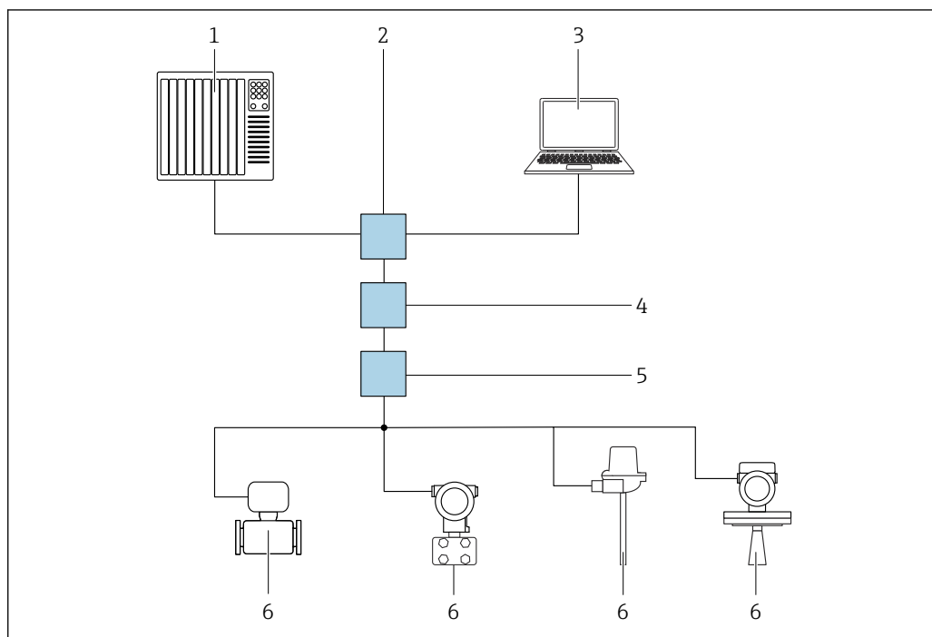
■ 59 Варианты дистанционного управления через сеть PROFINET с Ethernet-APL: топология «звезда»
