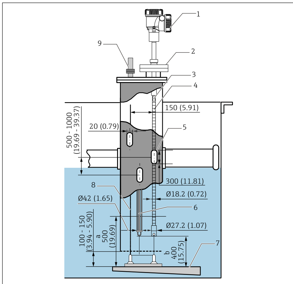
28 Metodo con ancoraggio superiore. Unità di misura mm (in)
