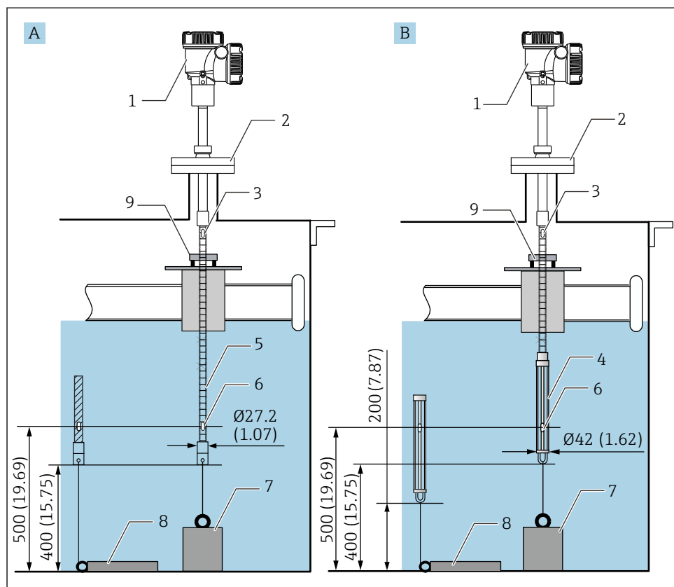
30 Metodo con anello di guida e peso di ancoraggio. Unità di misura mm (in)
