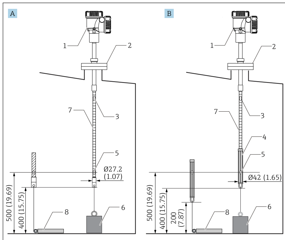
26 Metodo con peso di ancoraggio. Unità di misura mm (in)
