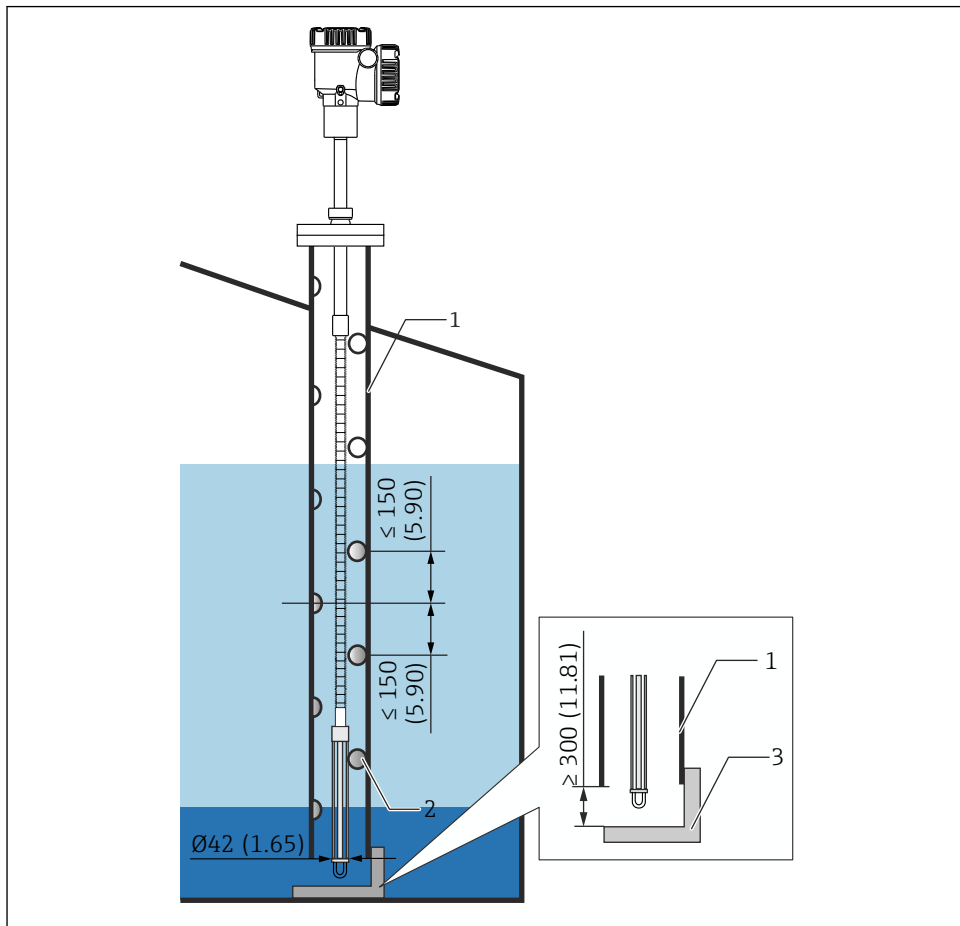
25 Tubo di calma. Unità di misura mm (in)
