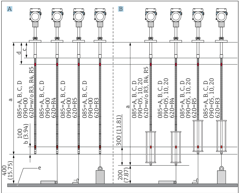
10 Posizione dell'elemento N. 1 di NMT81 in base al metodo di installazione. Unità di misura mm (in)
