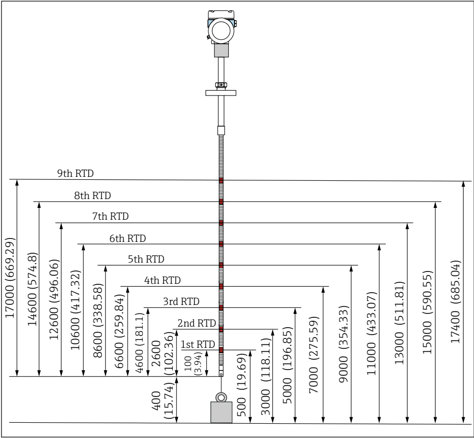
11 Posizione elemento. Unità di misura mm (in)
