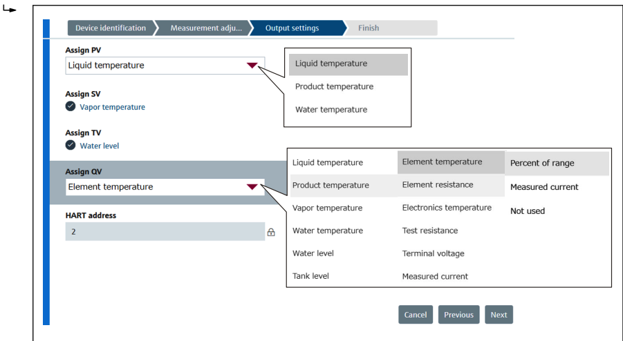
46 Schermata delle impostazioni uscita
