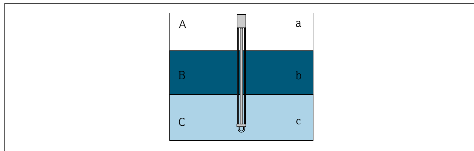
13 Misura del livello dell'acqua nelle tre fasi
