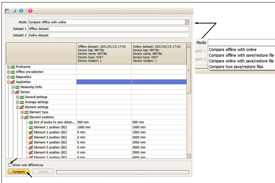
52 Экран сравнения наборов данных
