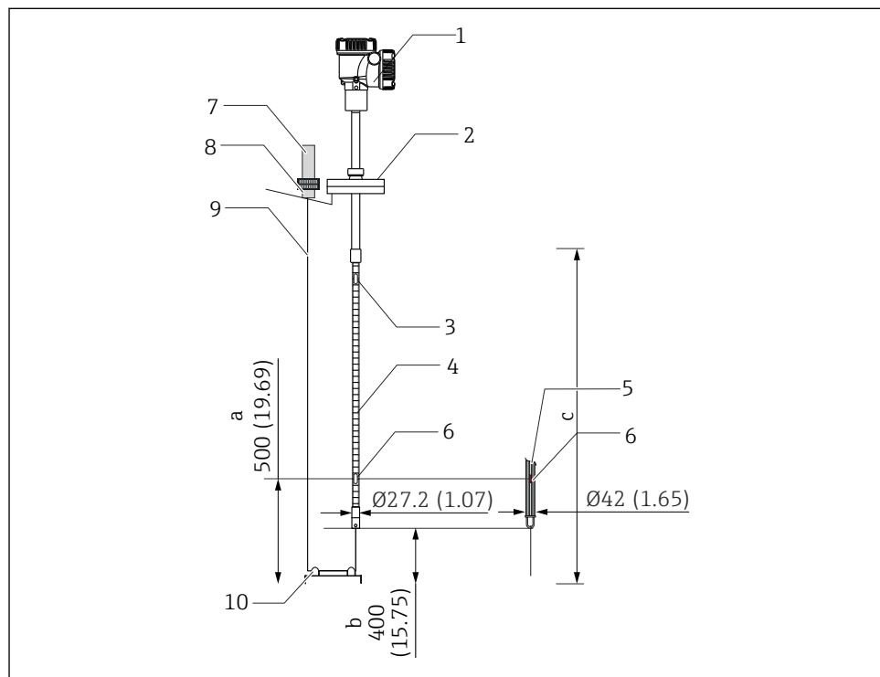
■ 22 Метод с использованием верхнего анкера. Единица измерения мм (дюйм)
