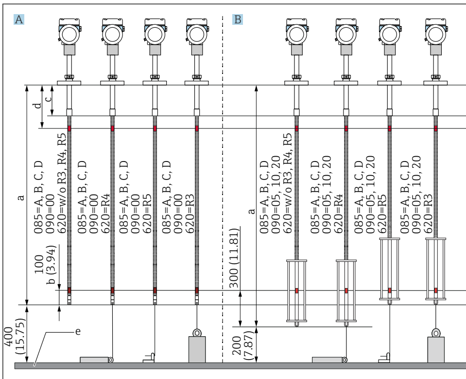
10 Положение чувствительного элемента №1 прибора NMT81 в зависимости от метода монтажа. Единица измерения мм (дюйм)
