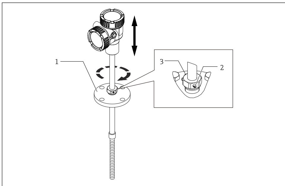
20 Прибор NMT81 с регулятором высоты
