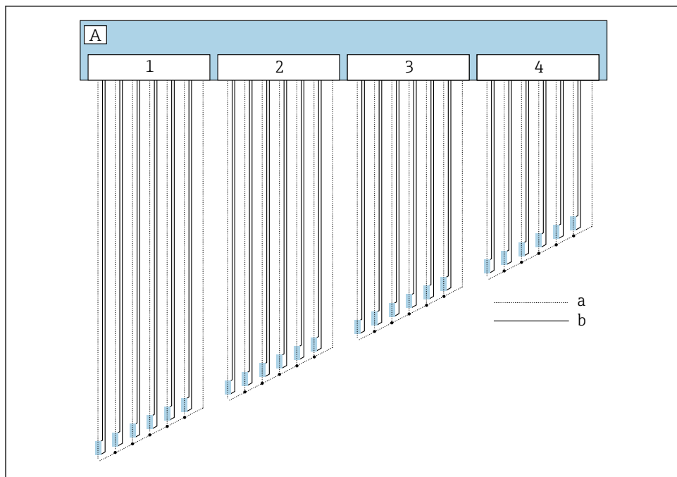
34 Схема четырехпроводного подключения
