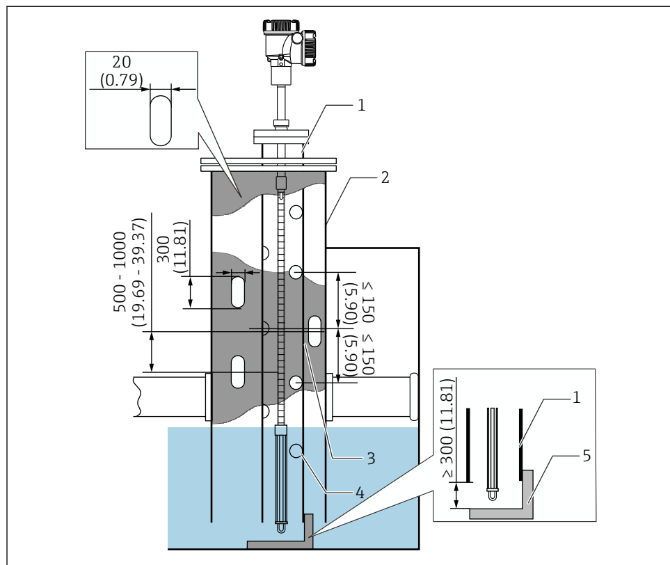
29 Метод с использованием успокоительной трубы. Единица измерения мм (дюйм)
