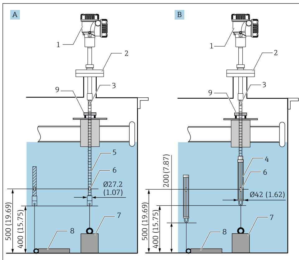
30 Метод с использованием направляющего кольца и якорного груза. Единица измерения мм (дюйм)
