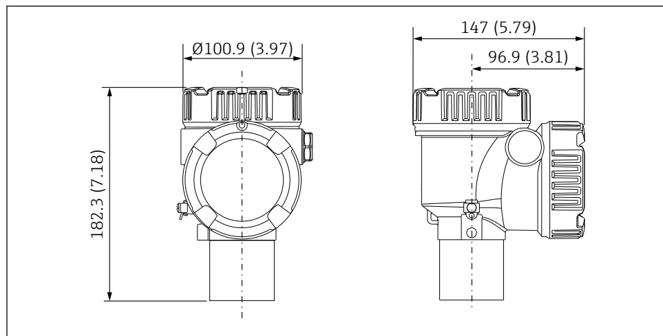
3 Стандартный преобразователь. Единица измерения мм (дюйм)
