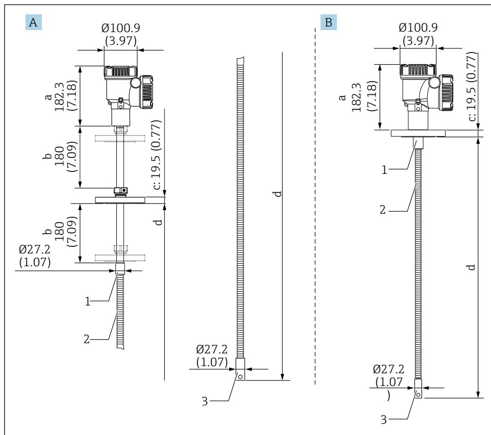
6 Преобразователь с зондом для измерения средней температуры. Единица измерения мм (дюйм)
