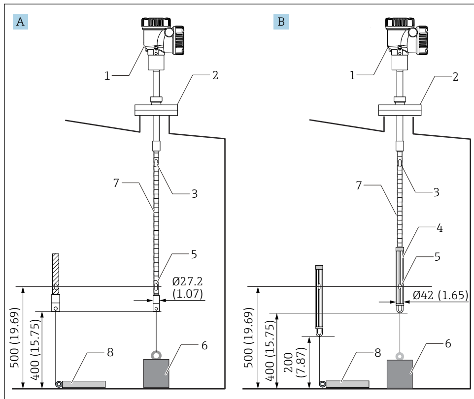
26 Метод с использованием якорного груза. Единица измерения мм (дюйм)
