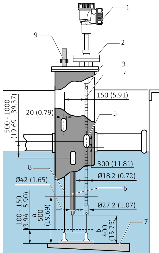
28 Метод с использованием верхнего анкера. Единица измерения мм (дюйм)
