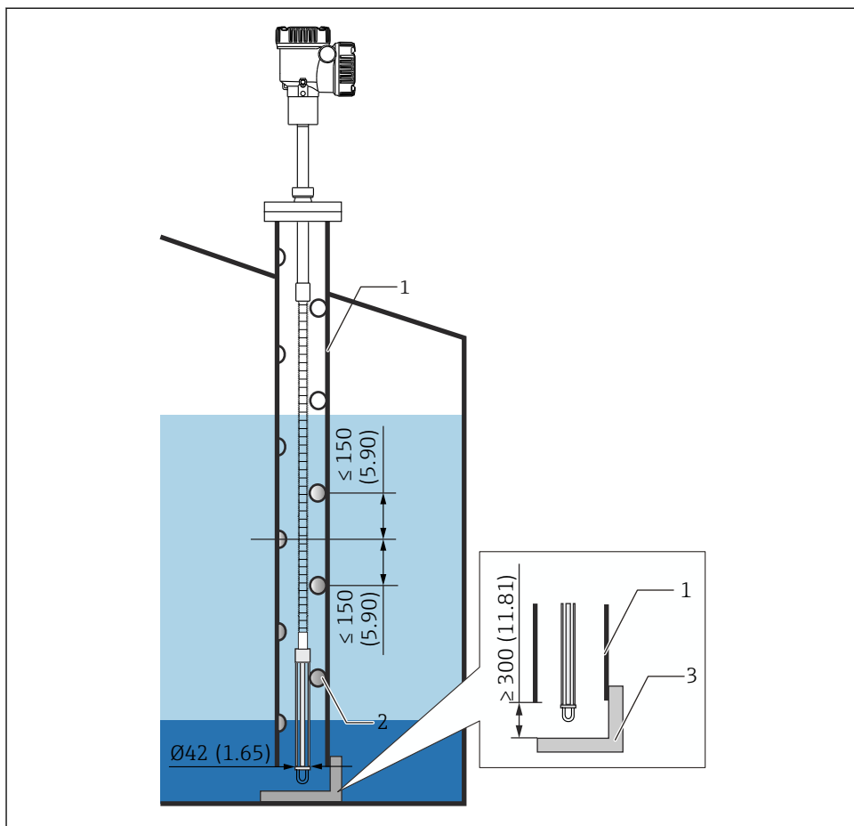
25 Успокоительная труба. Единица измерения мм (дюйм)
