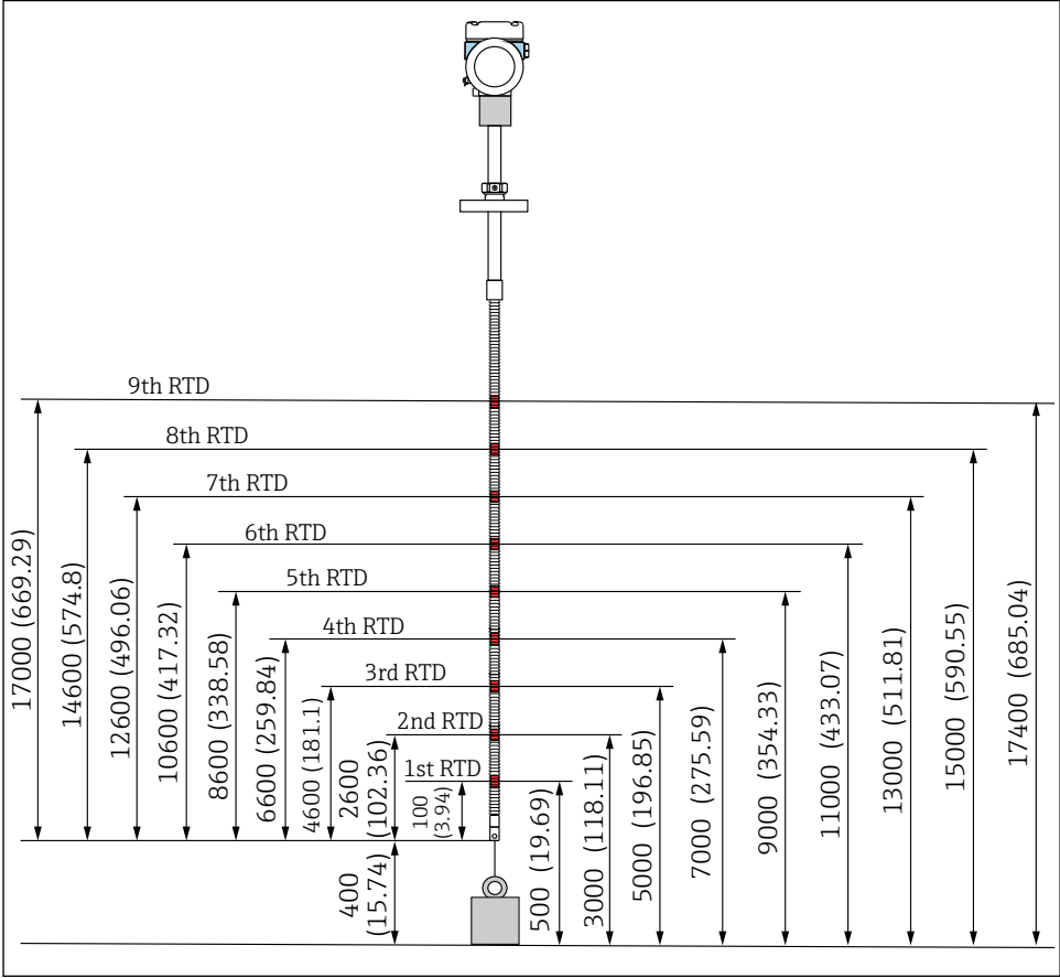
11 Положение чувствительного элемента. Единица измерения мм (дюйм)
