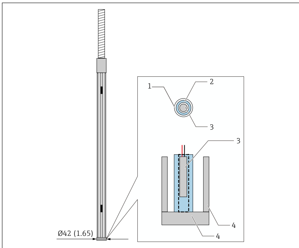
12 Конструкция зонда подтоварной воды. Единица измерения мм (дюйм)
