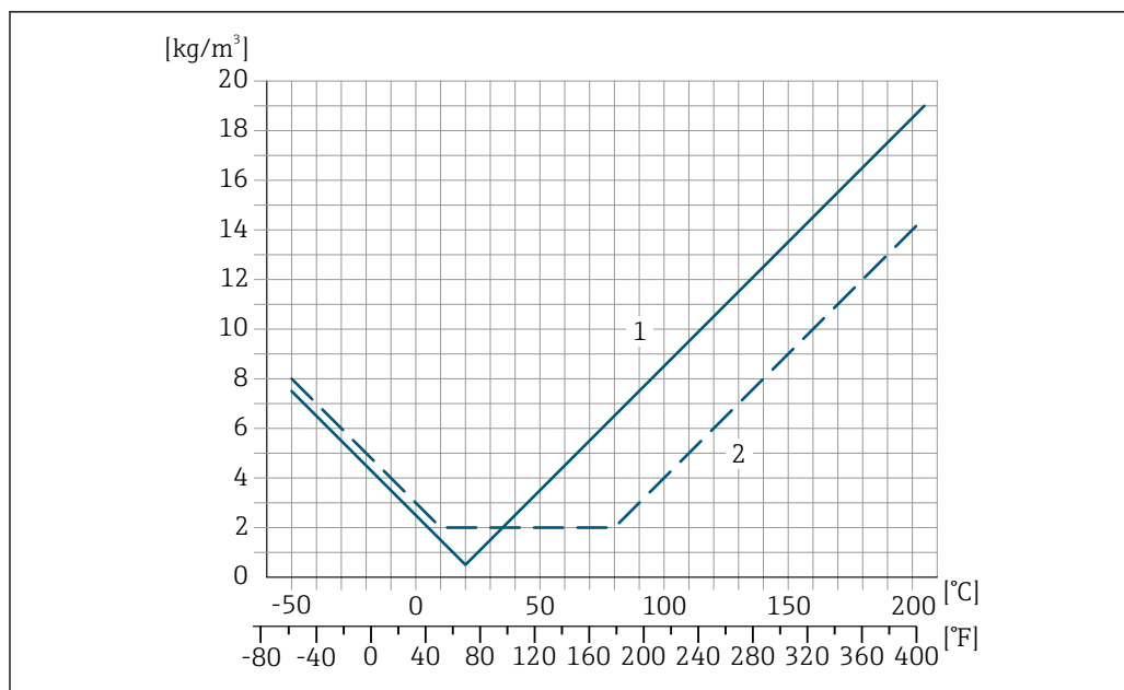
1 Калибровка по плотности на месте эксплуатации, в примере – при температуре +20 °C (+68 °F) 2 Специальная калибровка по плотности
