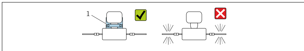
1 Держатель датчика (код заказа «Прилагаемые аксессуары», опция PR)
