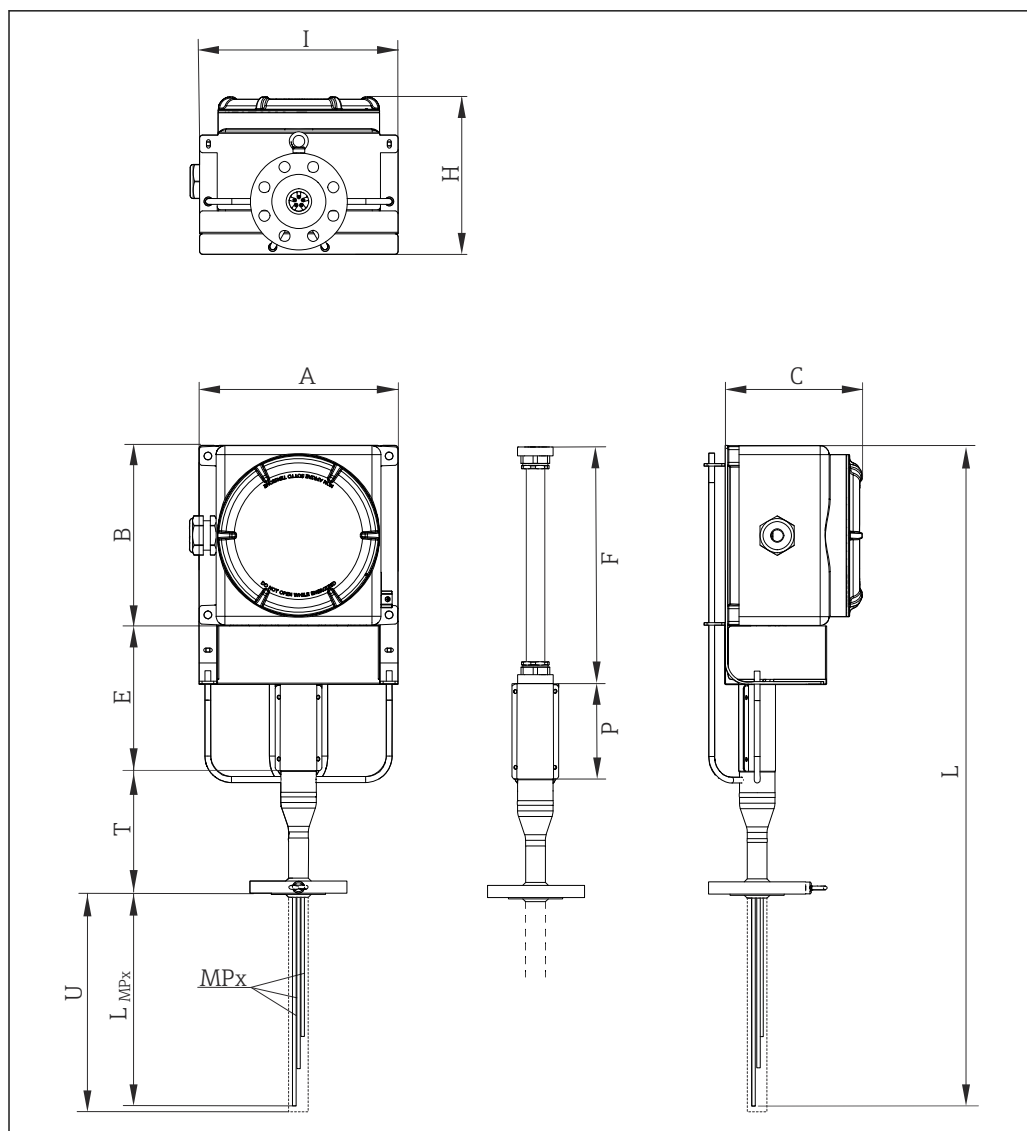
9 Diseño del termómetro multipunto modular, con bastidor de soporte. Todas las medidas están expresadas en mm (in)
