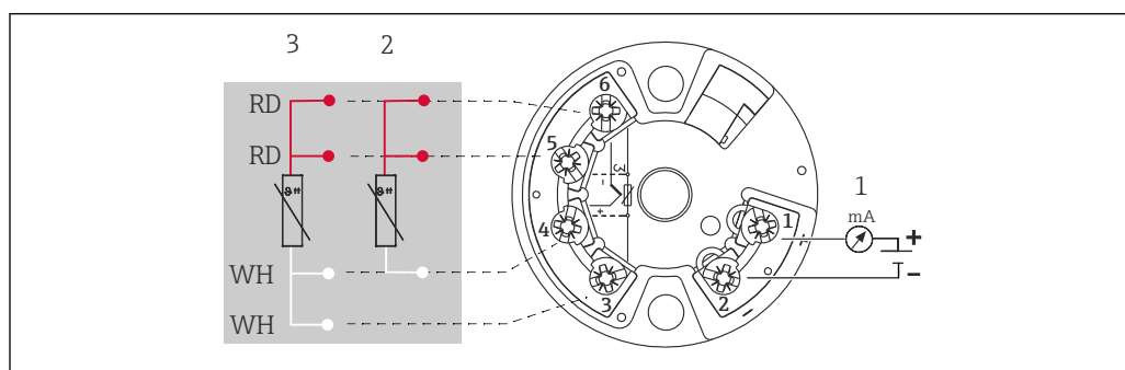
3 Transmisor montado en cabezal TMT18x (entrada de sensor simple)
