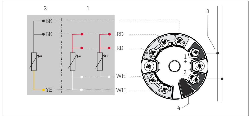
5 Transmisor montado en cabezal TMT8x (entrada de sensor doble)
