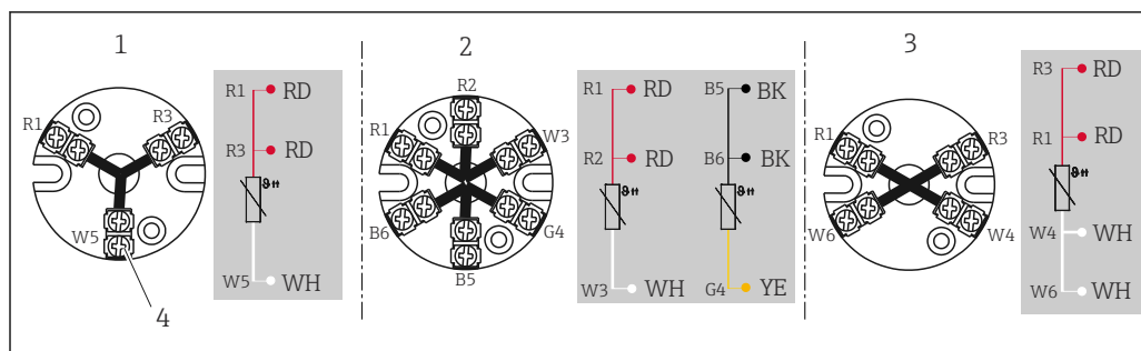
2 Regleta de terminales montada
