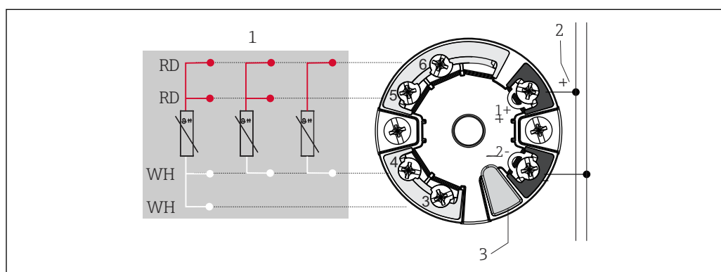
4 Transmisor TMT7x o TM31 (de una entrada) montado en cabezal
