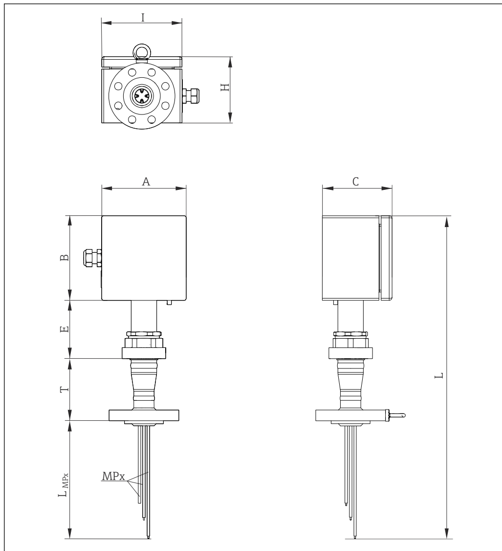
10 Diseño de la sonda de temperatura multipunto modular, con cuello para soporte tubular. Todas las medidas están expresadas en mm (in)
