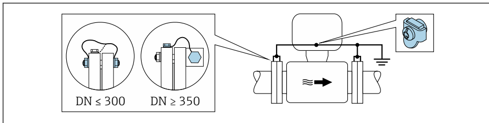
5 Potentialutjämning via jordanslutning och rörfänsar
