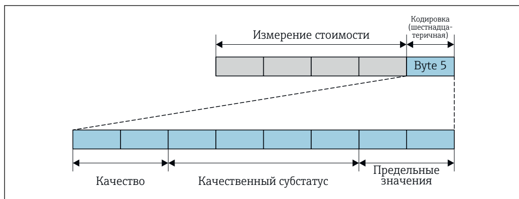
32 Структура байта состояния
