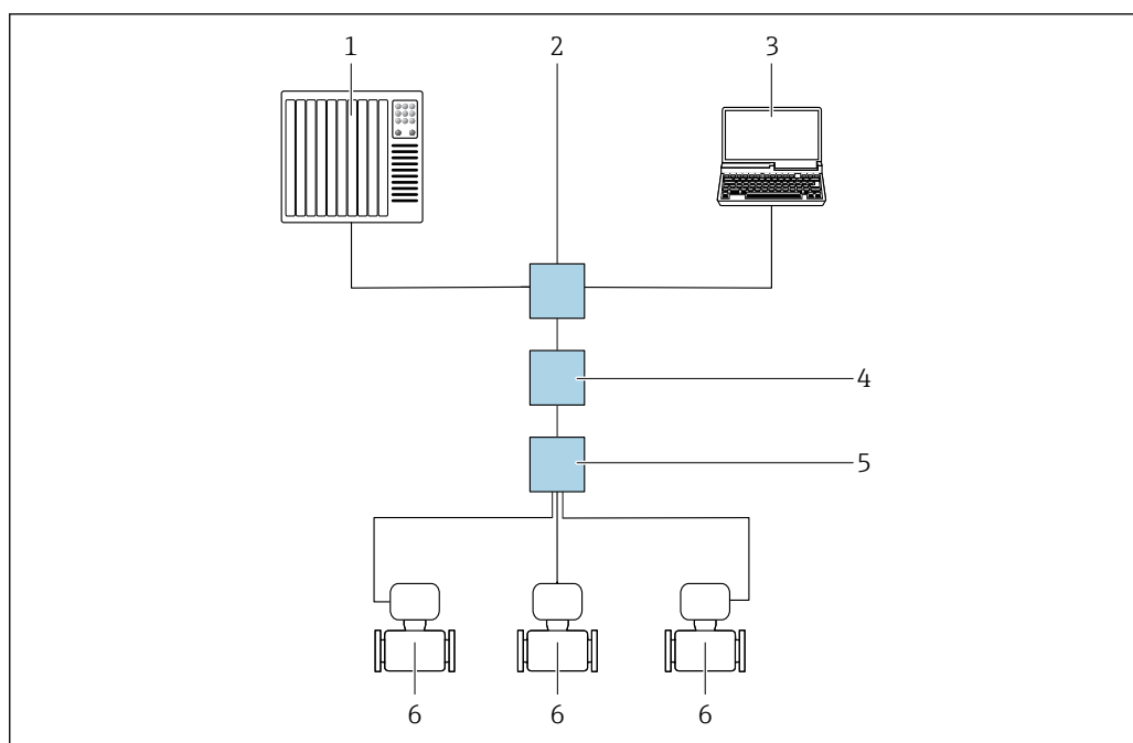
25 Варианты дистанционного управления через сеть APL
