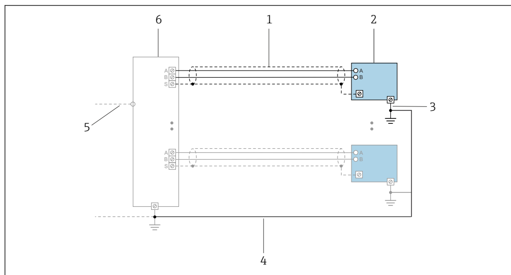
13 Пример подключения для интерфейса PROFINET с Ethernet-APL
