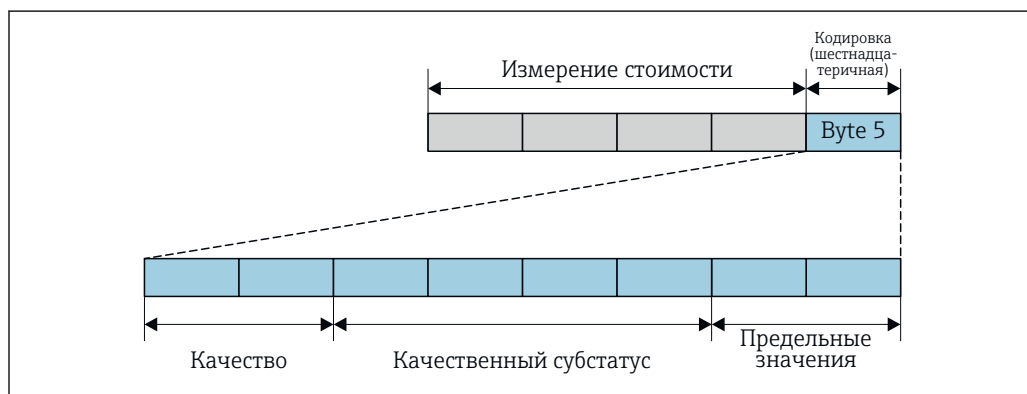
41 Структура байта состояния
