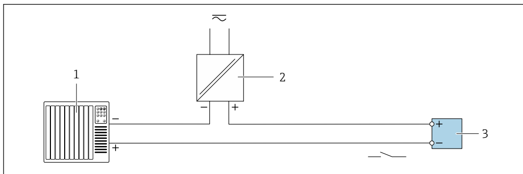
25 Пример подключения для релейного выхода (пассивного)
