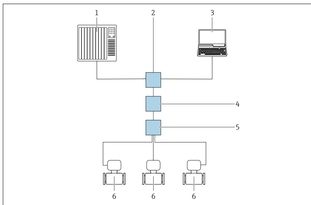
33 Варианты дистанционного управления через сеть APL
