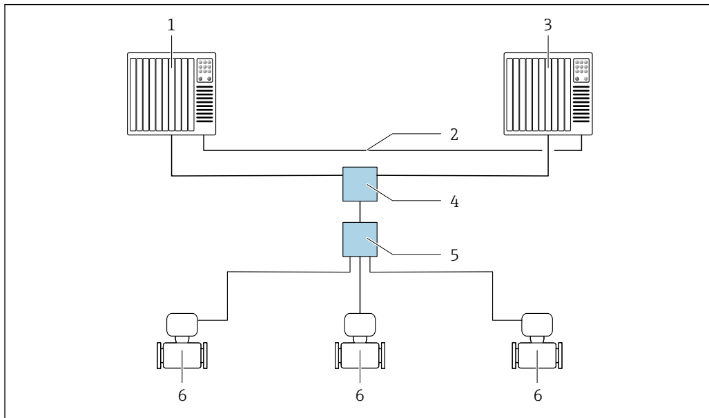
36 Пример компоновки резервируемой системы (S2): топология "звезда"
