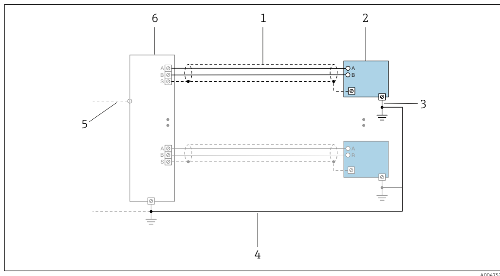
18 Пример подключения для PROFINET с Ethernet-APL
