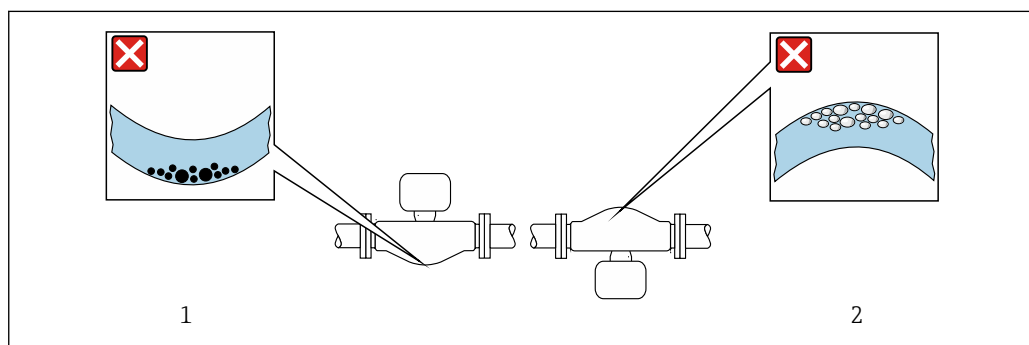
7 Ориентация датчика с изогнутой измерительной трубкой
