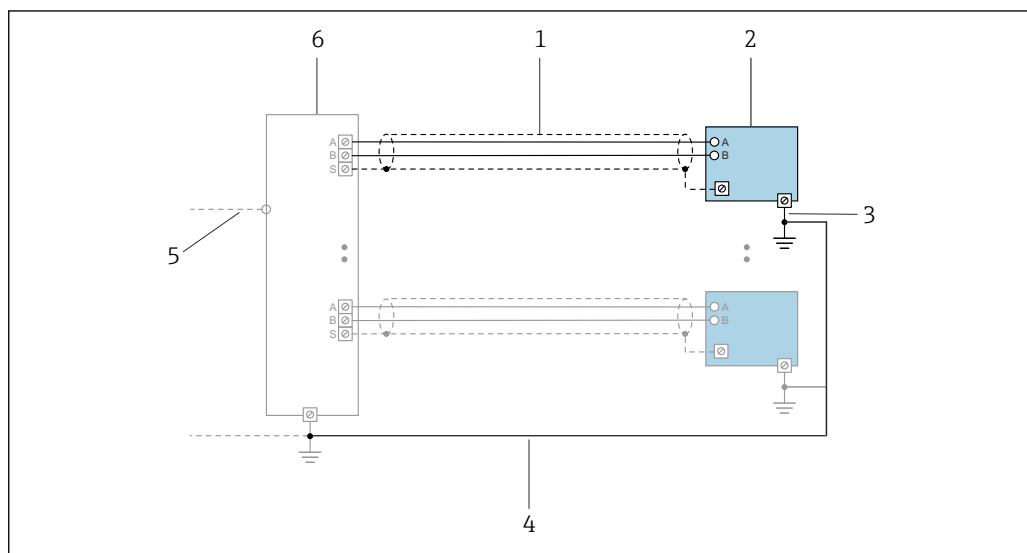
10 Пример подключения для интерфейса PROFINET с Ethernet-APL
