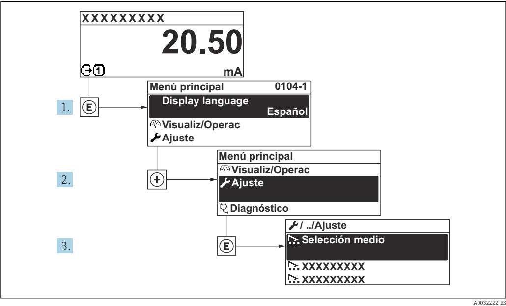
37 Navegación a Menú "Ajuste" utilizando el ejemplo del indicador local
