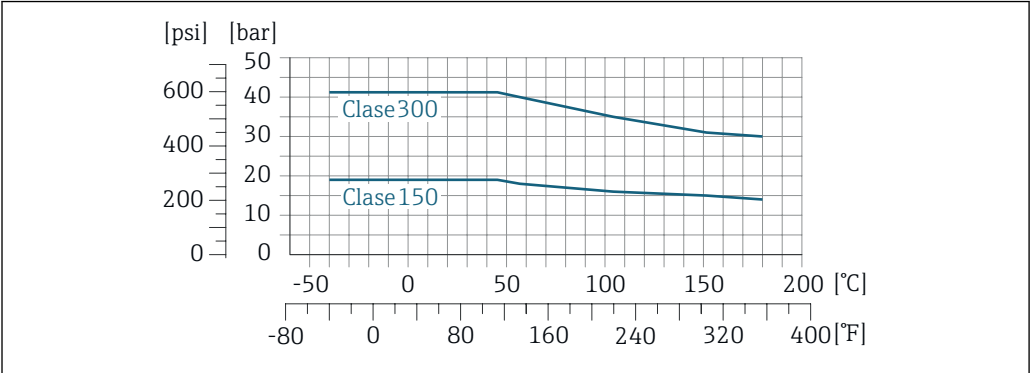
45 Con material 1.4404/F316L/F316 para la brida
