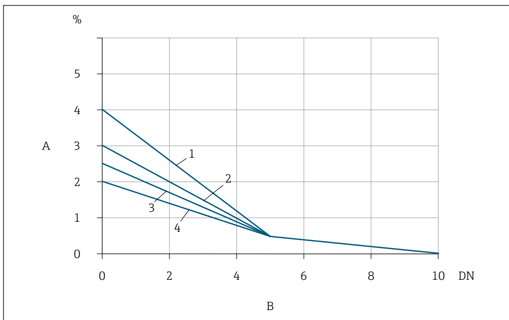
12 Error medido adicional que cabe esperar con acondicionadores de flujo en función del tipo de perturbación y del tramo recto de entrada
