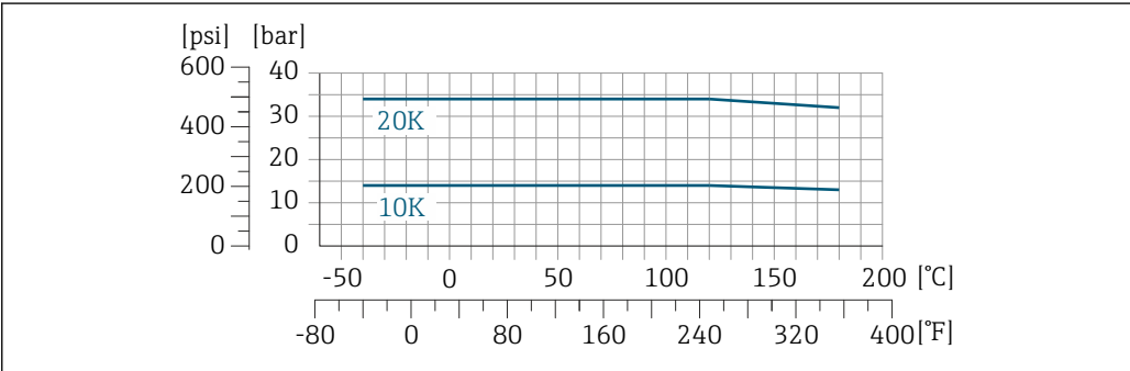
44 Con material 1.4404/F316L/F316 para la brida
