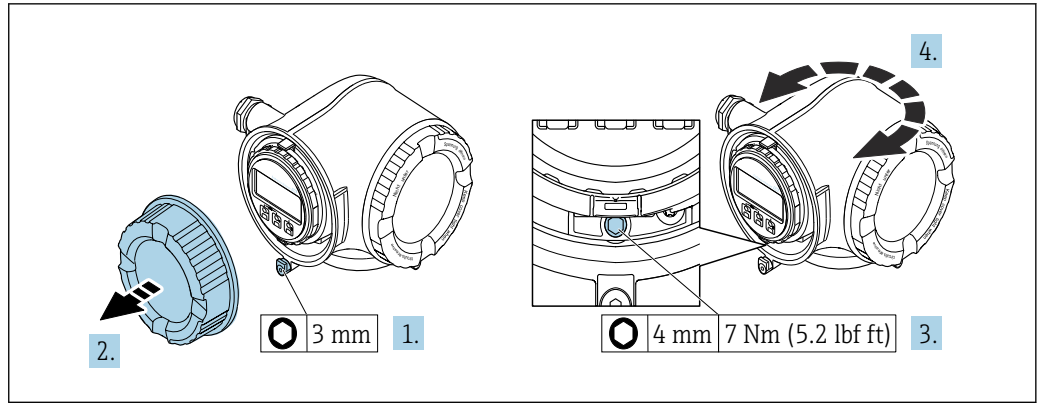
图 16 非防爆型外壳
