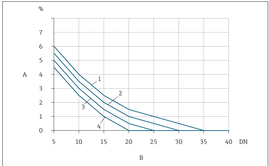
21 L'écart de mesure supplémentaire auquel il faut s'attendre en l'absence de tranquillisateurs de débit dépend du type de perturbation et de la longueur droite d'entrée
