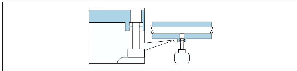
27 Isolation thermique avec tube prolongateur non isolé
