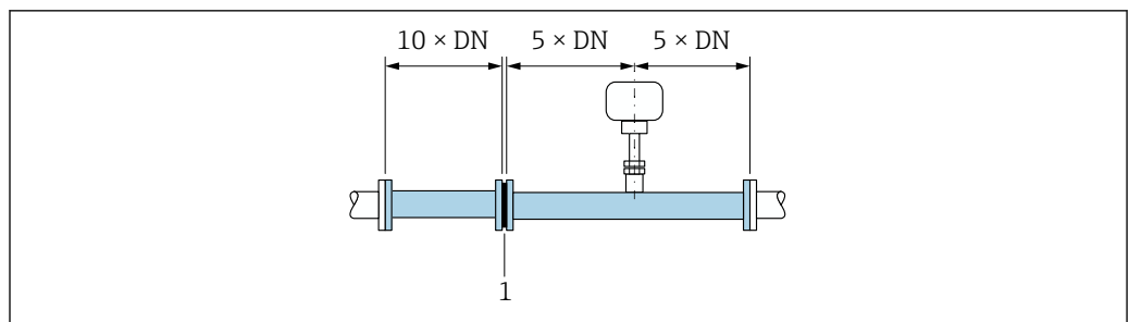
11 使用流量调节器时的推荐前后直管段长度
