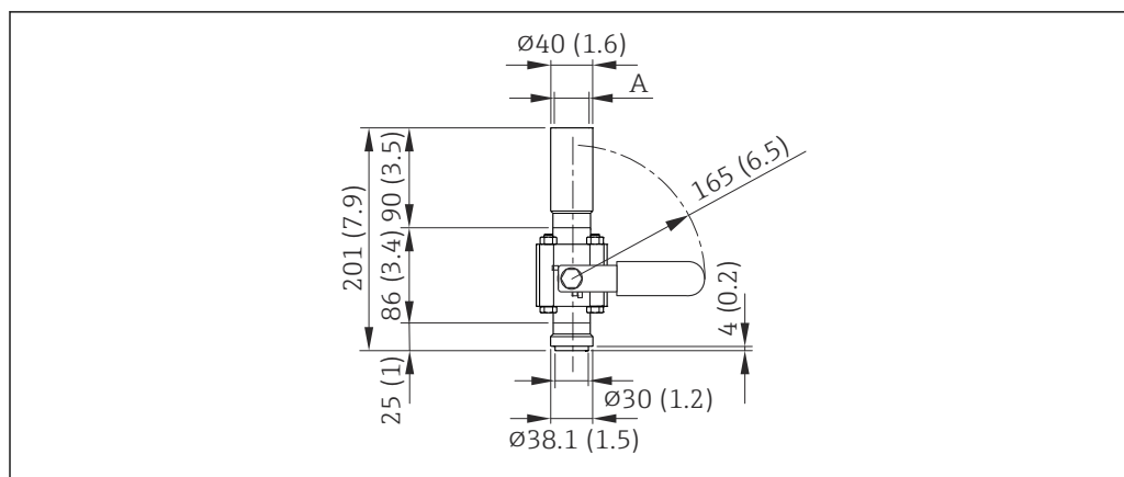
36 Dimensões: mm (pol.)
