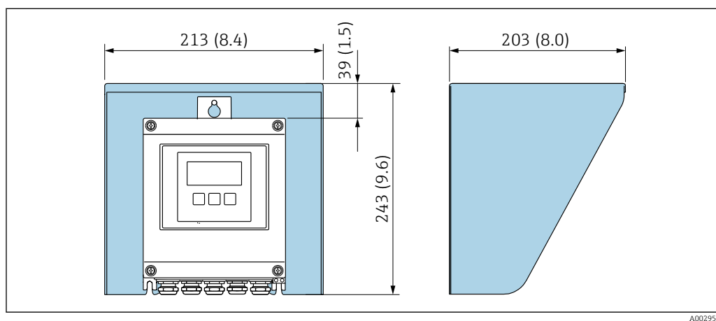
33 Tampa de proteção contra tempo para Proline 500 - digital; unidade de engenharia mm (pol.)
