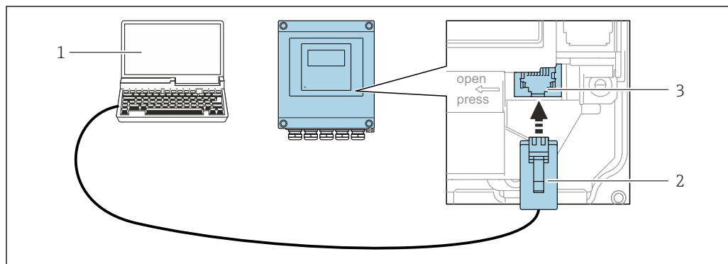
46 Conexão através de Interface de operação (CDI-RJ45)
