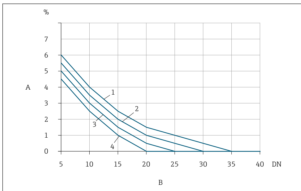
21 O erro medido adicional a ser esperado sem condicionadores de vazão depende do tipo de perturbação e do escoamento de entrada
