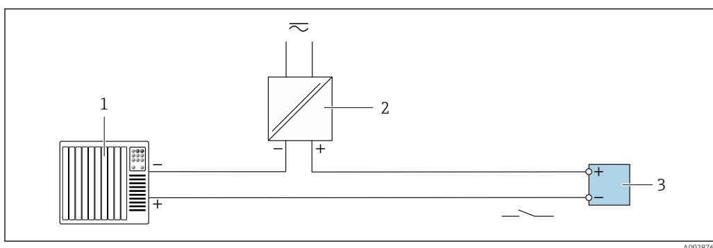
9 Exemplo de conexão para saída comutada (passiva)
