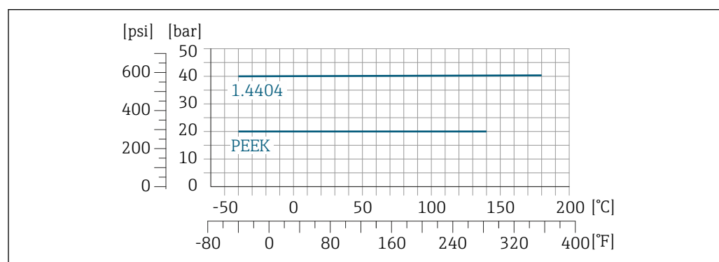
27 Com o material de conexão ajustável 1.4404/F316L/F316
