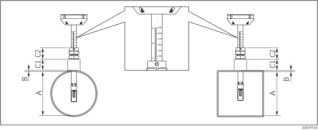
13 Déterminer les dimensions A, B, C1 et C2
