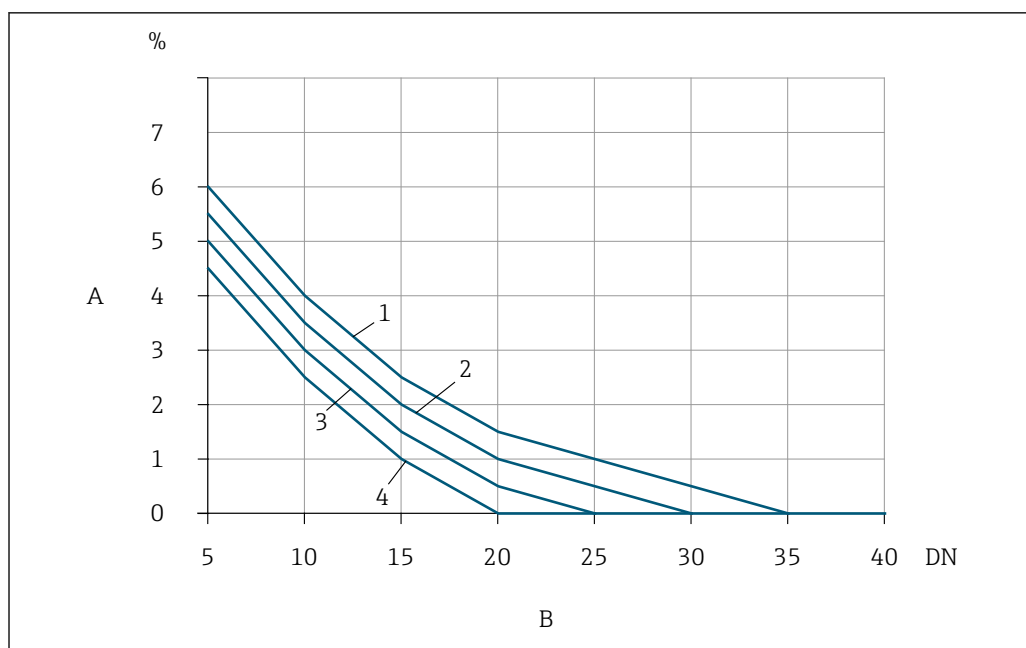
21 L'écart de mesure supplémentaire auquel il faut s'attendre en l'absence de tranquillisateurs de débit dépend du type de perturbation et de la longueur droite d'entrée
