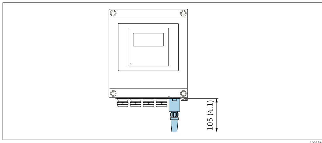
40 Unité de mesure mm (in)
