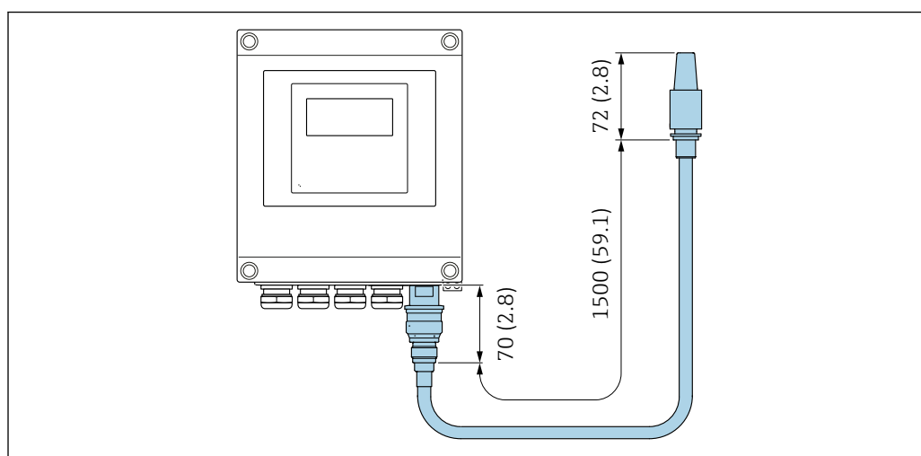
41 Unité de mesure mm (in)
