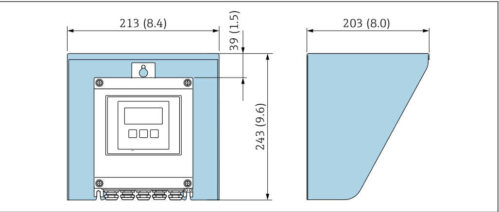
39 Capot de protection climatique pour Proline 500 – numérique ; unité de mesure mm (in)
