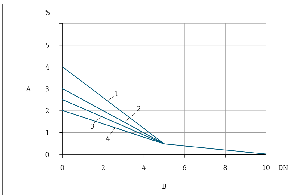
23 Écart de mesure supplémentaire auquel il faut s'attendre avec les tranquillisateurs de débit en fonction du type de perturbation et de la longueur droite d'entrée
