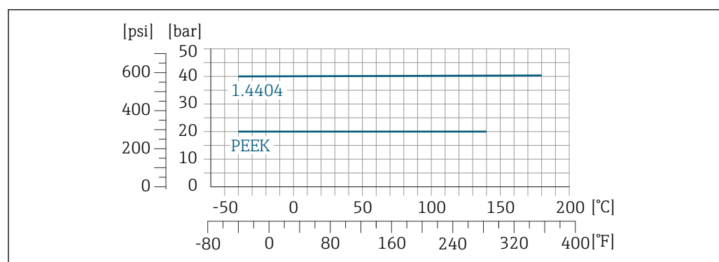
27 Avec matériau de raccord à compression 1.4404/F316L/F316
