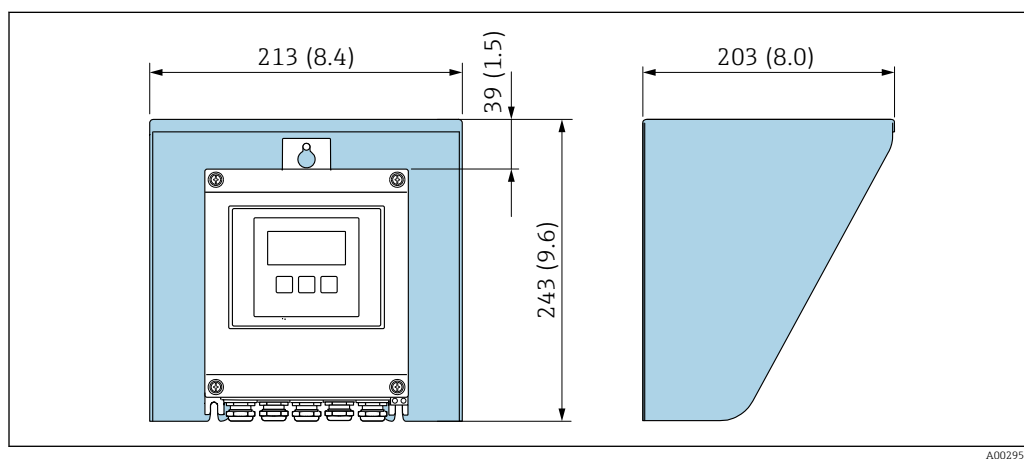
33 Capot de protection climatique pour Proline 500 – numérique ; unité de mesure mm (in)
