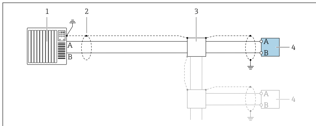
5 Exemple de raccordement pour Modbus RS485, zone non explosible et Zone 2 ; Class I, Division 2
